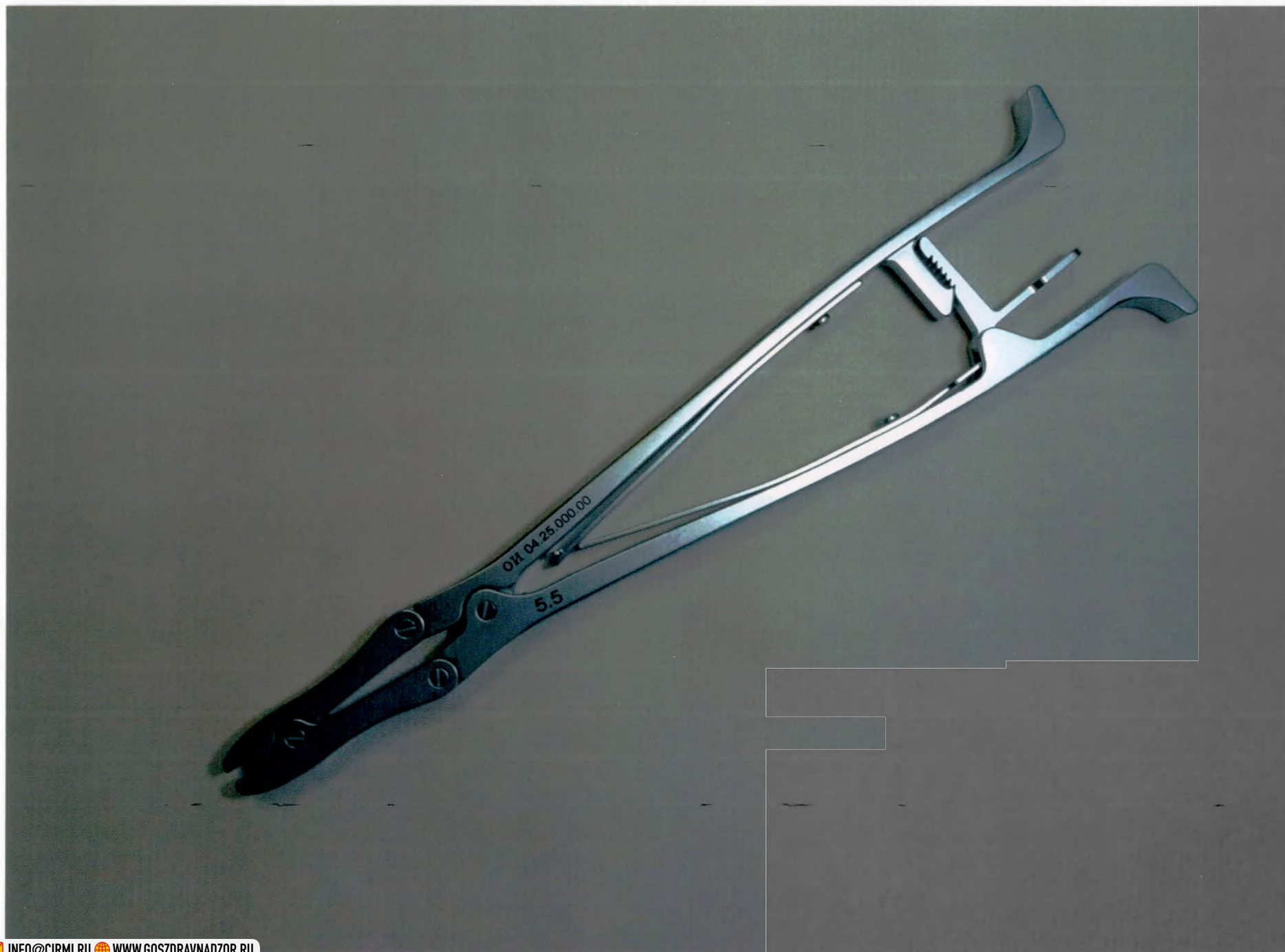
Рисунок 51. ОИ 04.25.000.00 Силовые щипцы. Общий вид.
