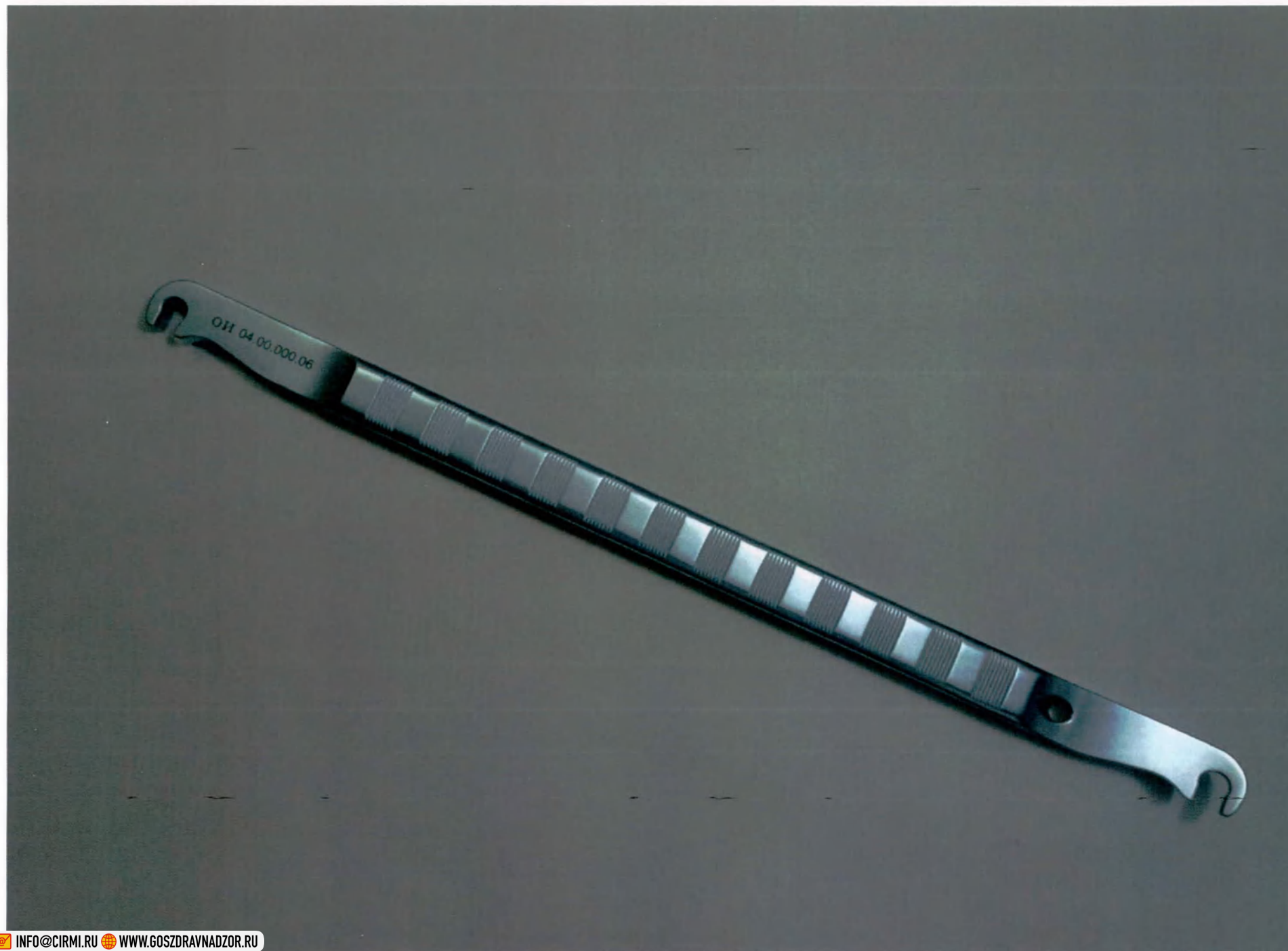
Рисунок 57. ОИ 04.00.000.06 Изгибатель стержня в ране правый. Общий вид.
