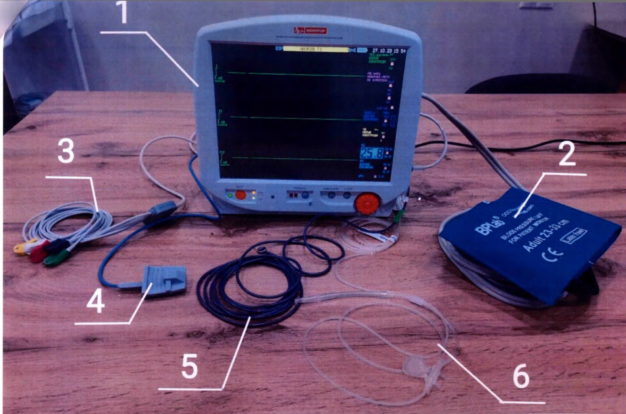
Общий вид Монитора реанимационного и анестезиологического для контроля ряда физиологических параметров МИТАР-01-«Р-Д»/12, МТЦ.83.00.100, где: 1 – блок монитора; 2 – манжета НИАД; 3 – кабель ЭКГ; 4 – датчик SpO 2 ; 5 – датчик температуры; 6 – одноразовая линия
