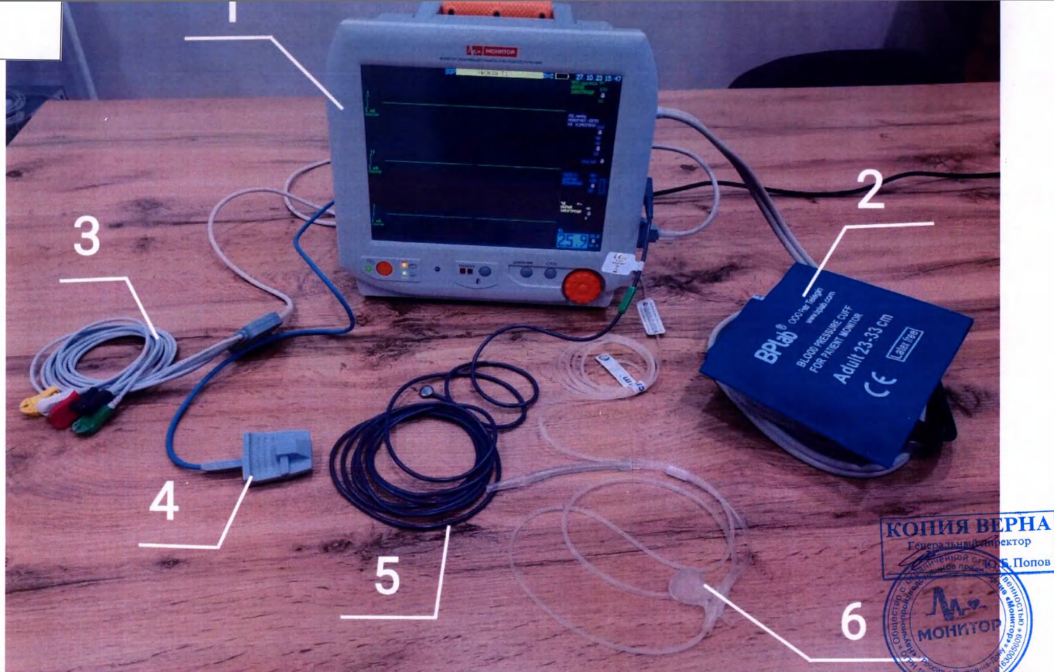
Общий вид Монитора реанимационного и анестезиологического для контроля ряда физиологических параметров МИТАР-01-«Р-Д» Т0, МТЦ.82.00.100, где: 1 – блок монитора; 2 – манжета НИАД; 3 – кабель ЭКГ; 4 – датчик SpO 2 ; 5 – датчик температуры; 6 – одноразовая линия
