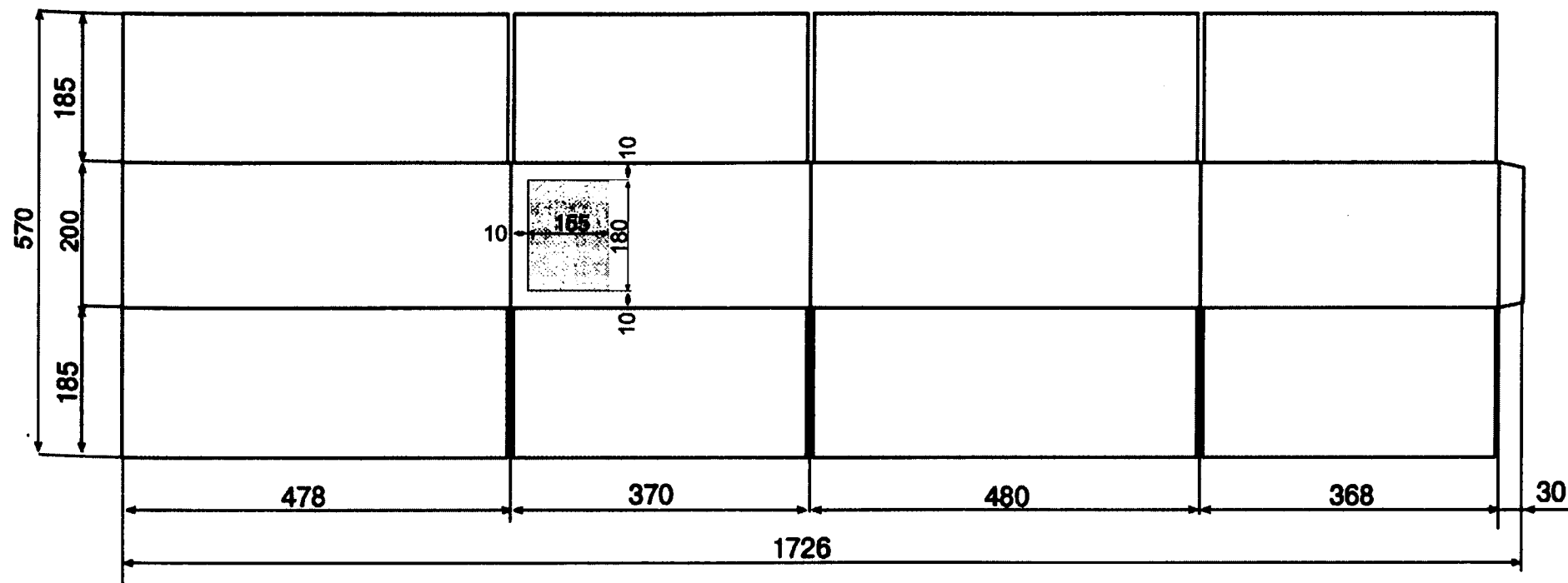
Рисунок 3 – Макет транспортной упаковки. Развертка короба из гофрированного картона с указанием размеров и места наклеивания этикетки.
