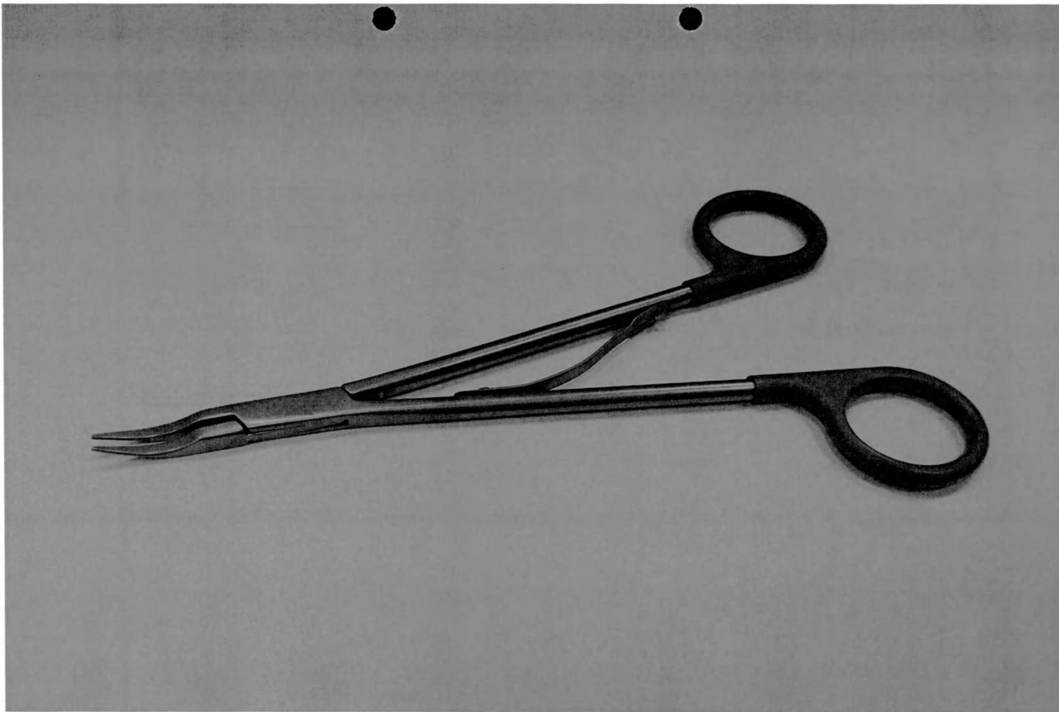
Фото 22. Клип-аппликатор хирургический «МЕРС», многоразового использования, вариант исполнения 4.1, с кольцевой рукояткой REF 2.1, совместимая клипса REF C2.01, REF C8.01, REF C8.02, REF C8.03, REF C8.04, REF C8.05, REF C8.06, REF C8.07, по ТУ 32.50.13-006-56695793-2024
