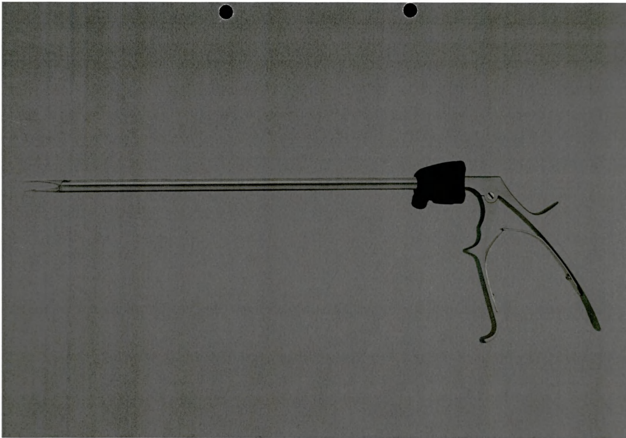
Фото 74. Клип-аппликатор хирургический «МЕРС», многоразового использования, вариант исполнения 6.1, с рычажной рукояткой REF 3.1, совместимая клипса REF C5.01, по ТУ 32.50.13-006-56695793-2024
