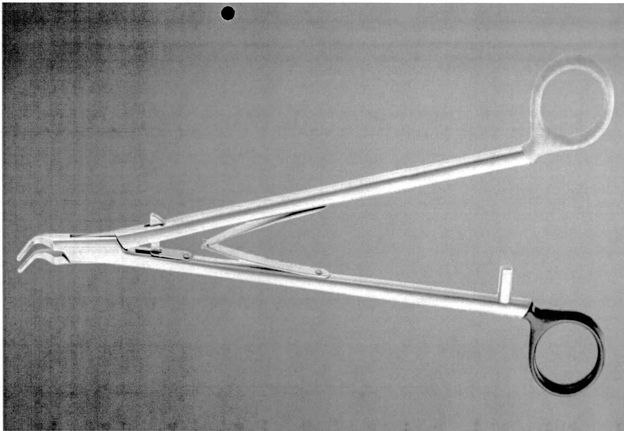
Фото 108. Клип-аппликатор хирургический «МЕРС», многоразового использования, вариант исполнения 7.3, с кольцевой рукояткой REF 2.1, совместимая клипса REF C6.03, REF C7.03, по ТУ 32.50.13-006-56695793-2024
