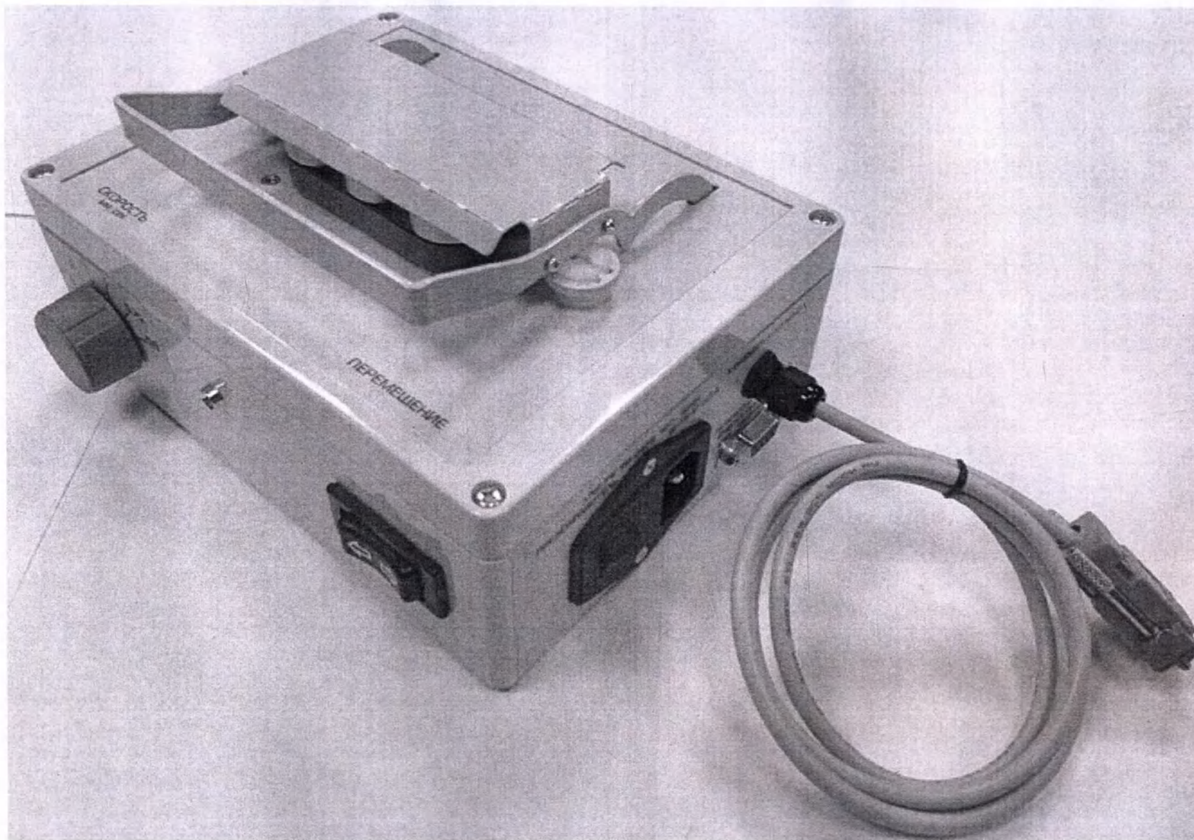
Вид общий. Позиционер электромеханический ин-струментальный ПИ-1
