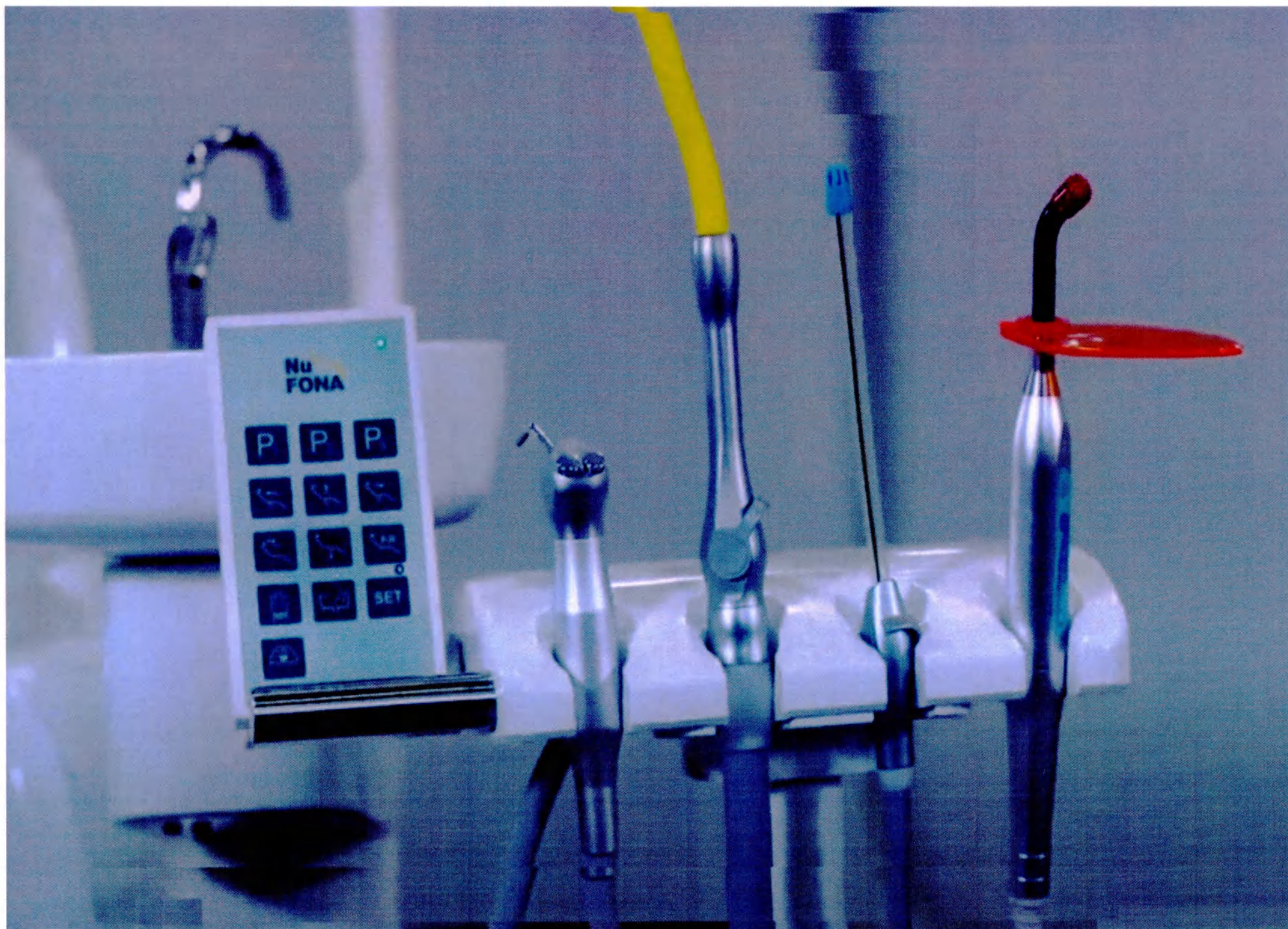
Фото 8. Модуль ассистента на кронштейне укомплектованный пистолетом воздух-вода, шлангом большого хирургического отсоса, шлангом слюноотсоса лампой светополимеризационной
