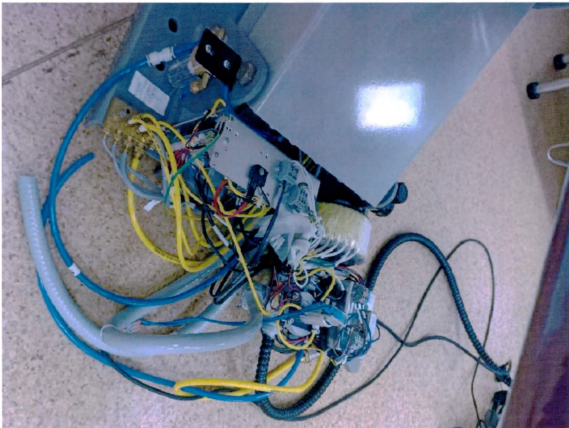
Фото 28. Встроенный электрический энергоблок со снятым корпусом.
