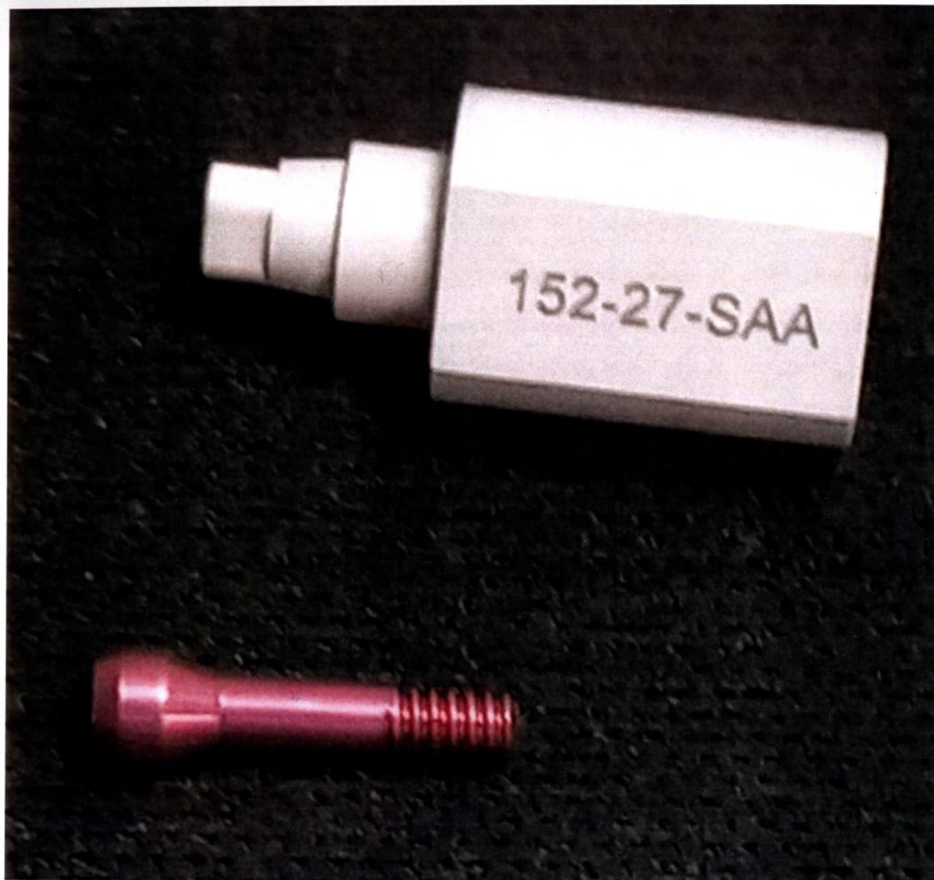
Скан-маркер BL, с уровня имплантата, лабораторный, с винтом
