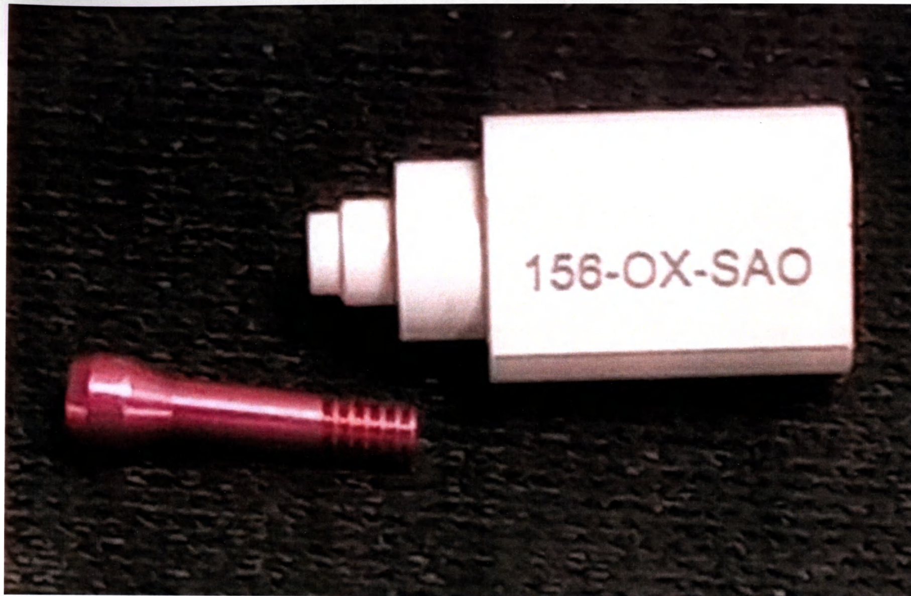
Скан-маркер inLink TL, с уровня имплантата, лабораторный, с винтом
