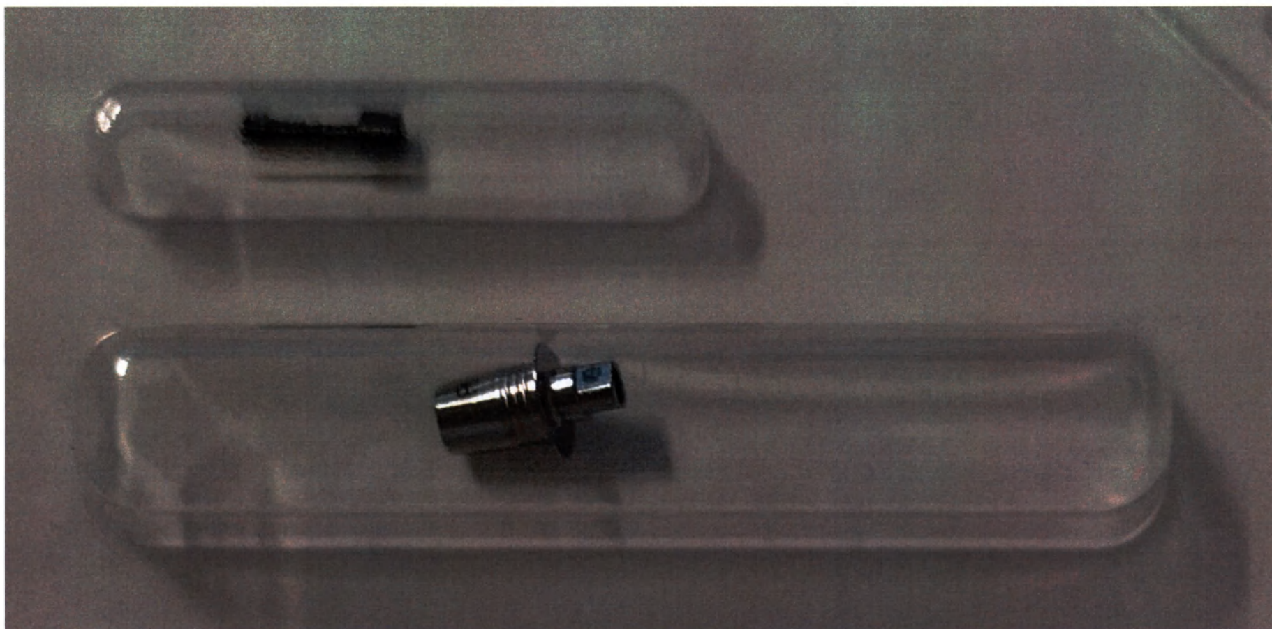
Титановое основание TL, для CEREC, платформа R 4.8 мм, с винтом
