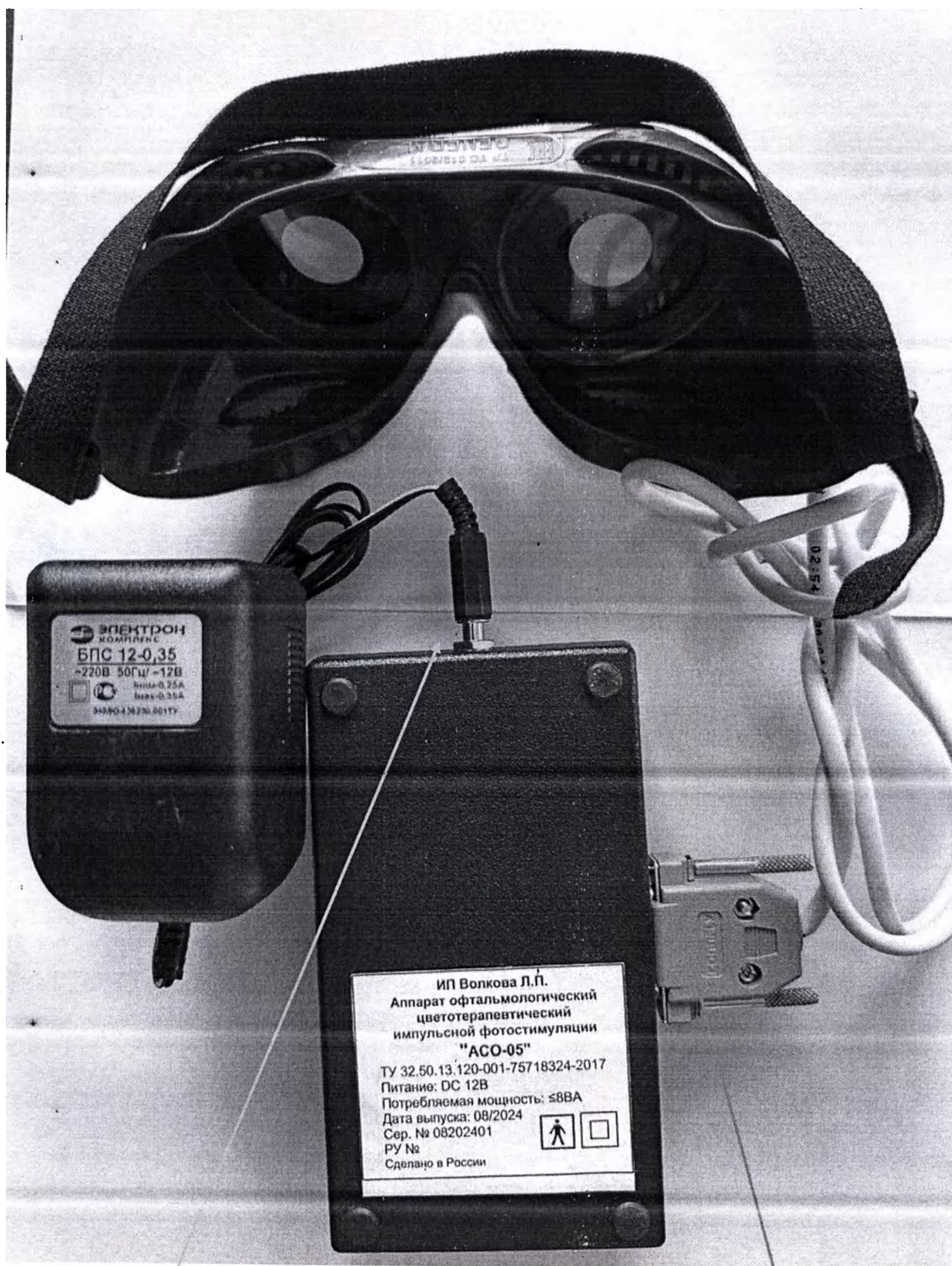
Разъём блока питания
