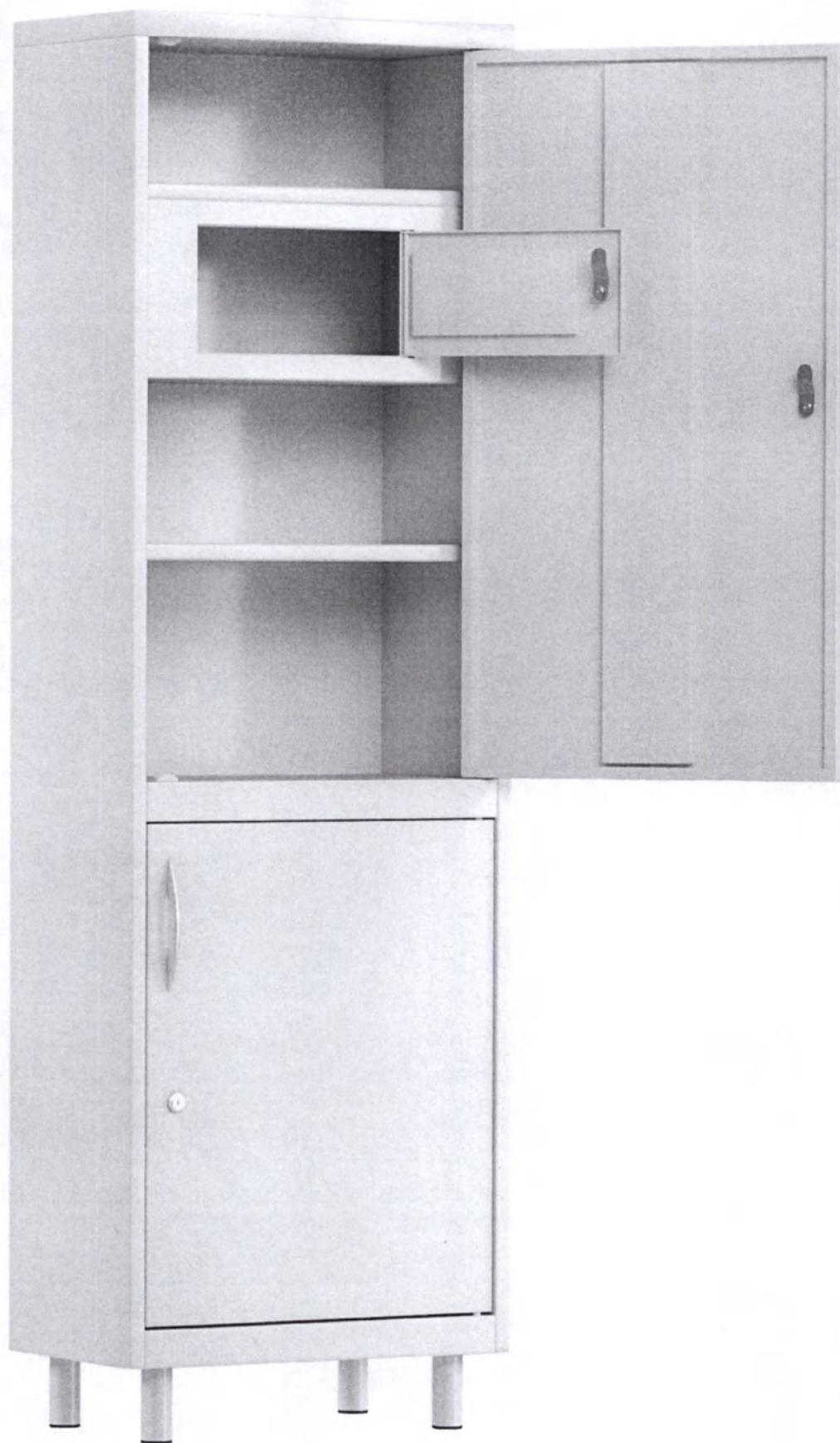
Фотография 34. Шкаф медицинский металлический для лекарственных средств по ТУ 32.50.30-005-68690950-2024, вариант исполнения ШММн.01.01 (мод.2). Общий вид (открыт).
