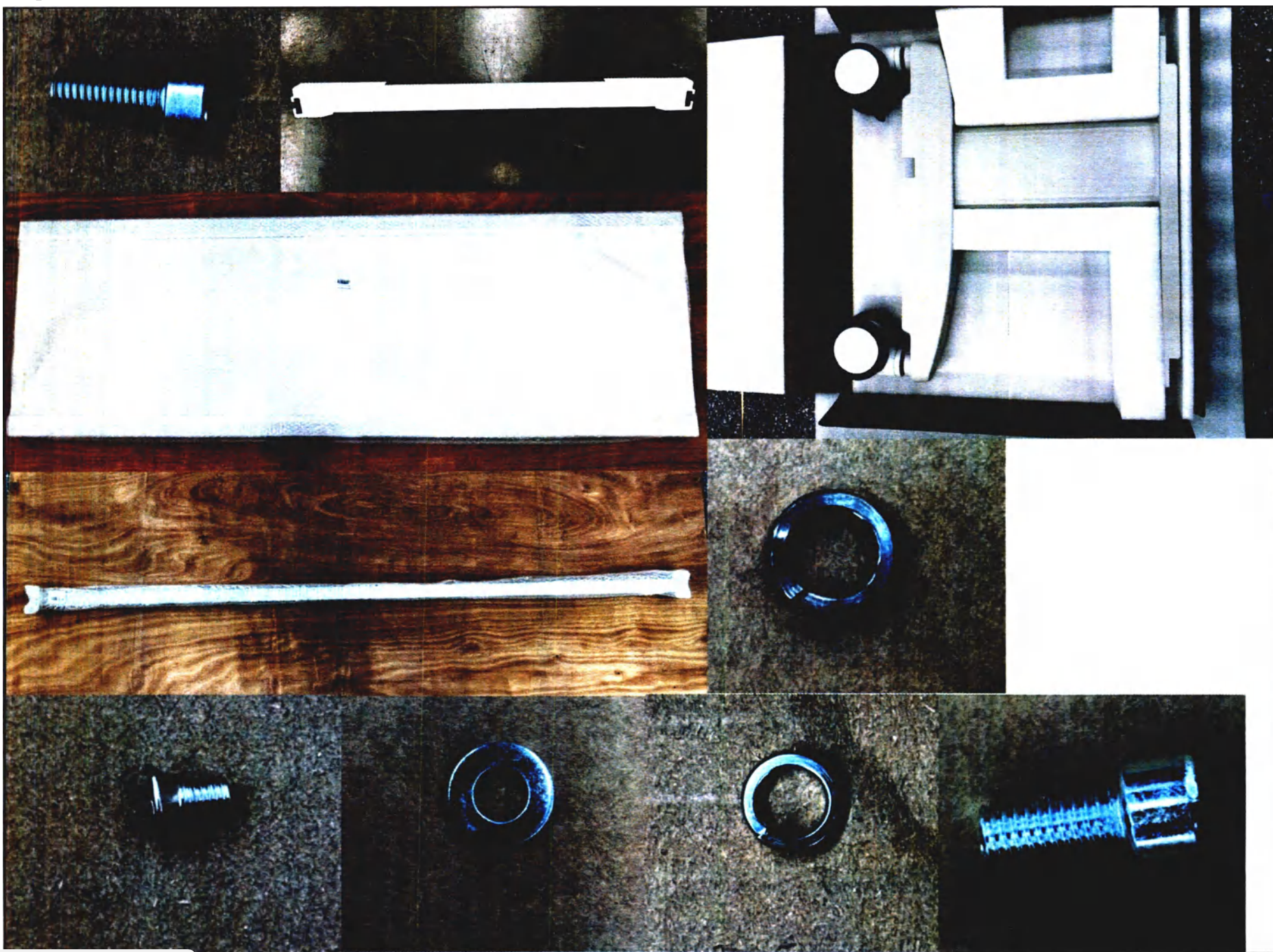
Передвижной стол для пациента (в разборе)
