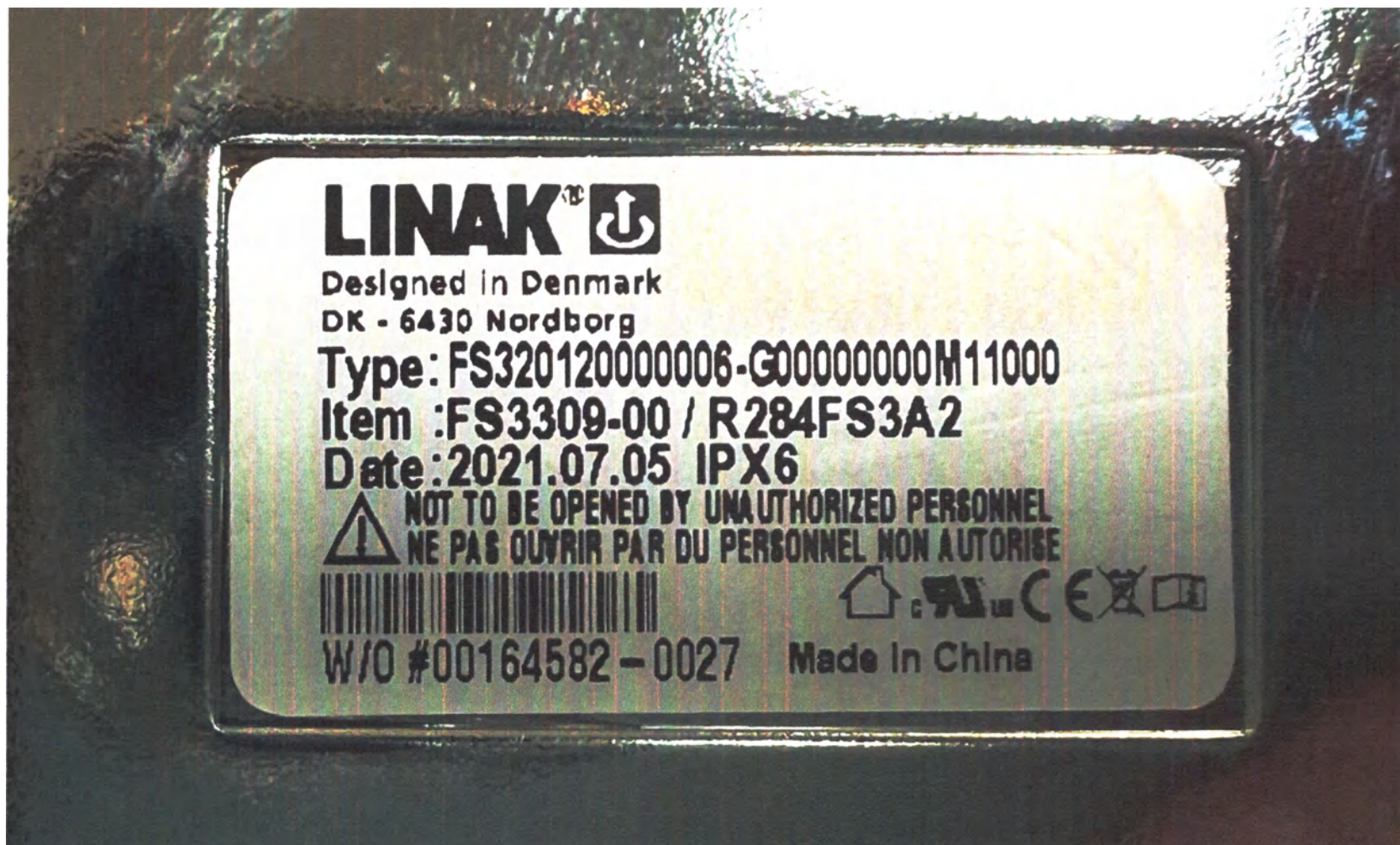
Маркировка: Пульт ногоного управления (Capre EX2)
