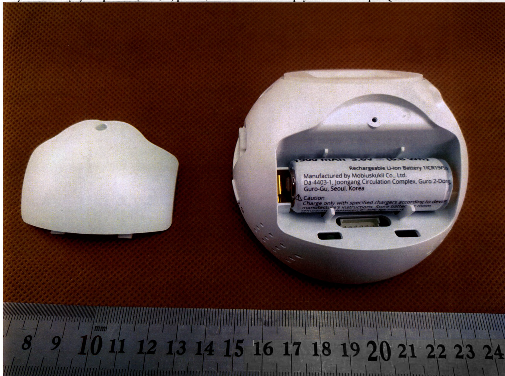
Рисунок 14. Аккумулятор Li-Ion (DC 3,6В) размещенный в основном корпусе апекслокатора EQ-PEX
