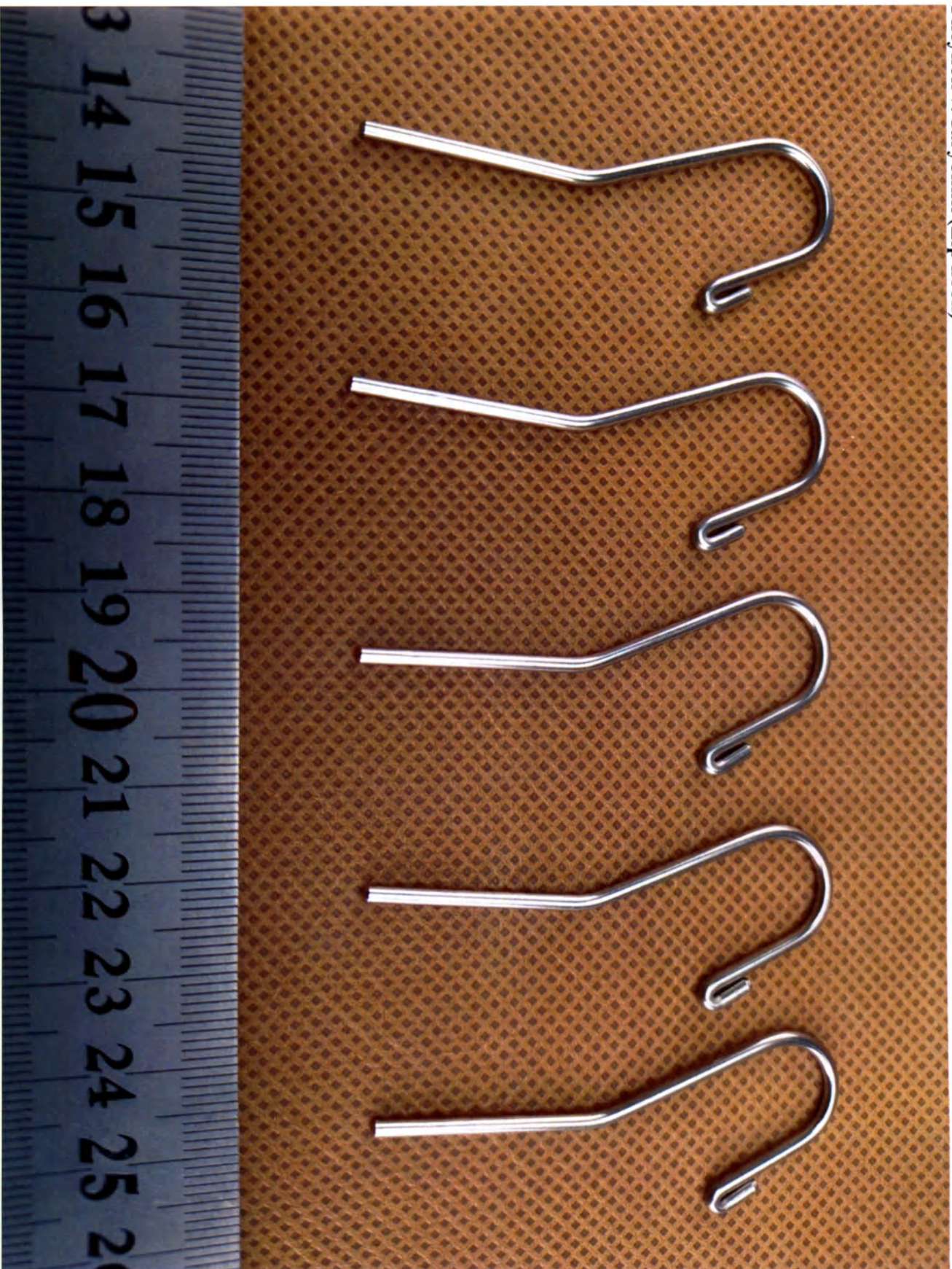
Рисунок 7. Затягивник (Lip hook)
