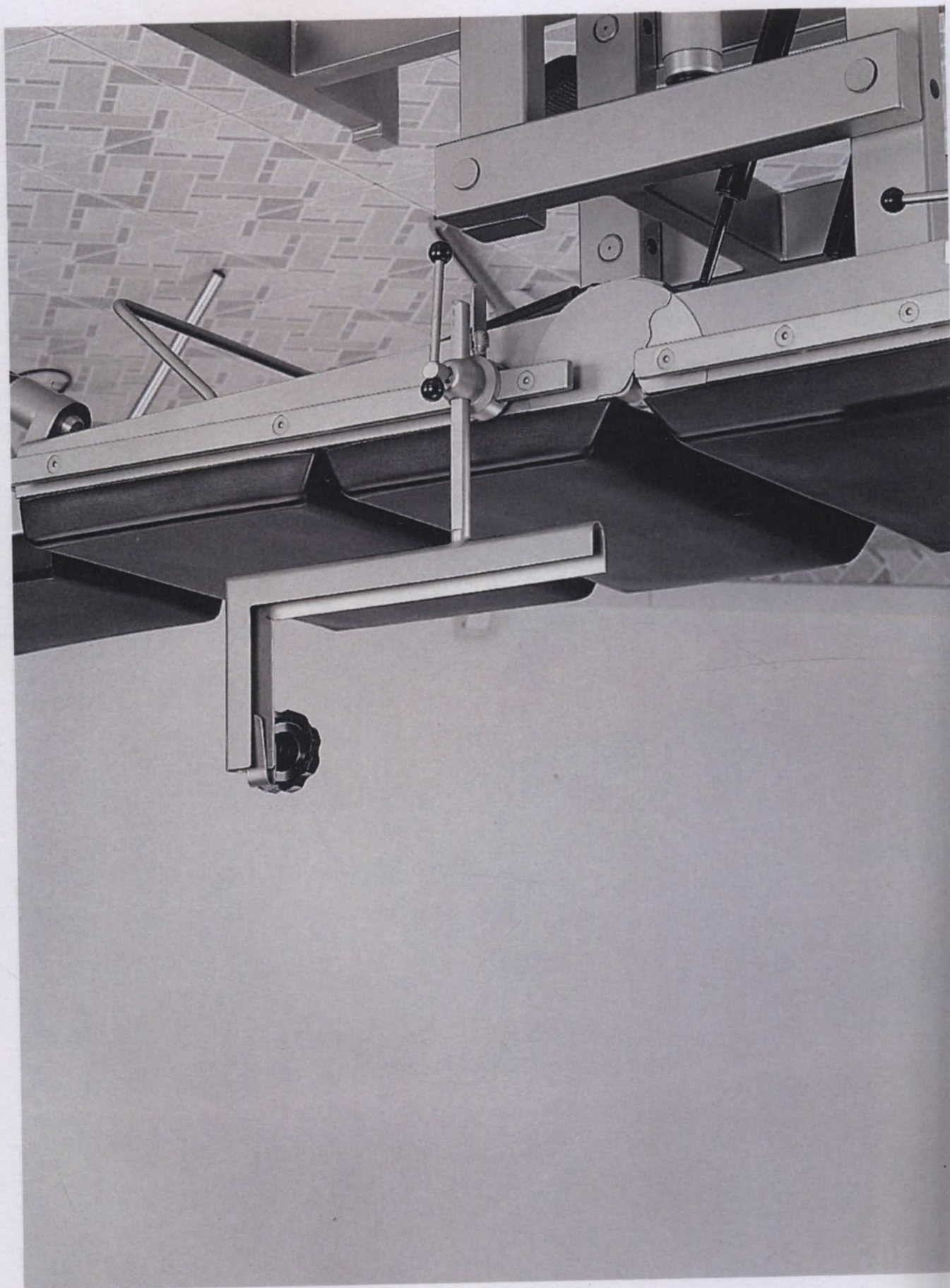
Держатель R-кассеты I-II, вертикальный, с креплением WS-33.0
