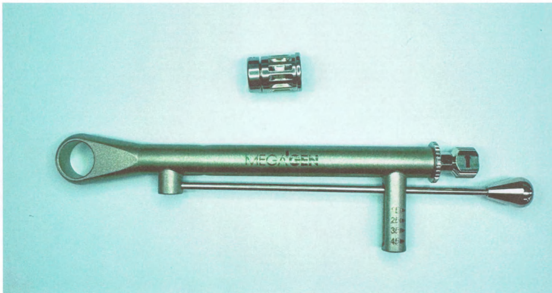
Ключ динамометрический (Torque Wrench), Адаптер для динамометрического ключа (Torque Wrench Adapter)
