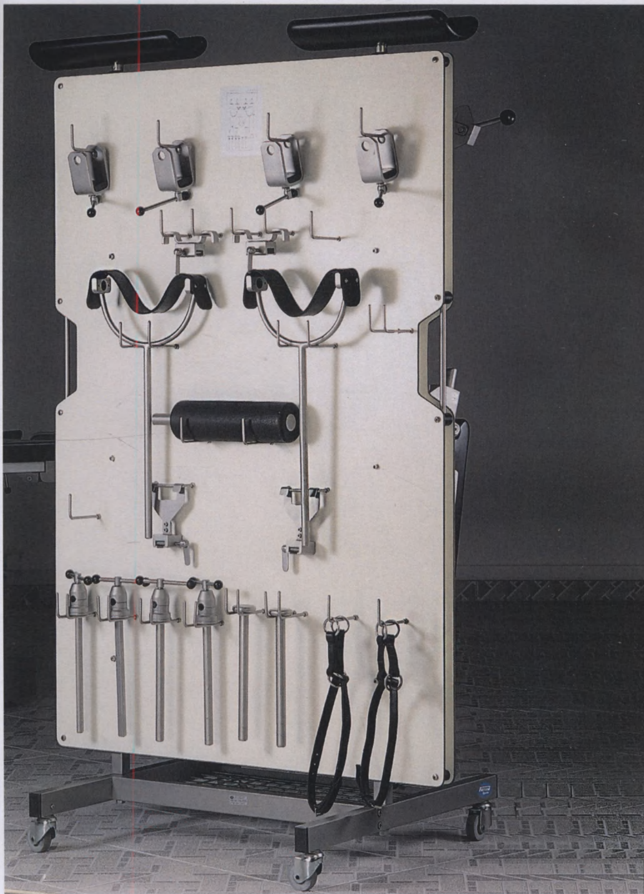
Стойка для ортопедической приставки, на роликах WS-13.6
