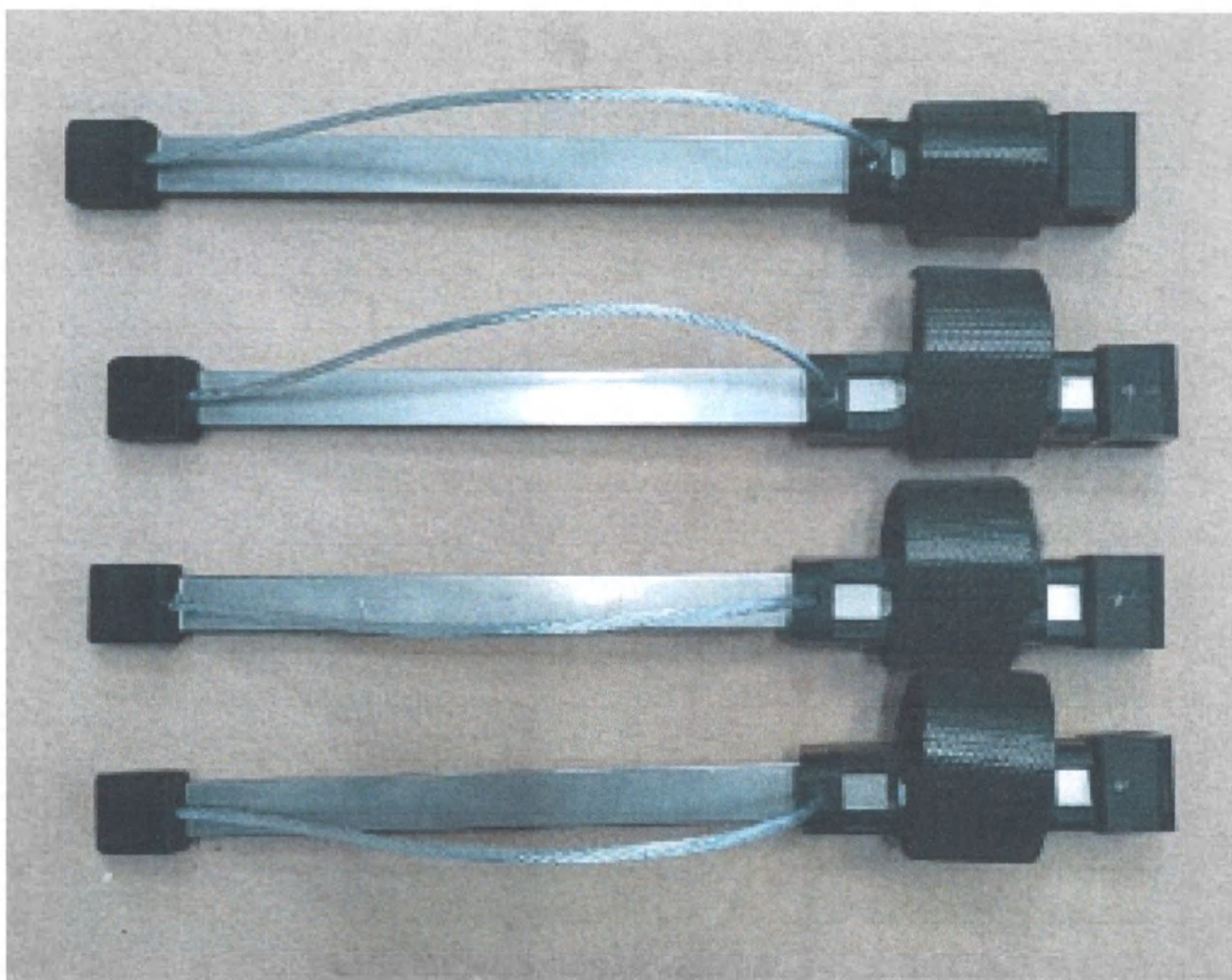
Поводок пальца в сборе с лентами липучками для фиксации пальцев
