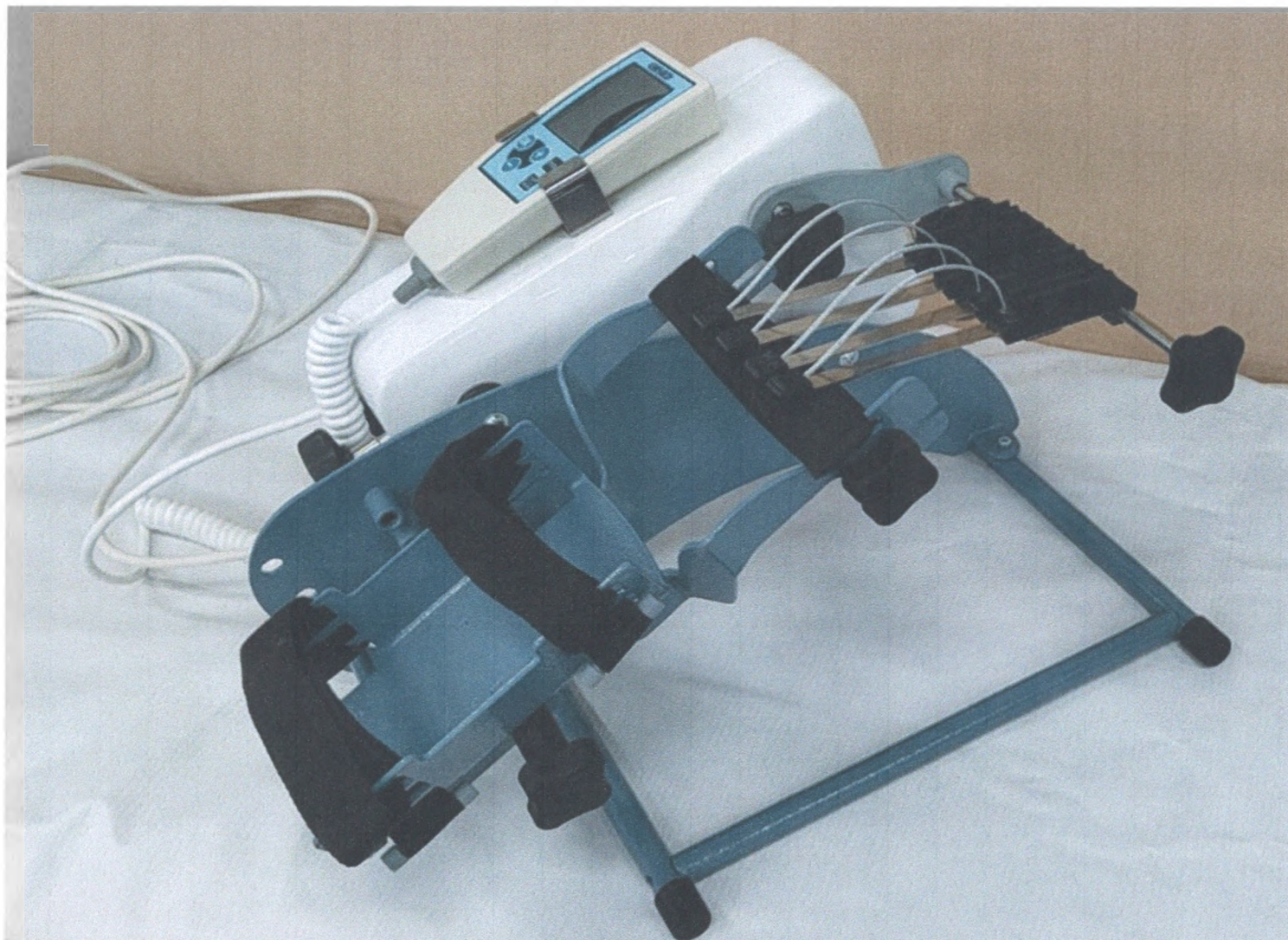
Аппарат для роботизированной механотерапии верхних конечностей в варианте исполнения «FLEX-F05F»
