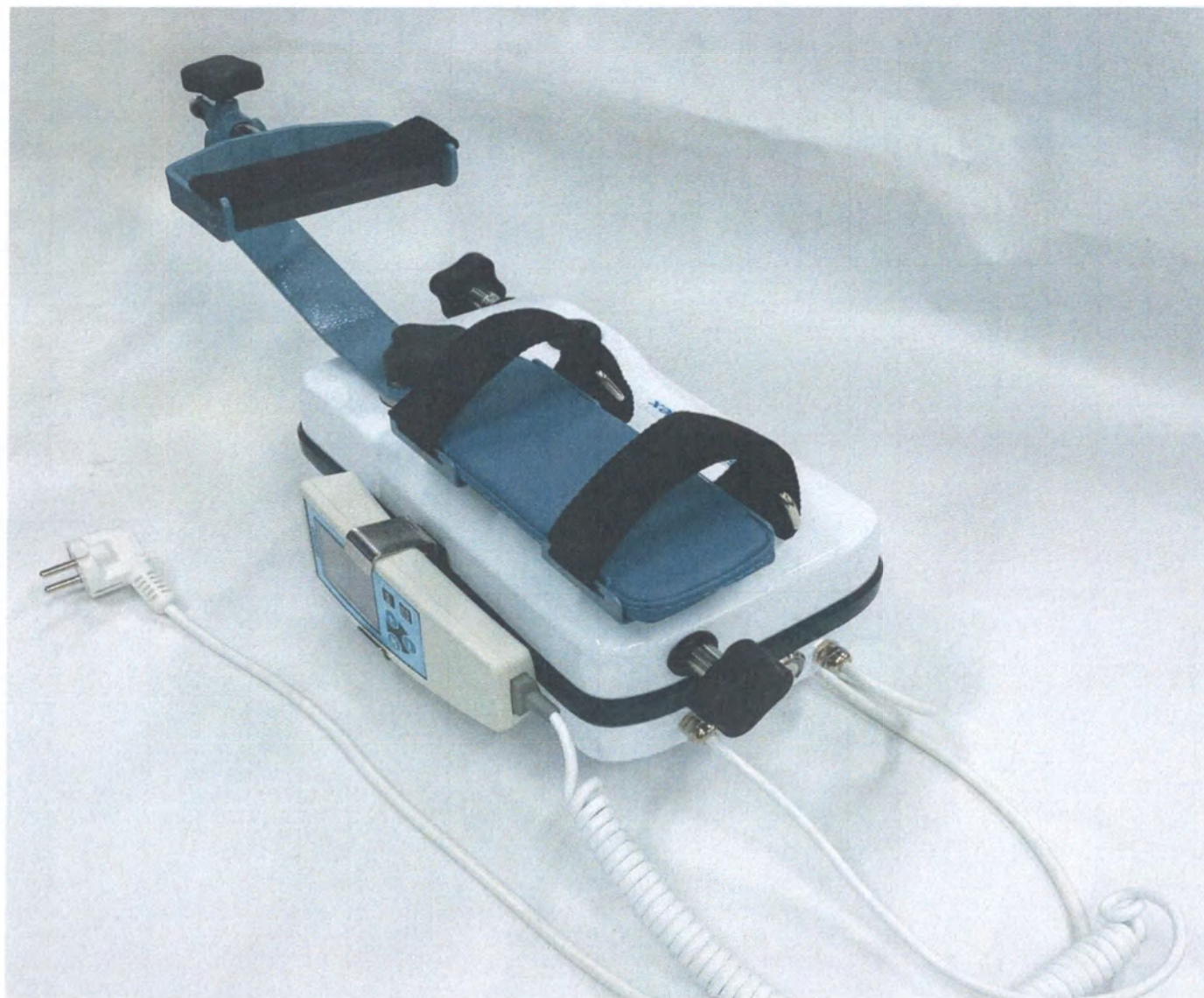
Аппарат для роботизированной механотерапии верхних конечностей в варианте исполнения «FLEX-F05FR» в положении разработки лучезапястного сустава
