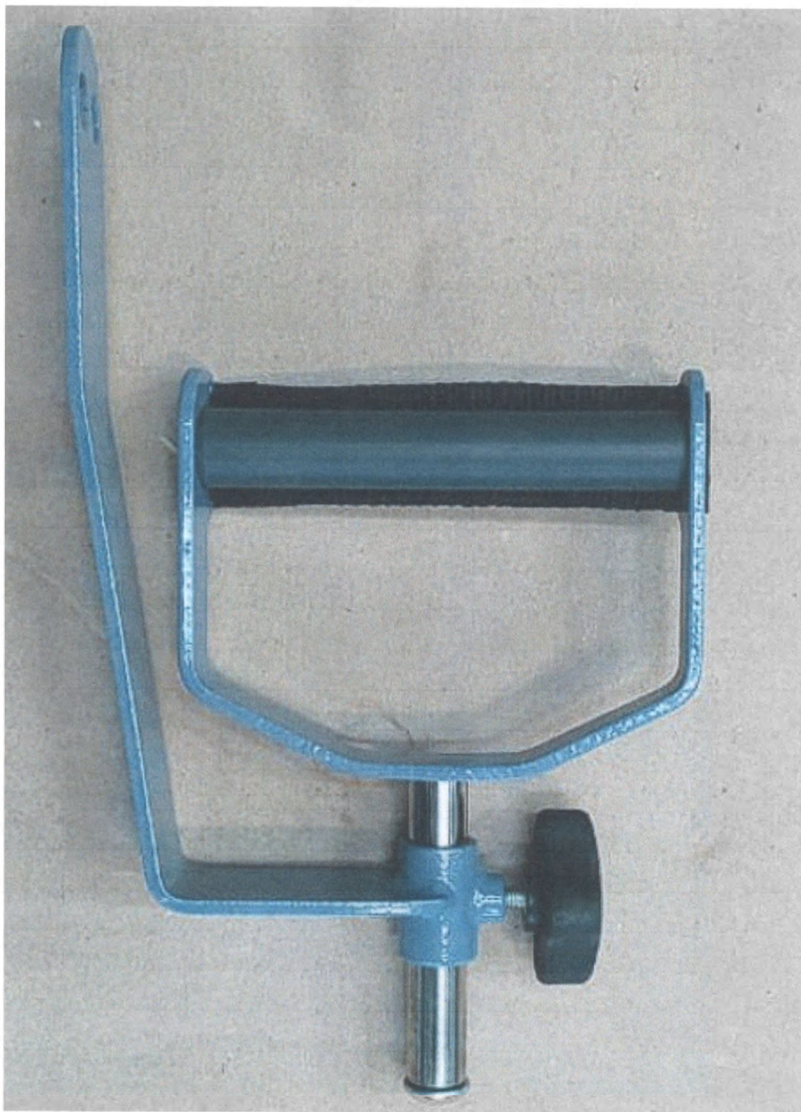
Ручка для сгибания/разгибания и девиации в сборе с водилом
