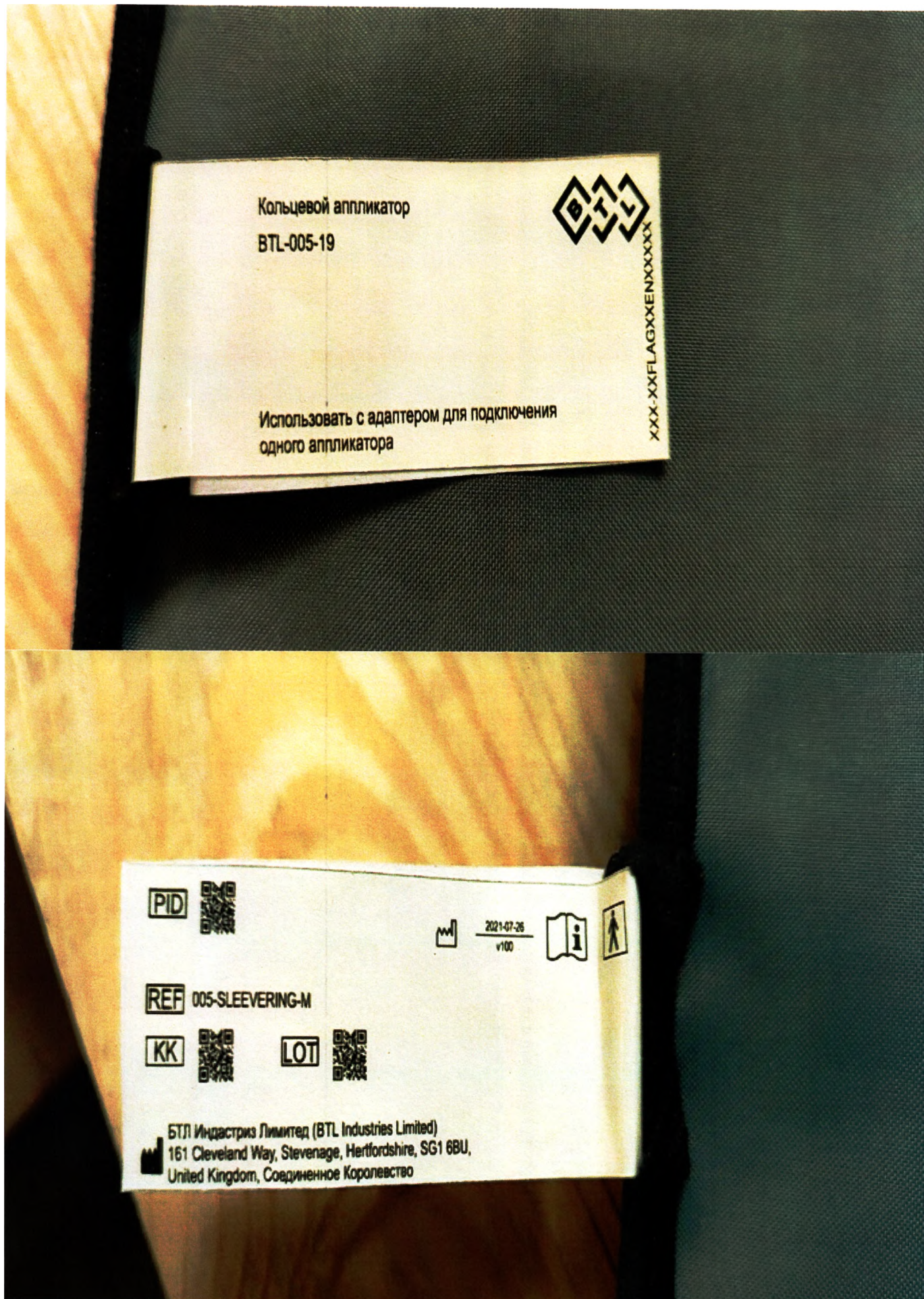
9.1 Маркировка на Кольцевом аппликаторе, артикул BTL-005-19
