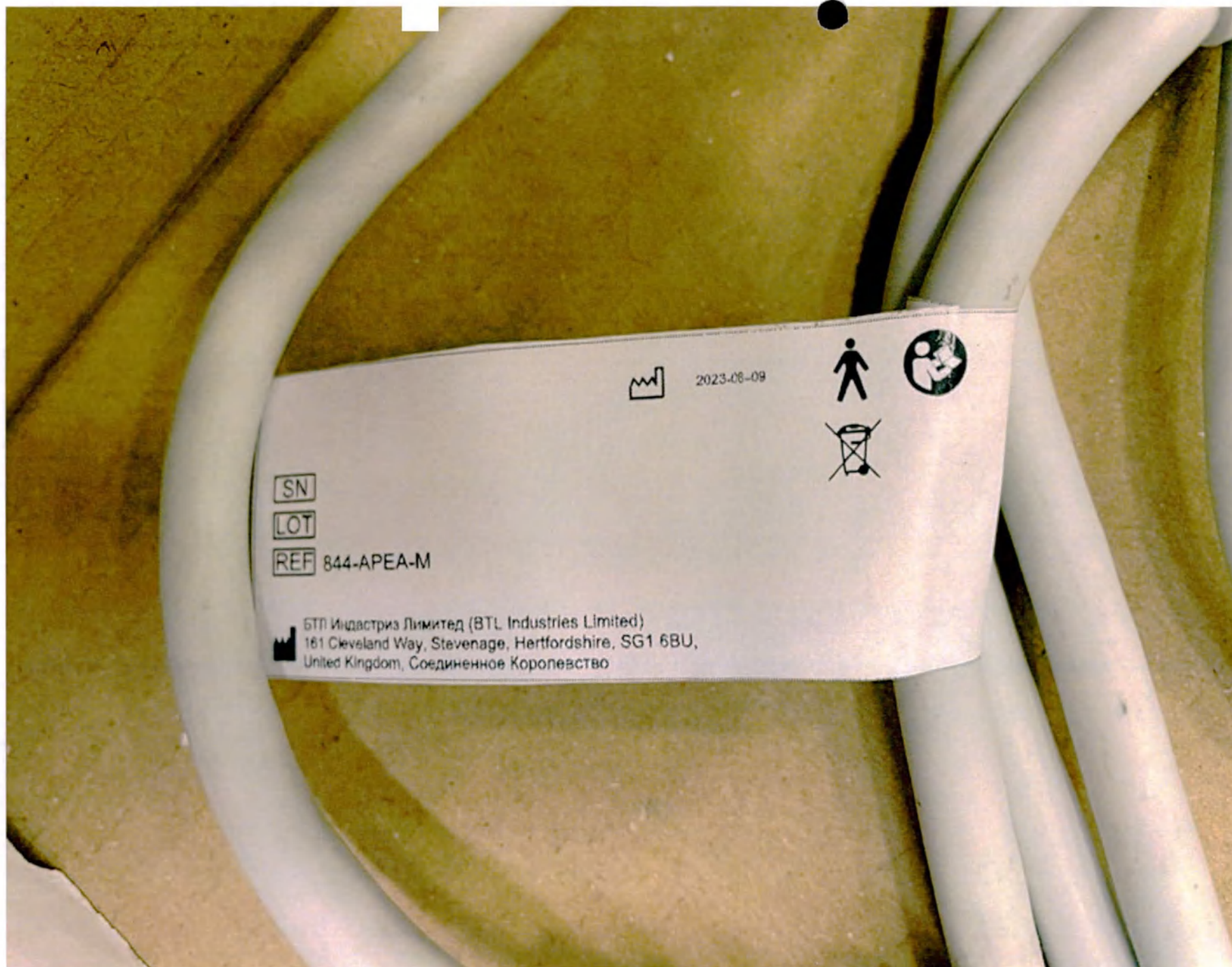
62 7.1 Маркировка аппликатора Easy 844-APEA-M
