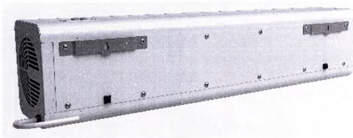
Рис.13. Модель II (вид сзади) с креплением для размещения горизонтально
