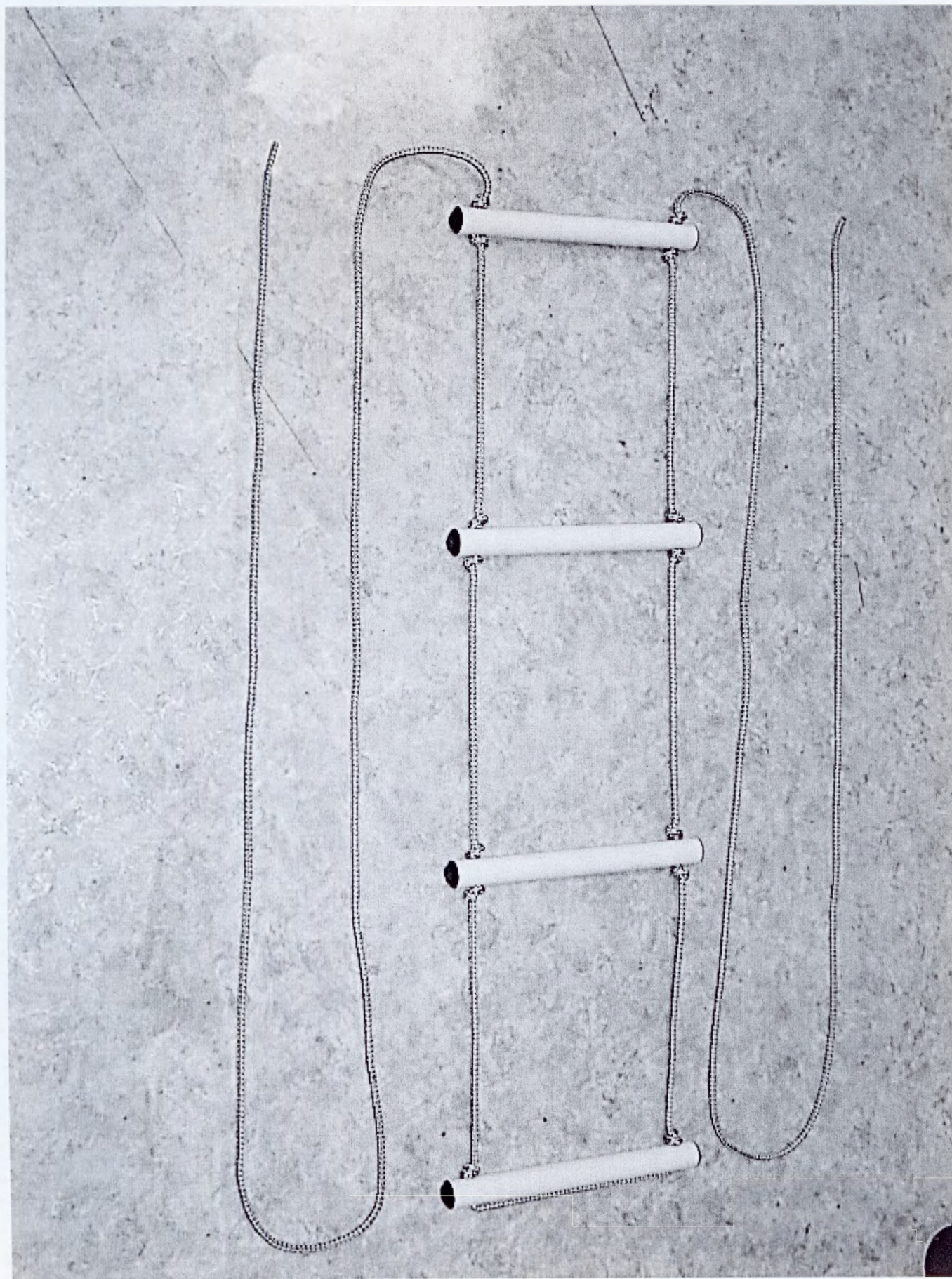
Устройство для подтягивания в виде лестницы
