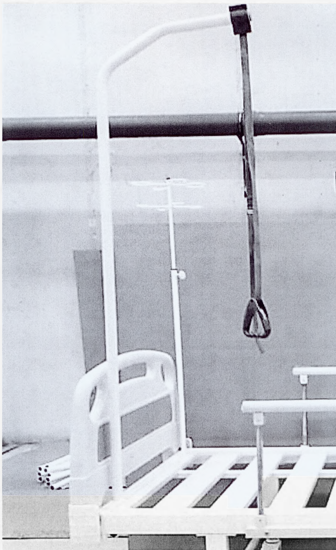
Устройство для подтягивания в виде стойки
