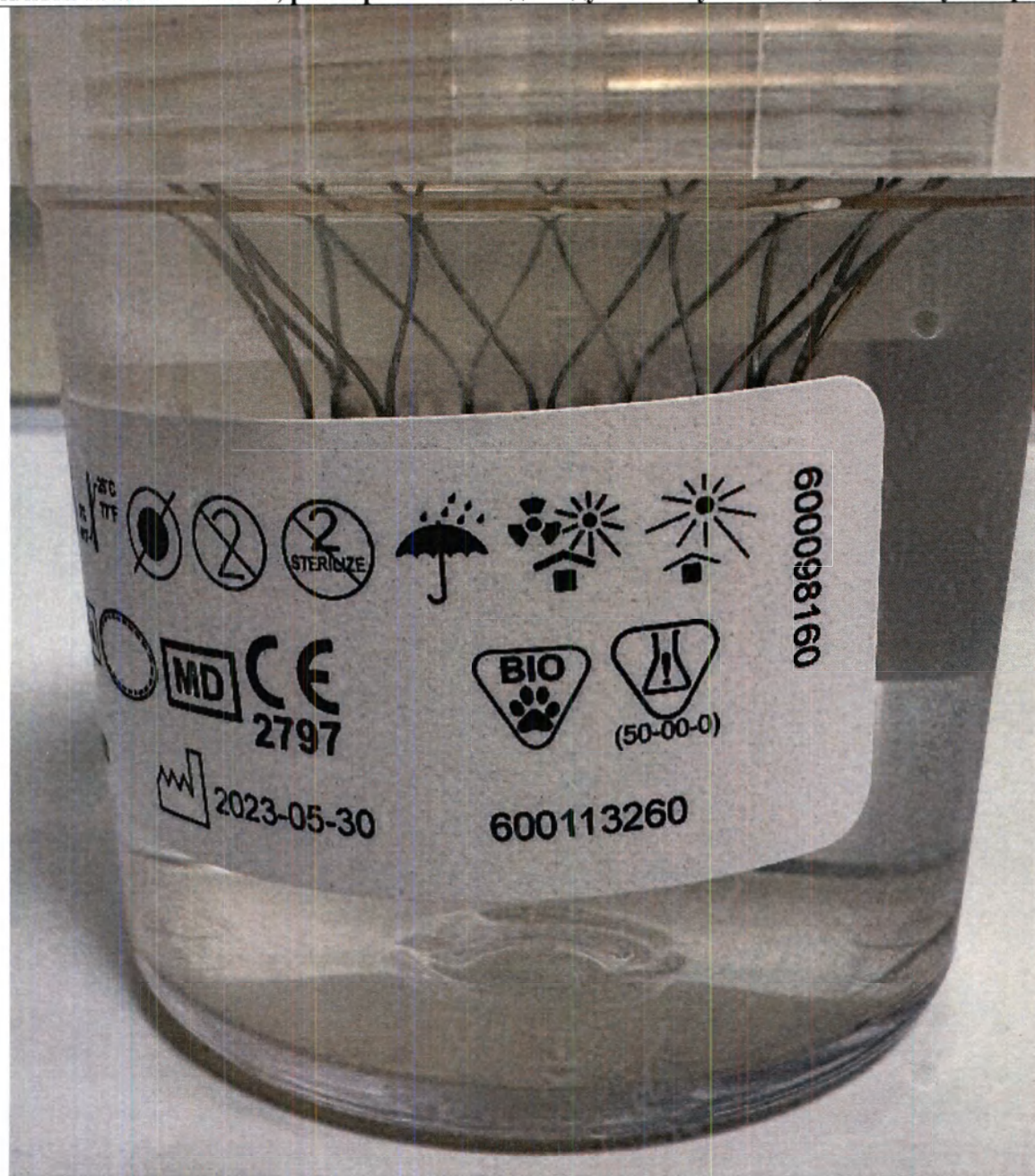
Система имплантации транскатетерного аортального клапана Navitor. Аортальный клапан Navitor, размер 23 мм. Индивидуальная упаковка, вид сбоку. Маркировка.
