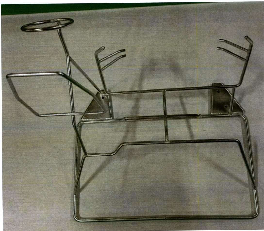
Машина мойки судов Каскад СМ-100, КСМ100.00.000_01 Принадлежности. Загрузочная корзина
