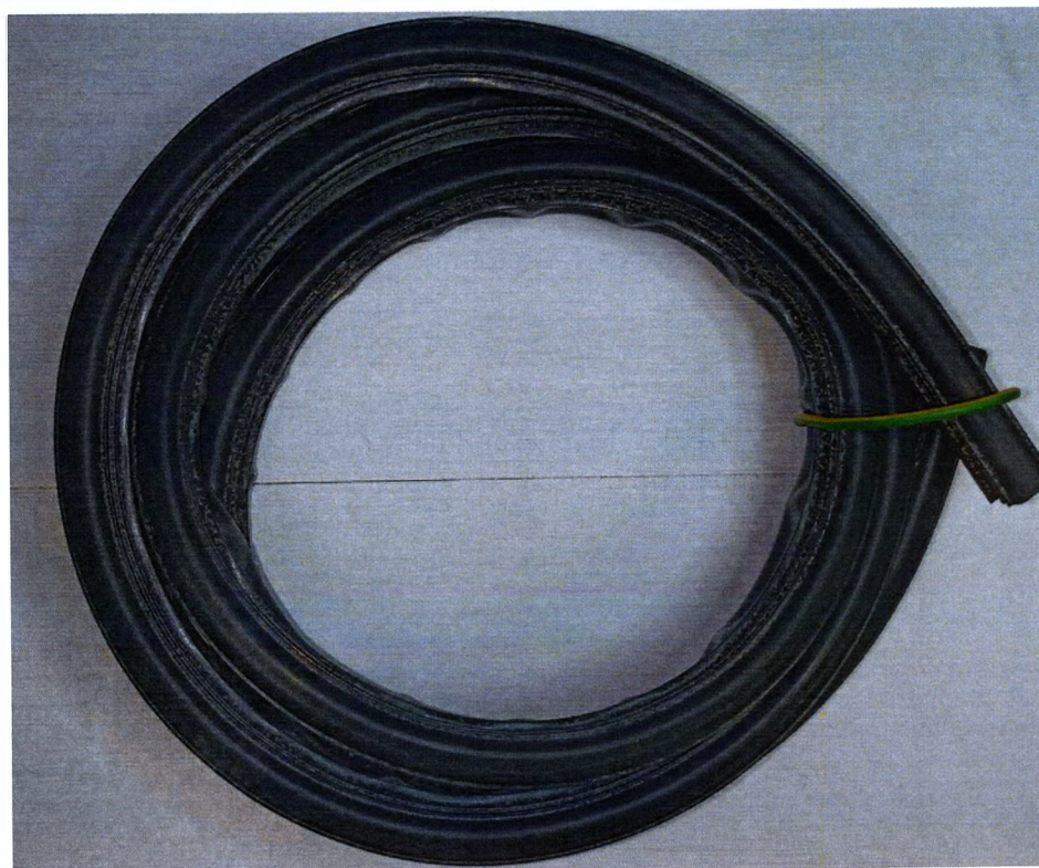
Машина мойки суден Каскад СМ-100, КСМ100.00.000 Запасные части. Прокладка двери камеры
