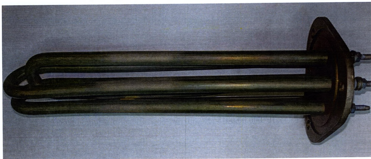
Машина мойки суден Каскад СМ-100, КСМ100.00.000_01 Запасные части. Блок ТЭН
