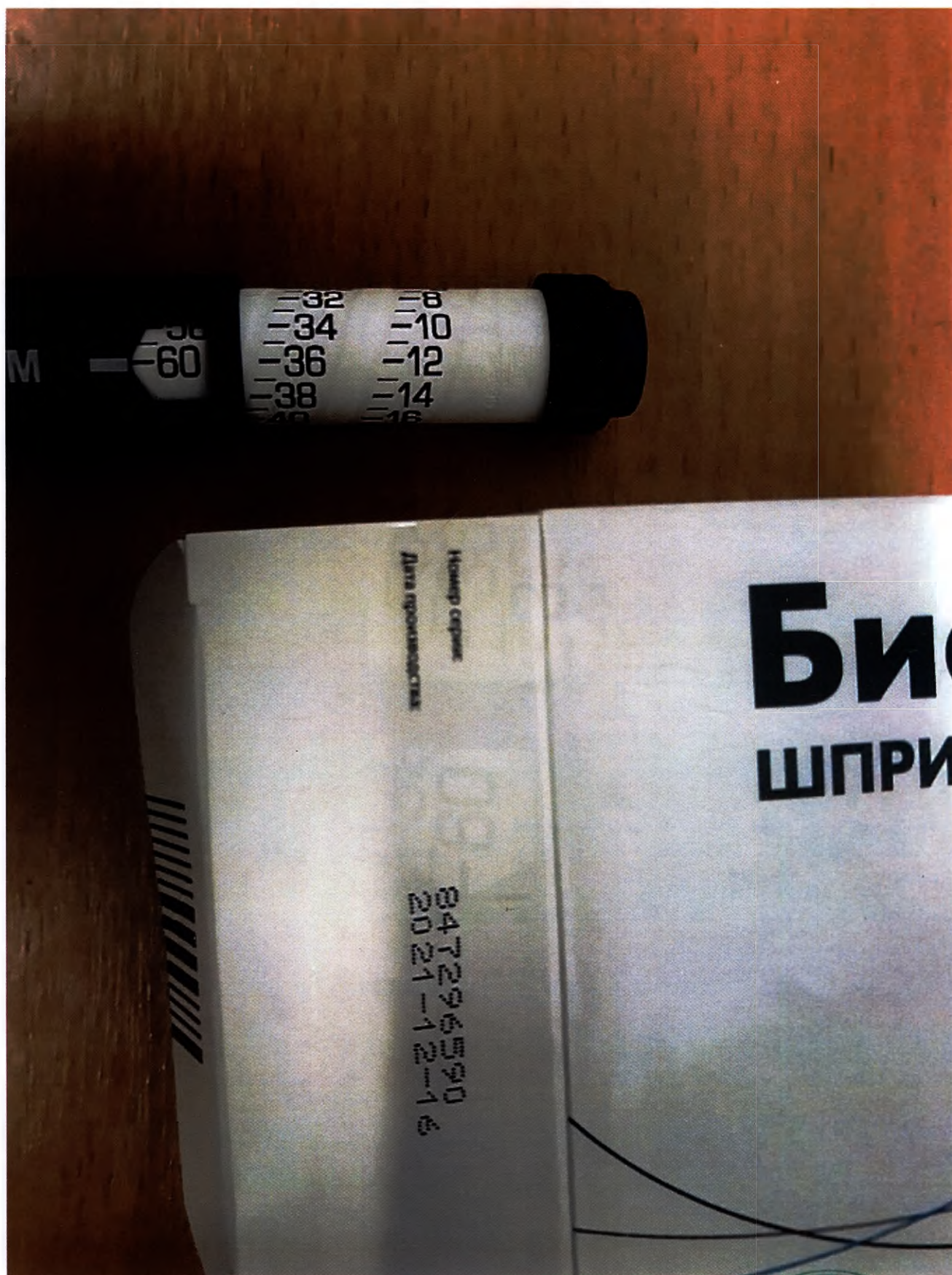
Фото 2. Шприц-ручка БиоматикПен®М для картриджей емкостью 3 мл (фрагмент пачки и шприц-ручки с номером серии).
