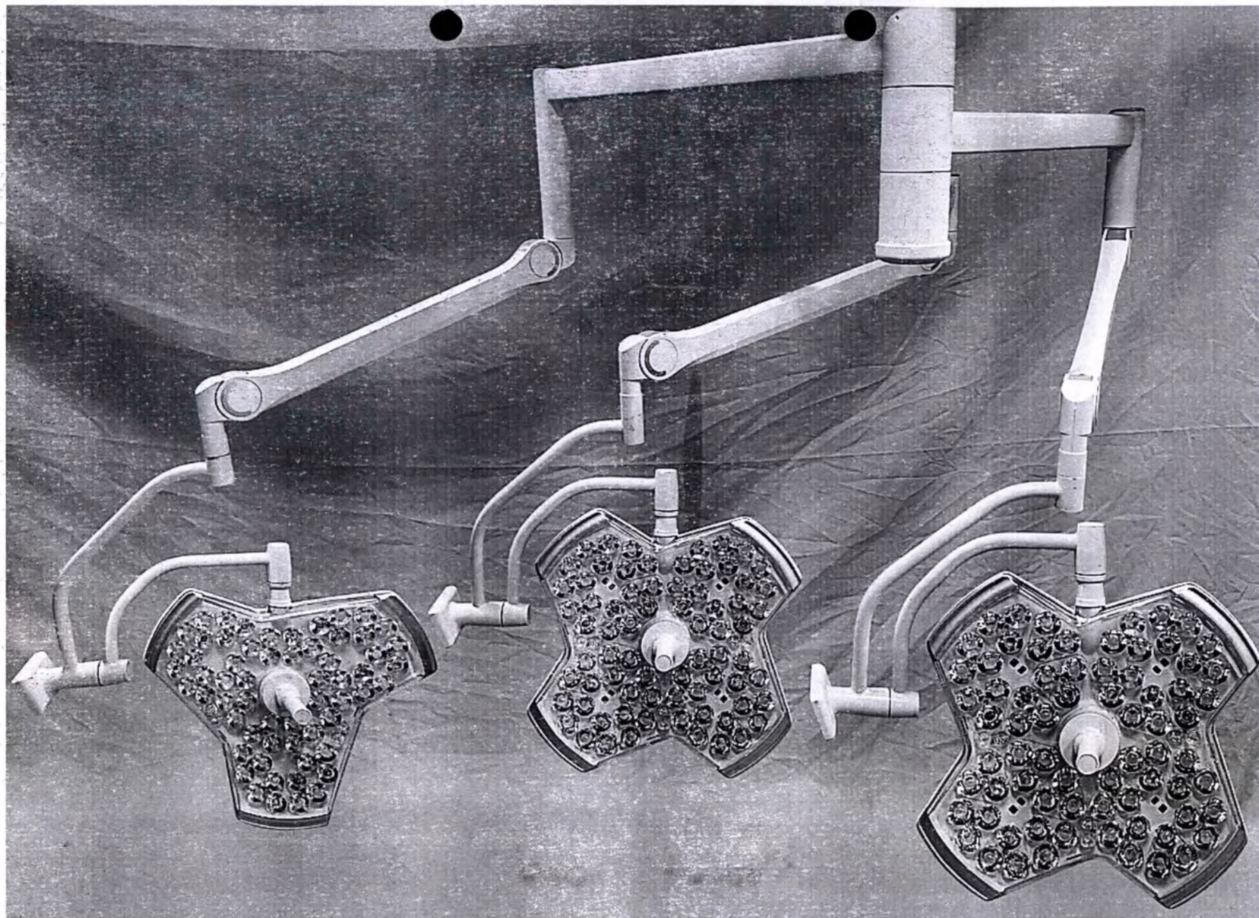
113. Светильник хирургический светодиодный HyLED X9/X9/X5/ HyLED X90/X90/X50 (блок осветительный X9/ X90 (2 шт.), блок осветительный X5/ X50 (1 шт.), панель управления сенсорная (3 шт.), рукоятка центральная multifunctional (3 шт.) и кронштейн
