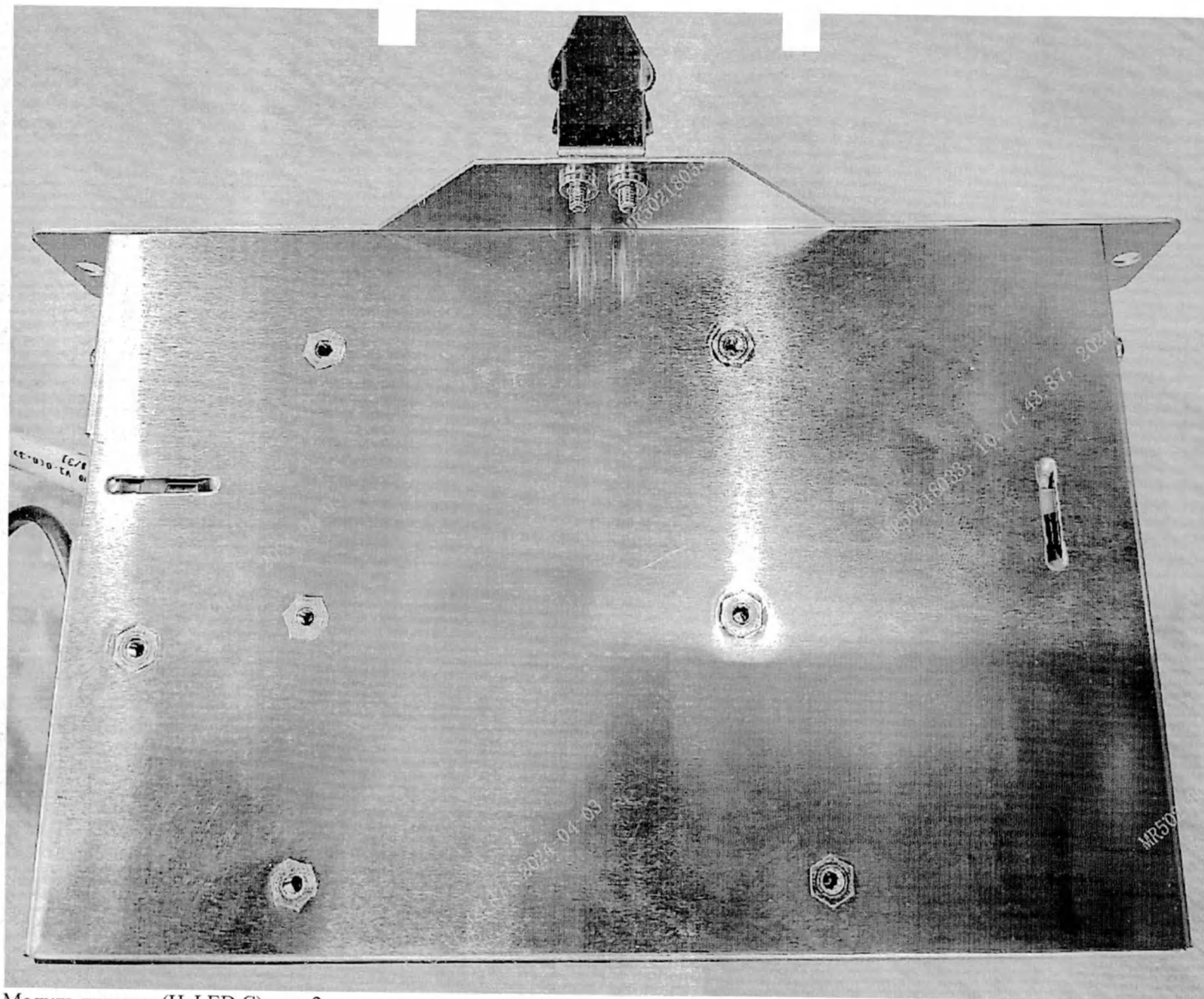
23. Модуль питания (HyLED C), тип 2
