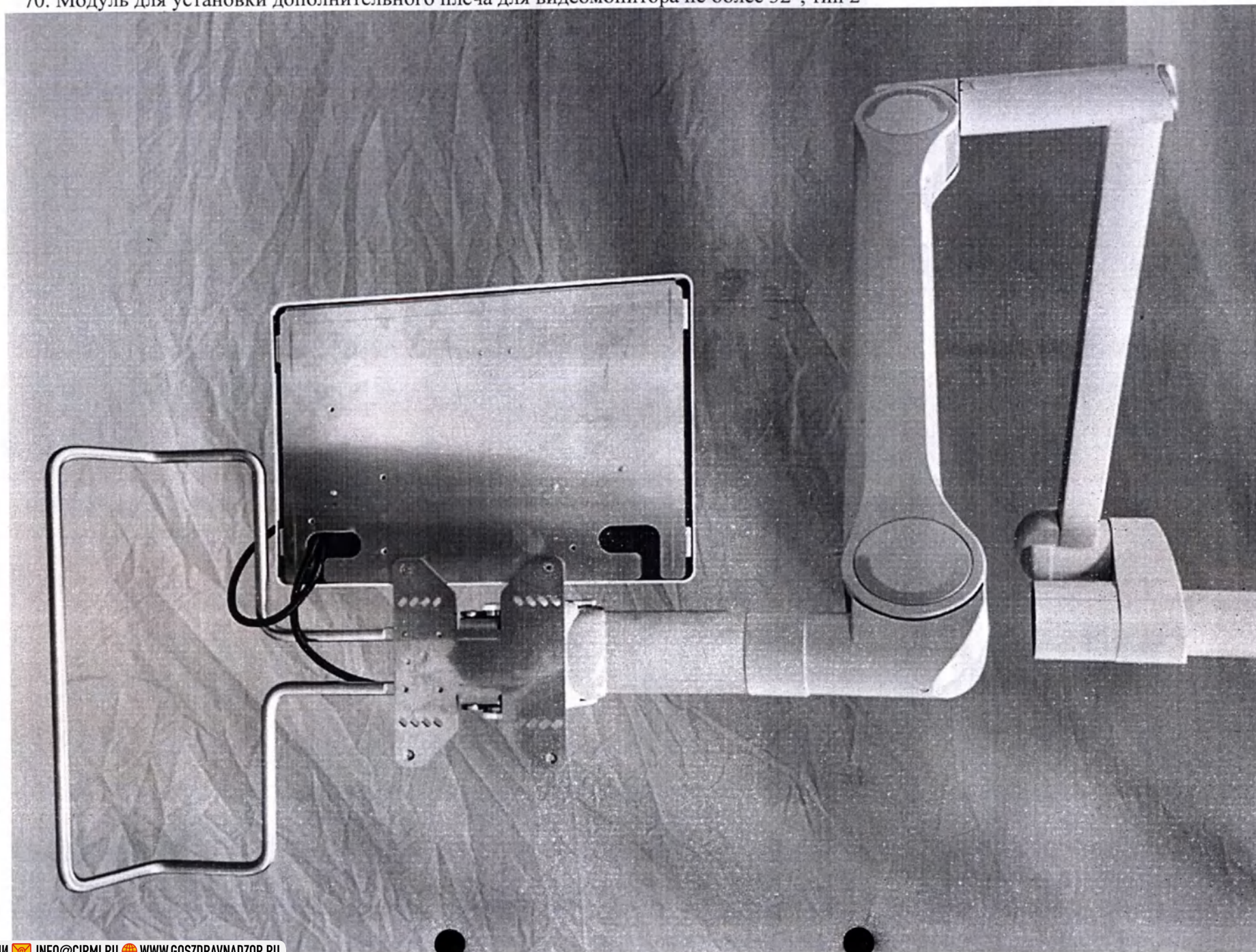
70. Модуль для установки дополнительного плеча для видеомонитора не более 32", тип 2
