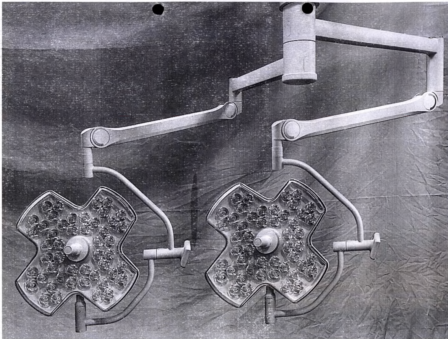
123. Светильник хирургический светодиодный HyLED C8/C8/ HyLED C80/C80 (блок осветительный C8/ C80 (2 шт.) с панелью ояткой центральной многофункциональной (2 шт.) и кронштейном пружинным стандартным (2 шт.))
