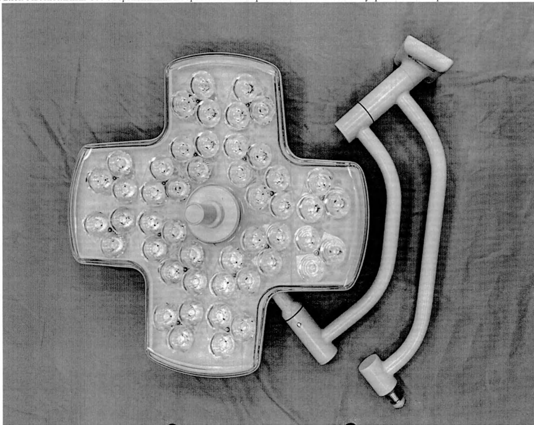
14. Блок осветительный С80 с вертикальным и горизонтальным кронштейнами и с панелью управления сенсорной
