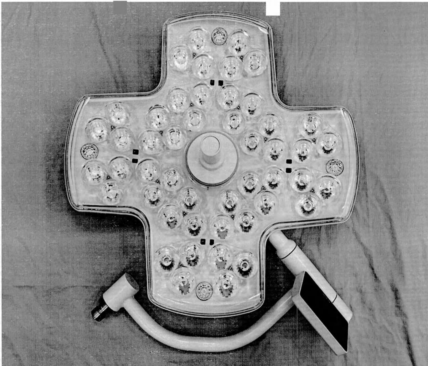
17. Блок осветительный C8 с вертикальным кронштейном и с панелью управления сенсорной (устанавливается вместе с кронштейном пружинным для использования в помещениях с низким потолком и в составе светильников хирургических светодиодных HyLED C8M)
