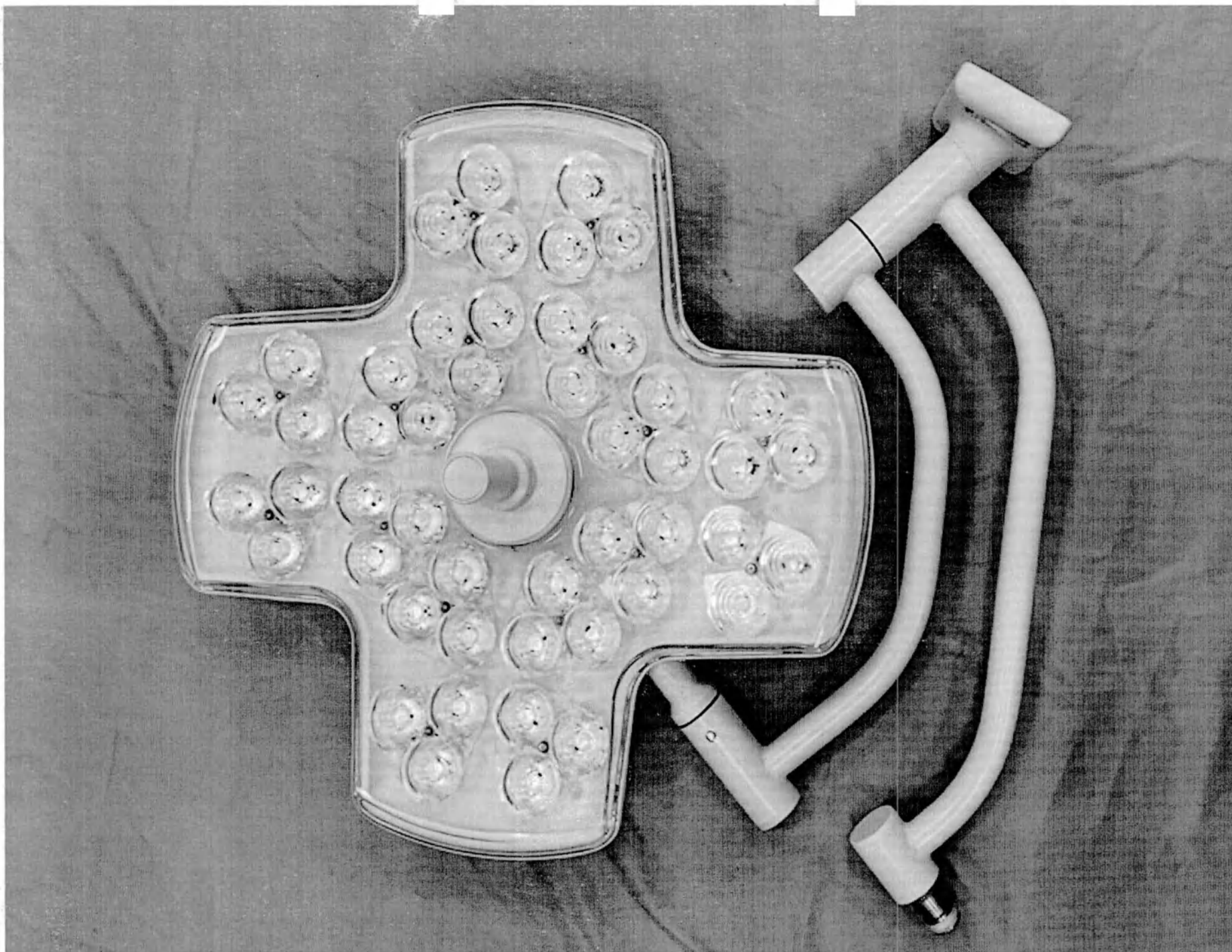
13. Блок осветительный С8 с вертикальным и горизонтальным кронштейнами и с панелью управления сенсорной
