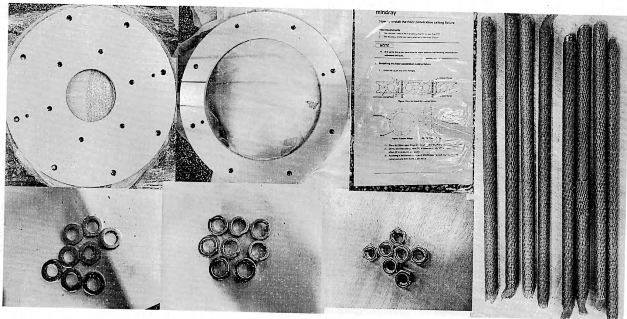
65. Система потолочного крепления сквозная, металлическая разобранная
