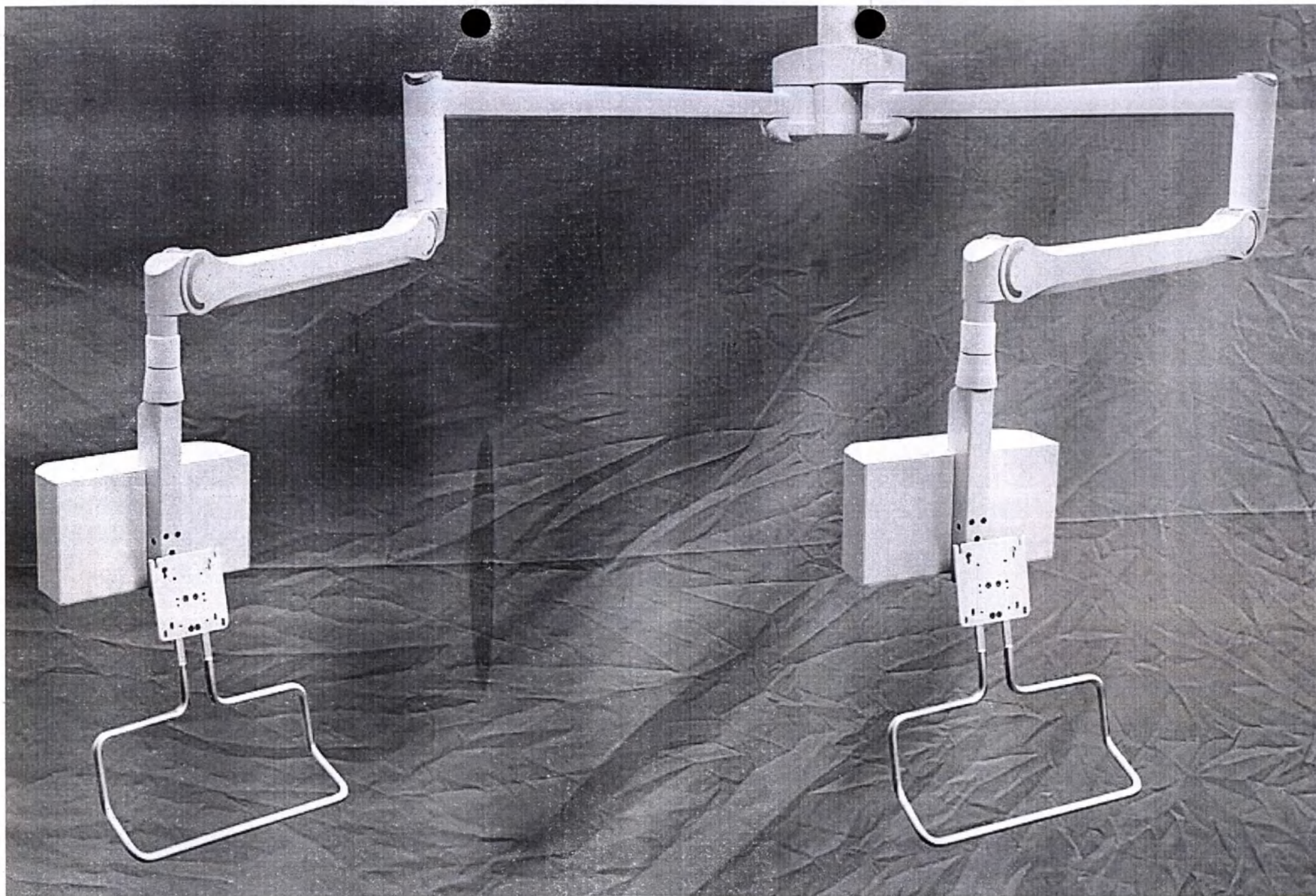
75. Модуль для установки двух дополнительных плеч для двух видеомониторов не более 27"
