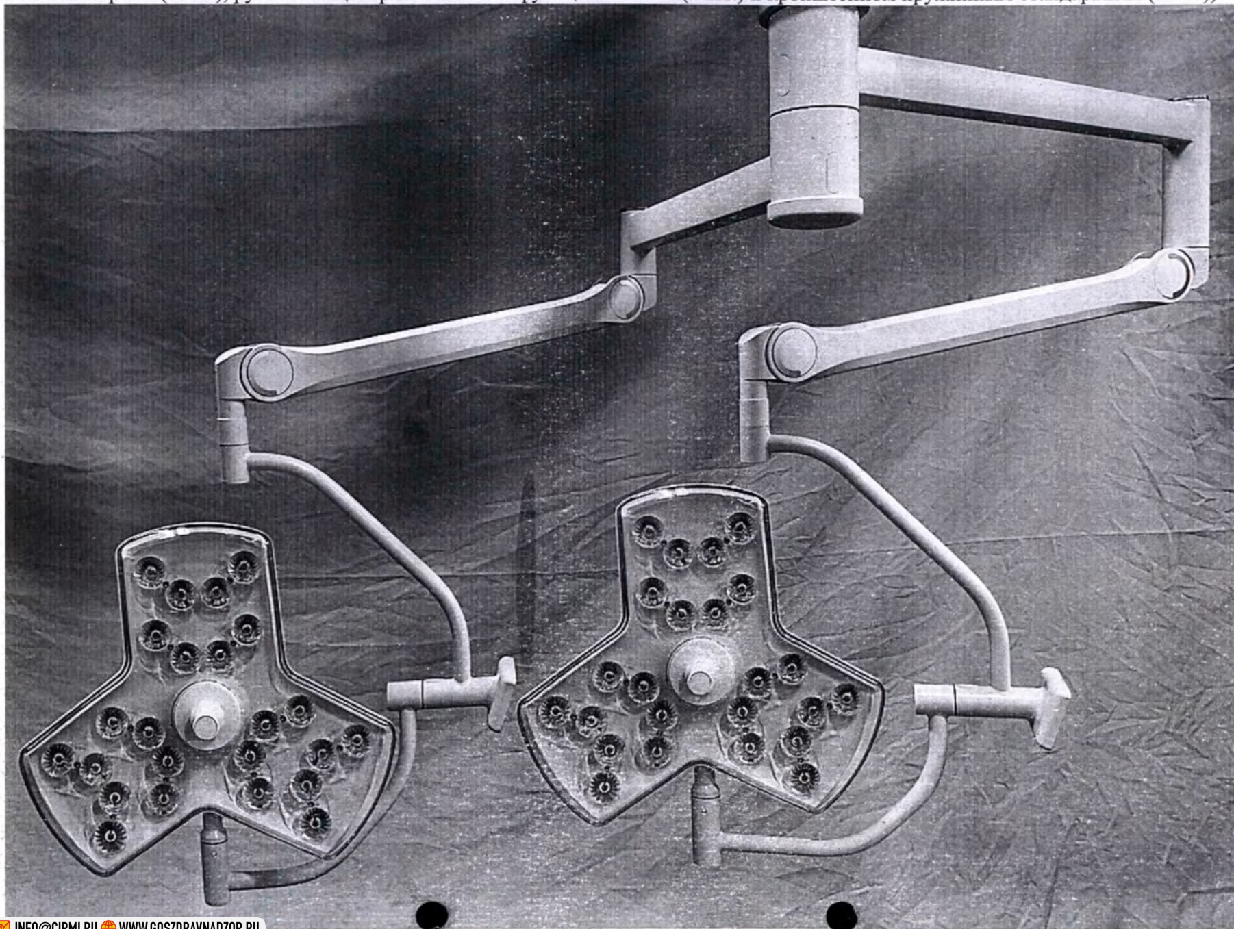
118. Светильник хирургический светодиодный HyLED C5/C5/ HyLED C50/C50 (блок осветительный C5/ C50 (2 шт.) с панелью управления сенсорной (2 шт.), рукояткой центральной многофункциональной (2 шт.) и кронштейном пружинным стандартным (2 шт.))
