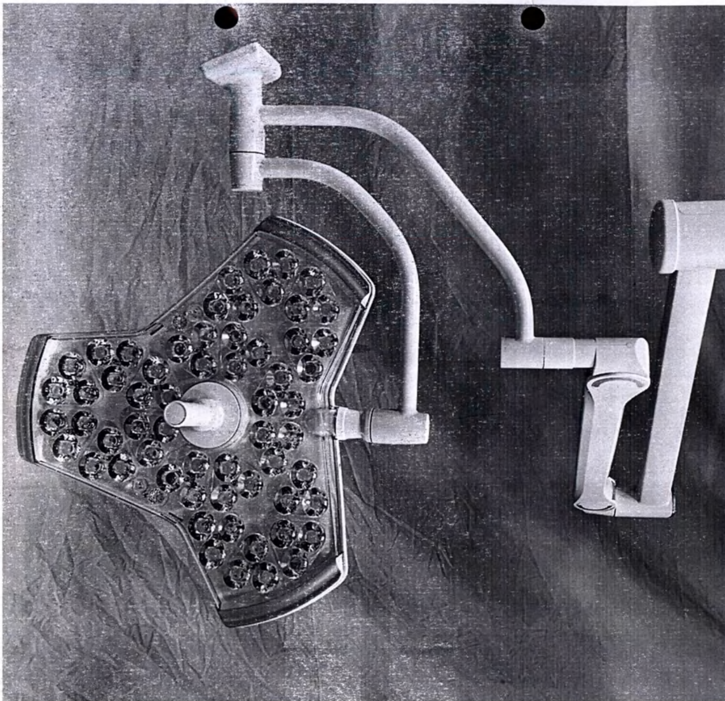
107. Светильник хирургический светодиодный HyLED X5/ HyLED X50 (блок осветительный X5/ X50 с панелью управления сенсорной, кциональной и кронштейном пружинным стандартным)
