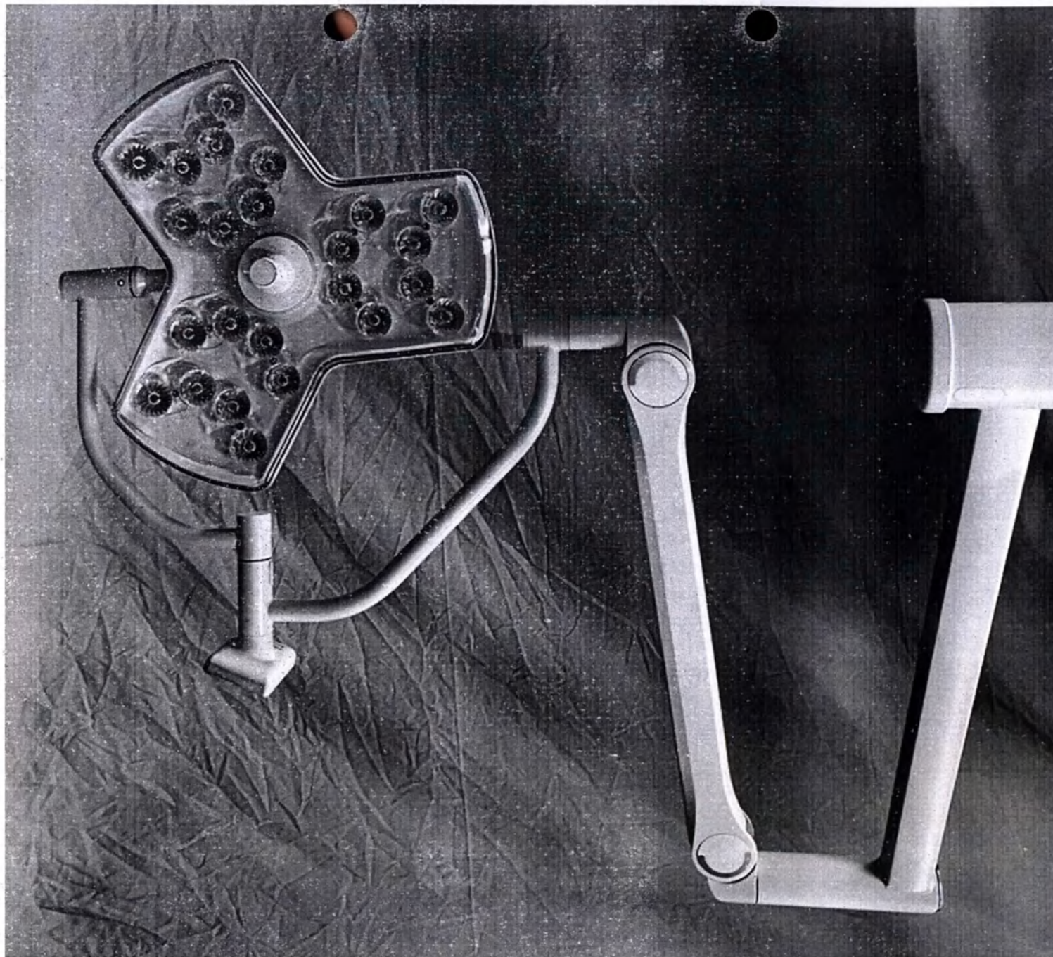
115. Светильник хирургический светодиодный HyLED C5/ HyLED C50 (блок осветительный C5/ C50 с панелью управления сенсорной,
