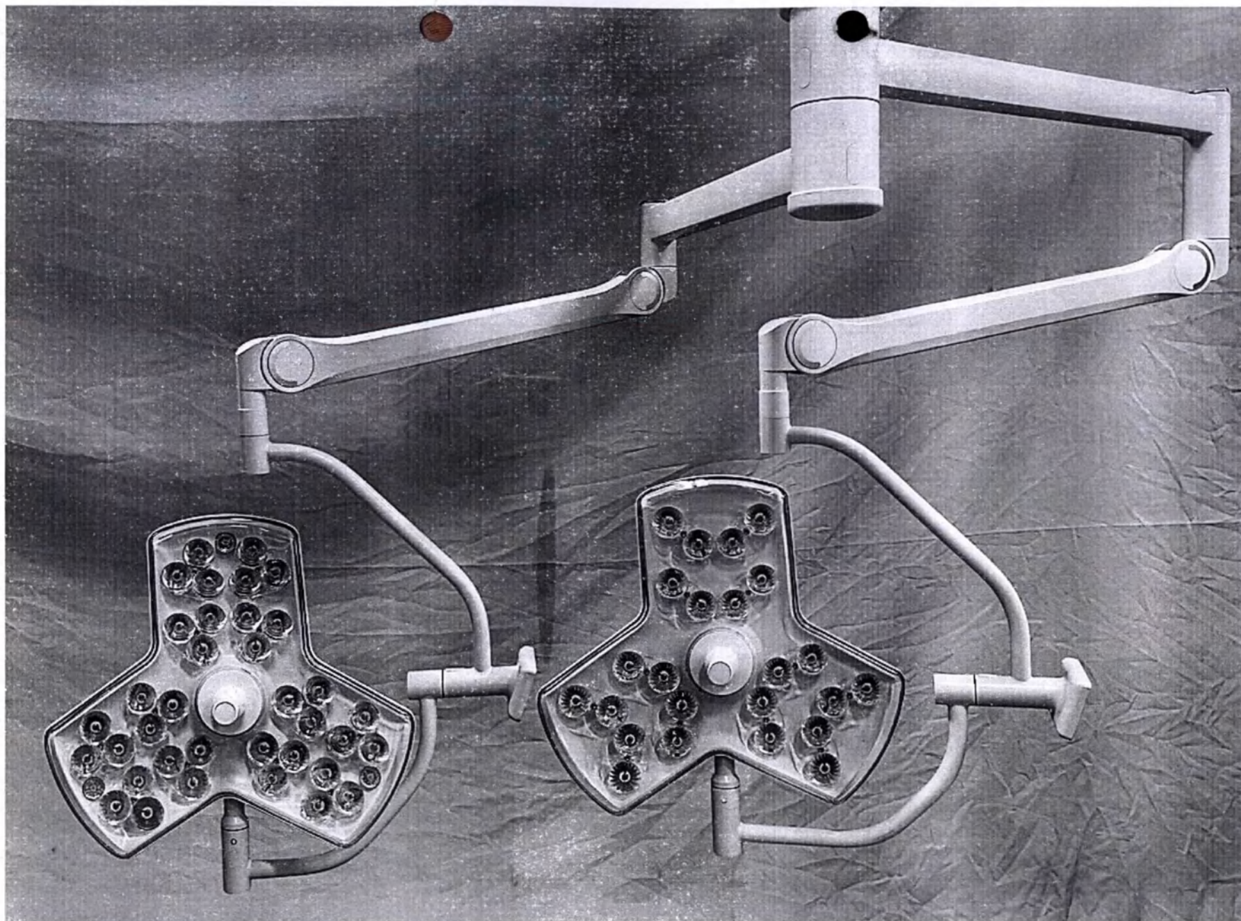
119. Светильник хирургический светодиодный HyLED C7/C5/ HyLED C70/C50 (блок осветительный C7/ C70 (1 шт.), блок осветительный C5/ C50 (1 шт.), панель управления сенсорная (2 шт.), рукоятка центральная multifunctional (2 шт.) и кронштейн
