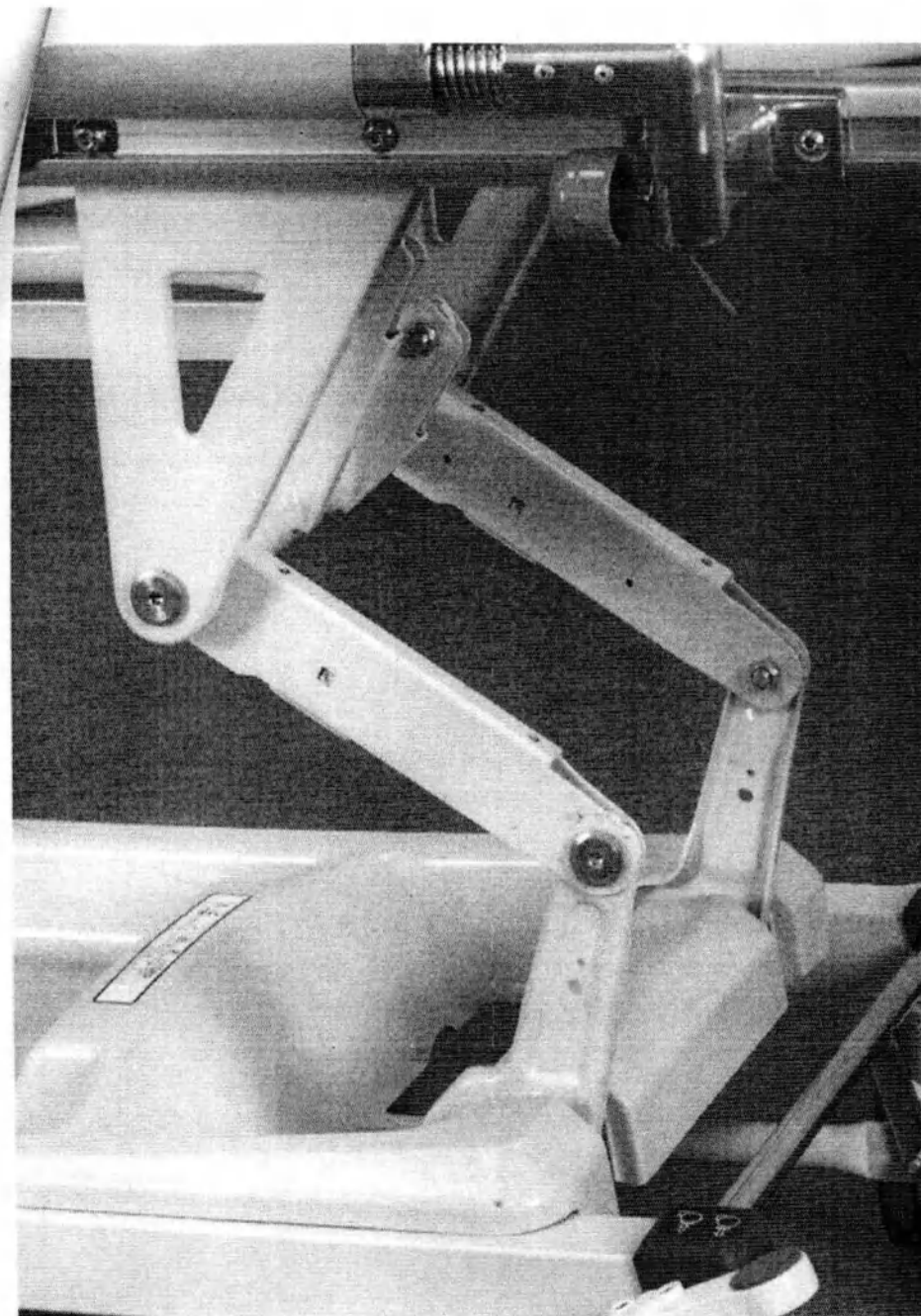
Подъемный механизм. Общий вид.
