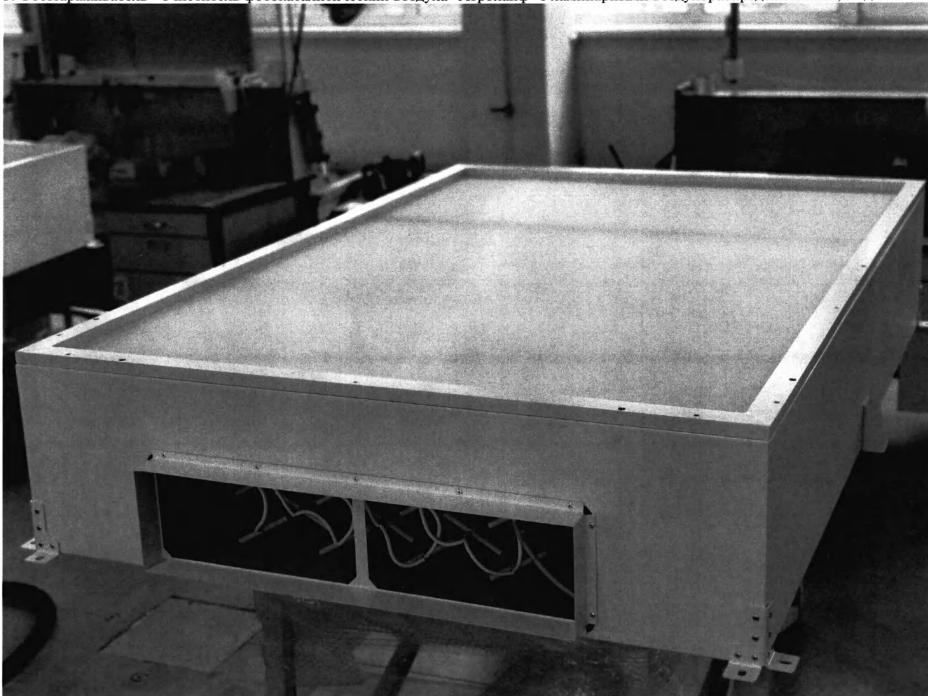
3. Обеззараживатель - очиститель фотокаталитический воздуха "Аэролайф" с ламинарными воздухораспределителями, модель ЛАМ 1401
