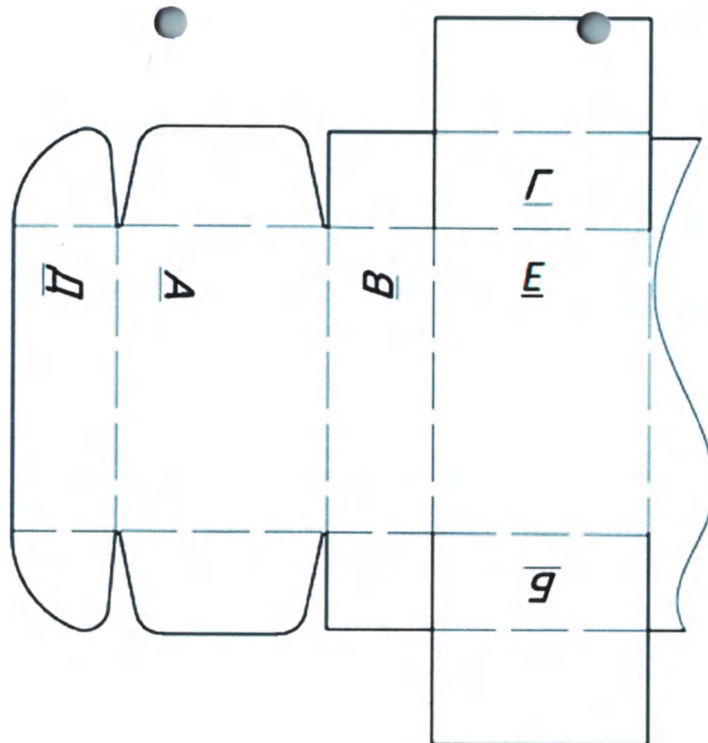
Маркировка коробки СА (развертка коробки).
