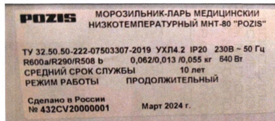
МАРКИРОВКА МОРОЗИЛЬНИКА
