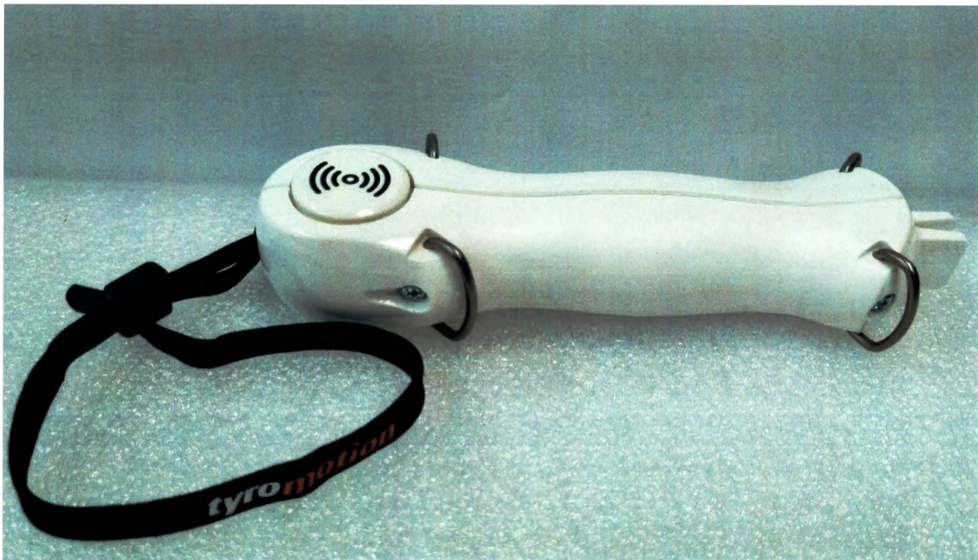
Рукоятка сенсорная PABLO (с предохранительным ремнем)
