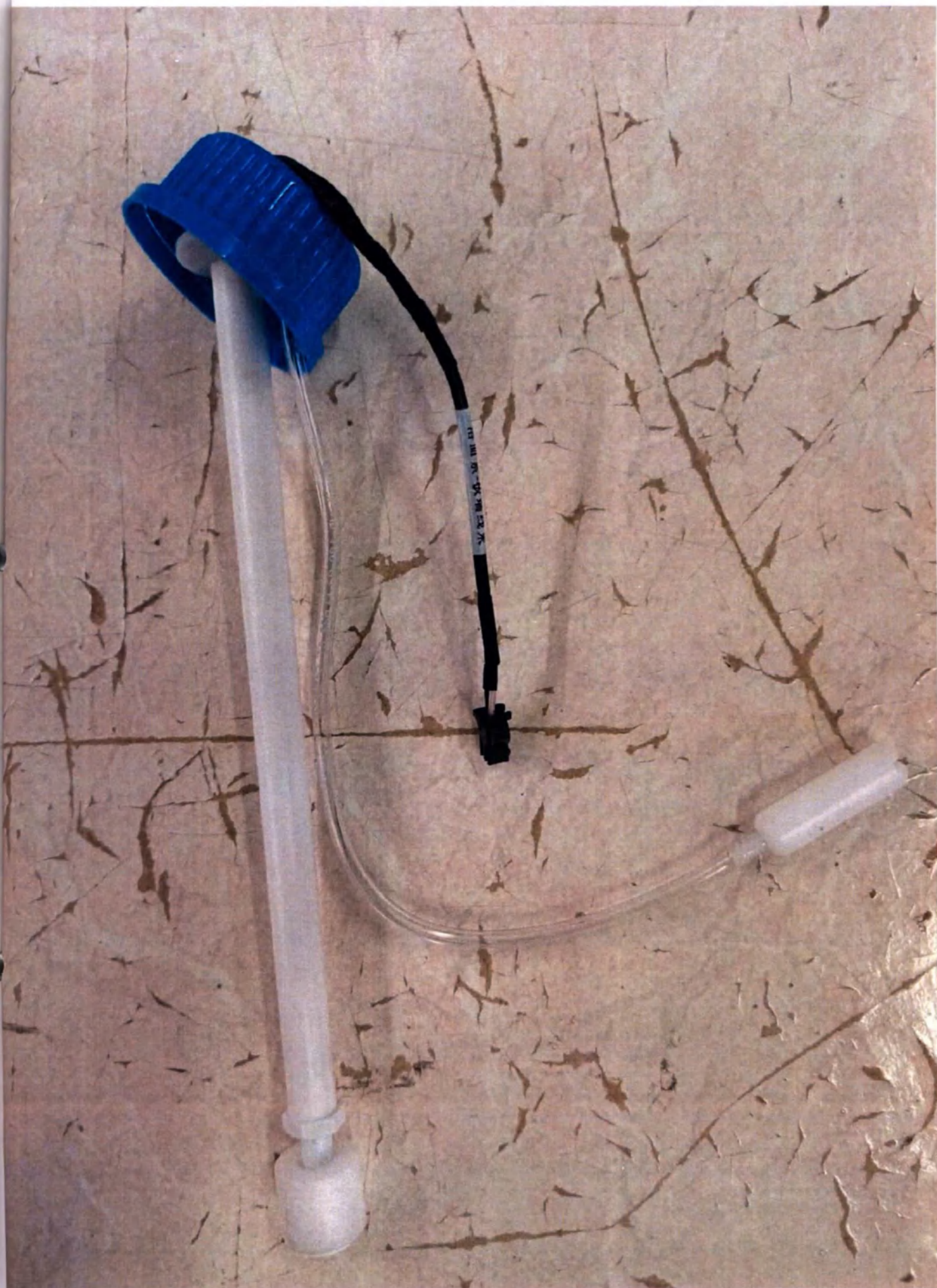
рышка для бутылки лизирующего раствора в сборе (MCC-1000-004)
