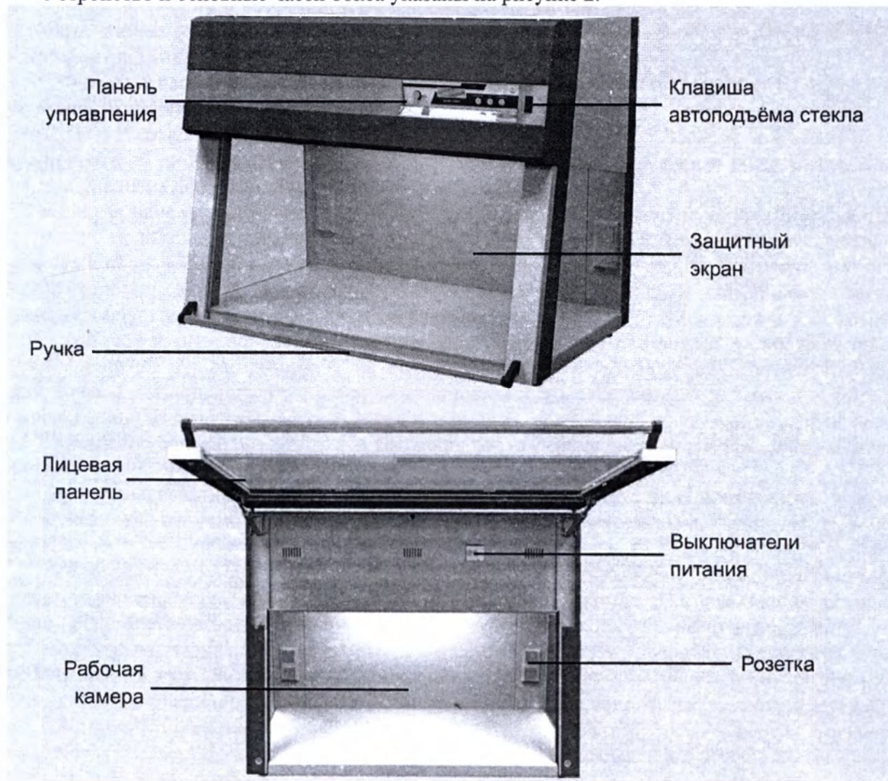
Рисунок 2 – Устройство и основные части бокса (вид спереди)
