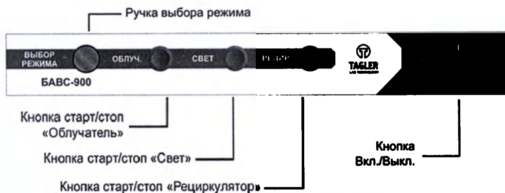
Рисунок 3 – Панель управления бокса
