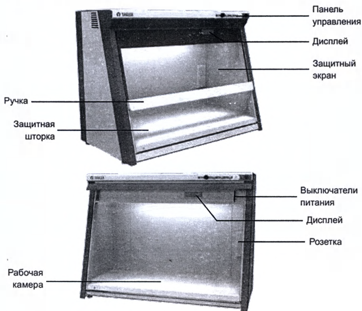
Рисунок 2 – Устройство и основные части бокса (вид спереди) На рисунке 3 представлена панель управления изделием
