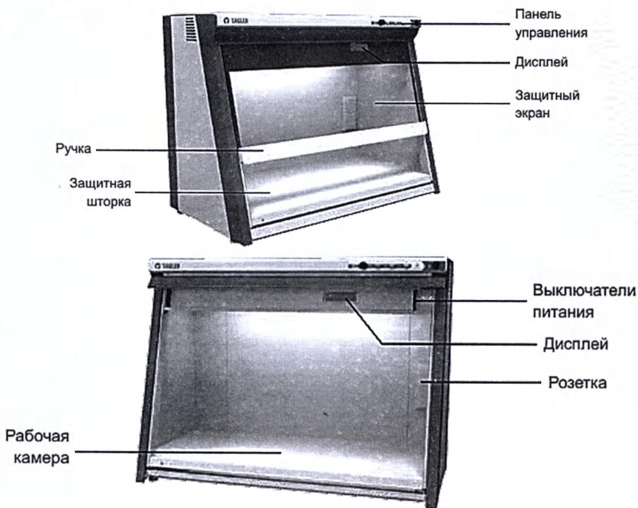
Рисунок 2 – Устройство и основные части бокса (вид спереди) На рисунке 3 представлена панель управления изделием.
