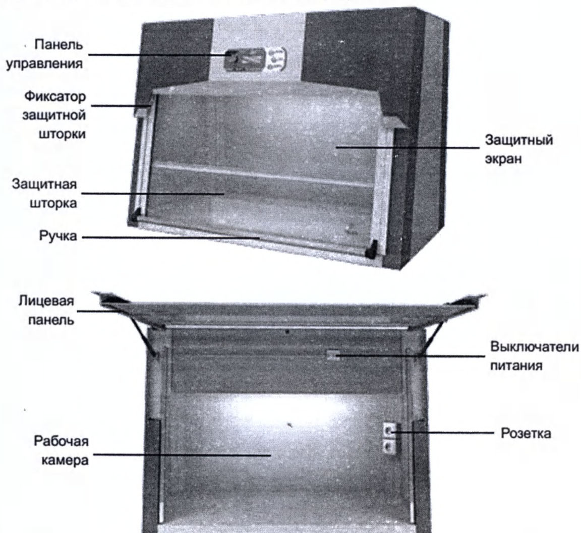
Рисунок 2 – Устройство и основные части бокса (вид спереди) На рисунке 3 представлена панель управления изделием.
