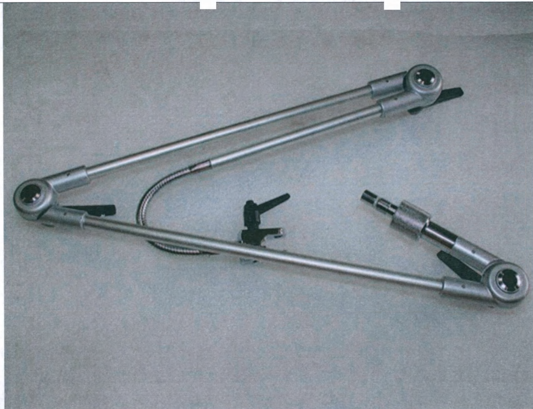
4. Шарнирный держатель дыхательного контура
