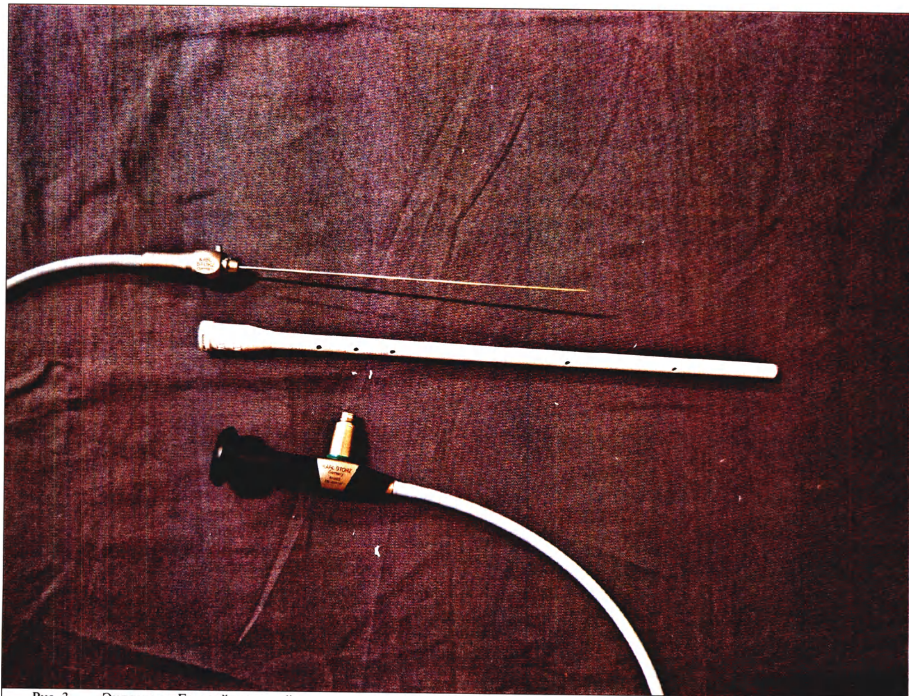
Рис. 3. Эндоскоп с Гильзой защитной
