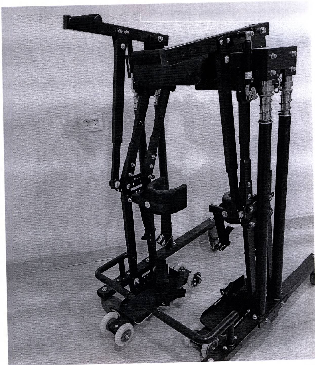
Вид спереди
