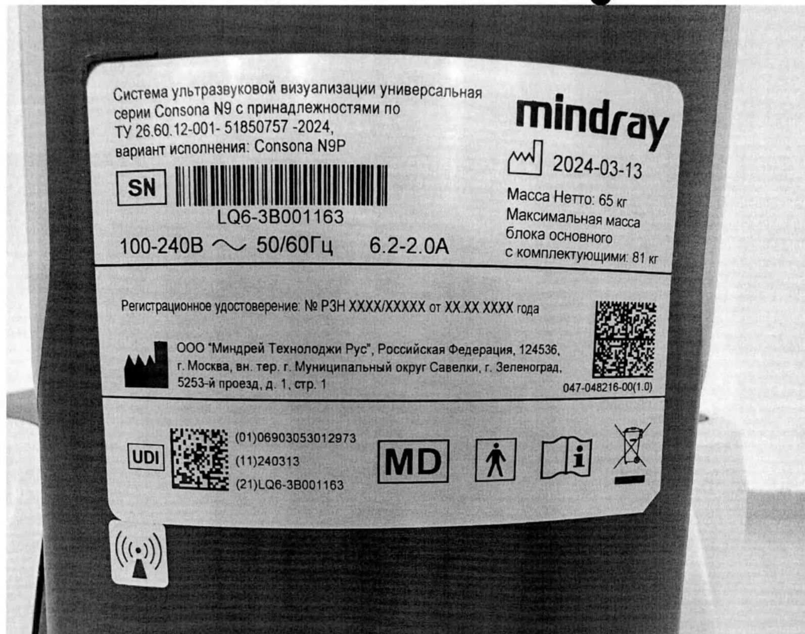
Вариант исполнения: Consona N9P по ТУ 26.60.12-002-51850757 -2024. Блок основной, Этикетка на корпусе.
