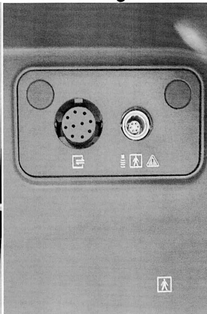
Порт для ввода и вывода ЭКГ сигнала, порт для подключения датчиков ультразвуковых кардиальных
