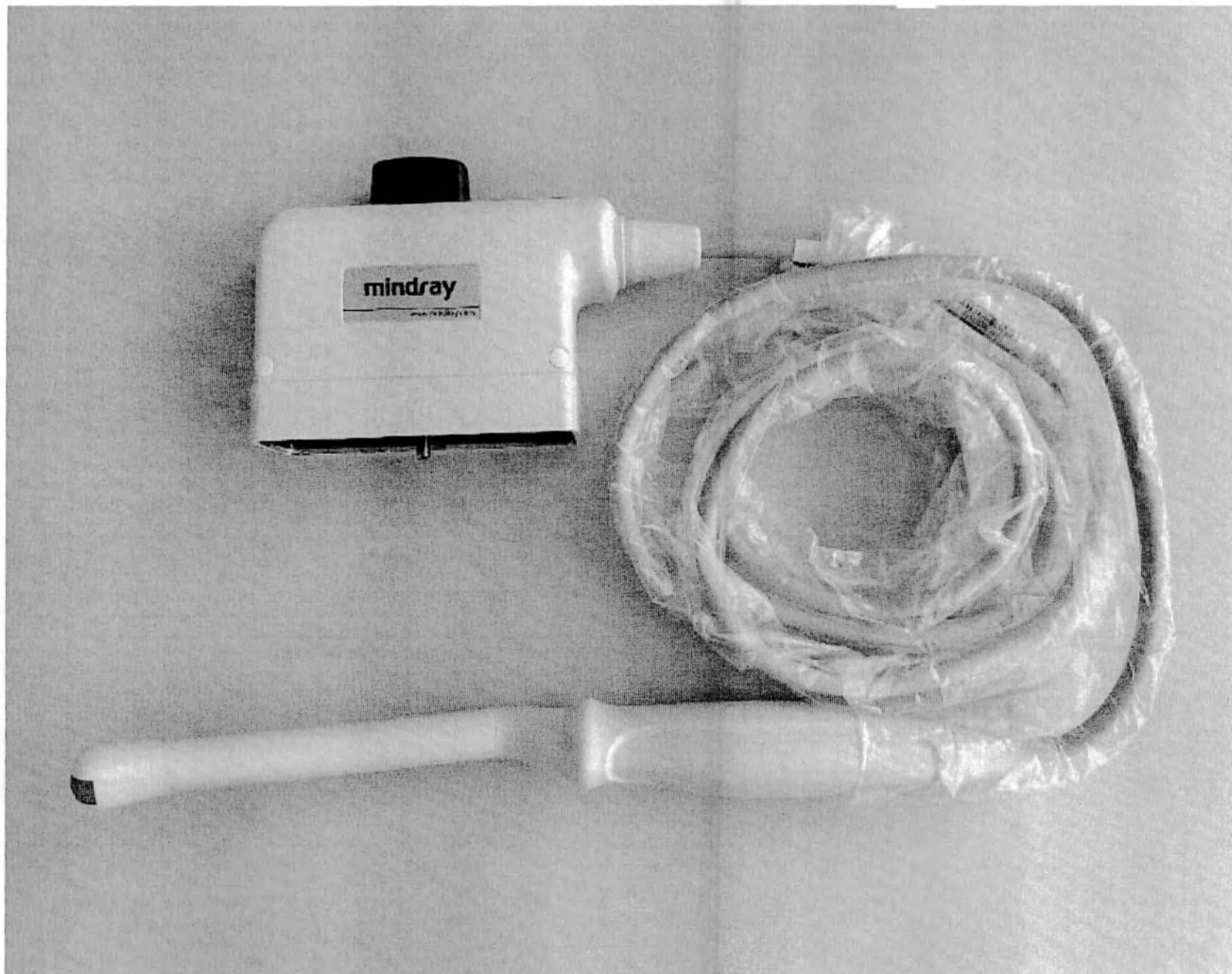
Датчик ультразвуковой микроконвексный внутривидовой V10-4B
