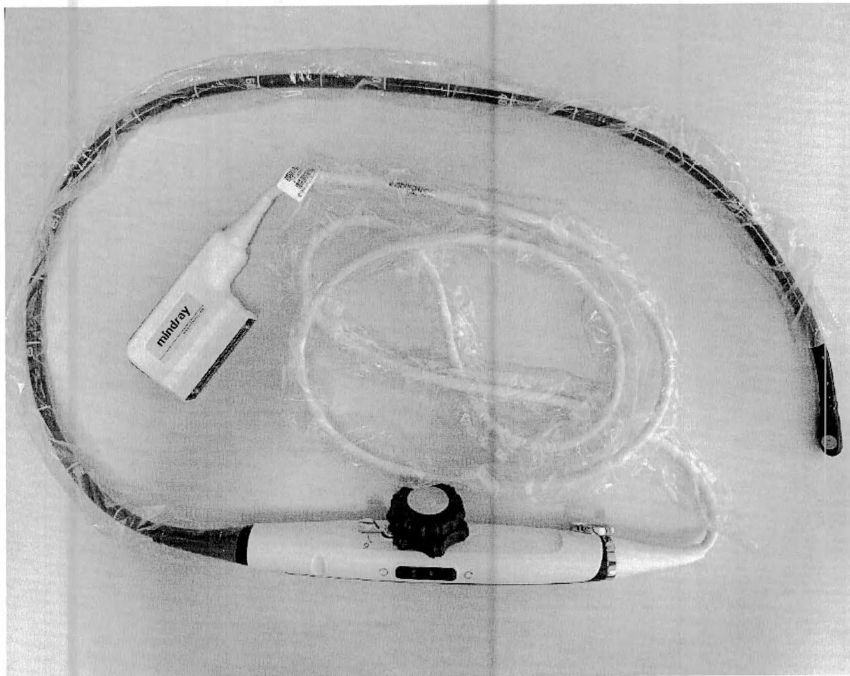
Датчик ультразвуковой секторный фазированный чреспищеводный Р8-2Ts, в составе: Датчик ультразвуковой секторный фазированный чреспищеводный Р8-2Ts
