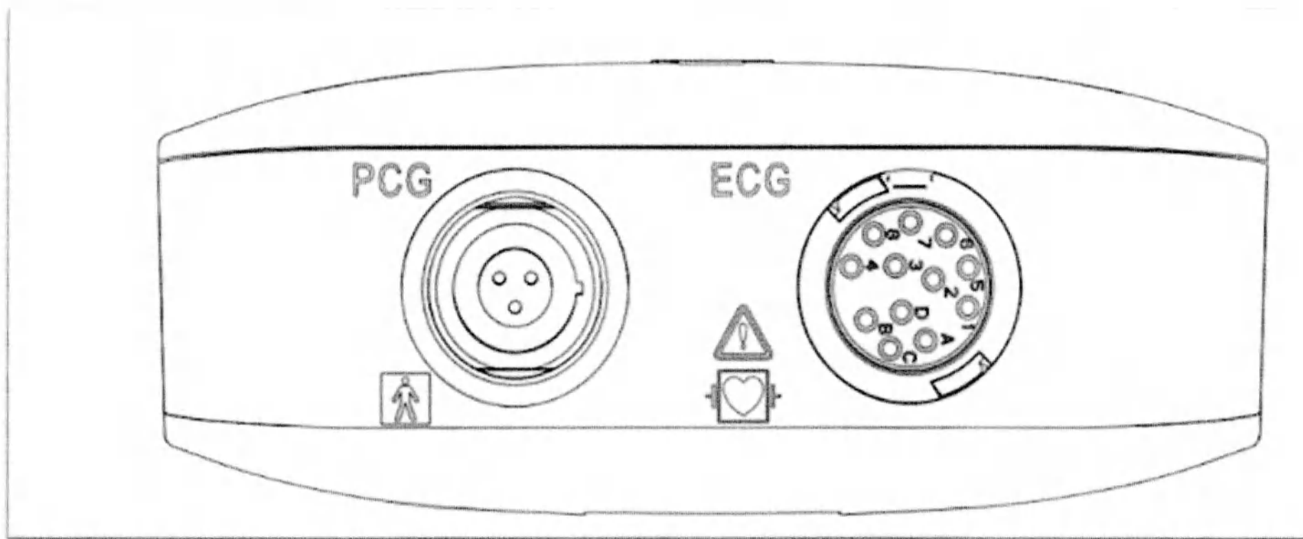
Модуль ЭКГ (ECG Module), модель ECG-43. Маркировка электрических разъёмов
