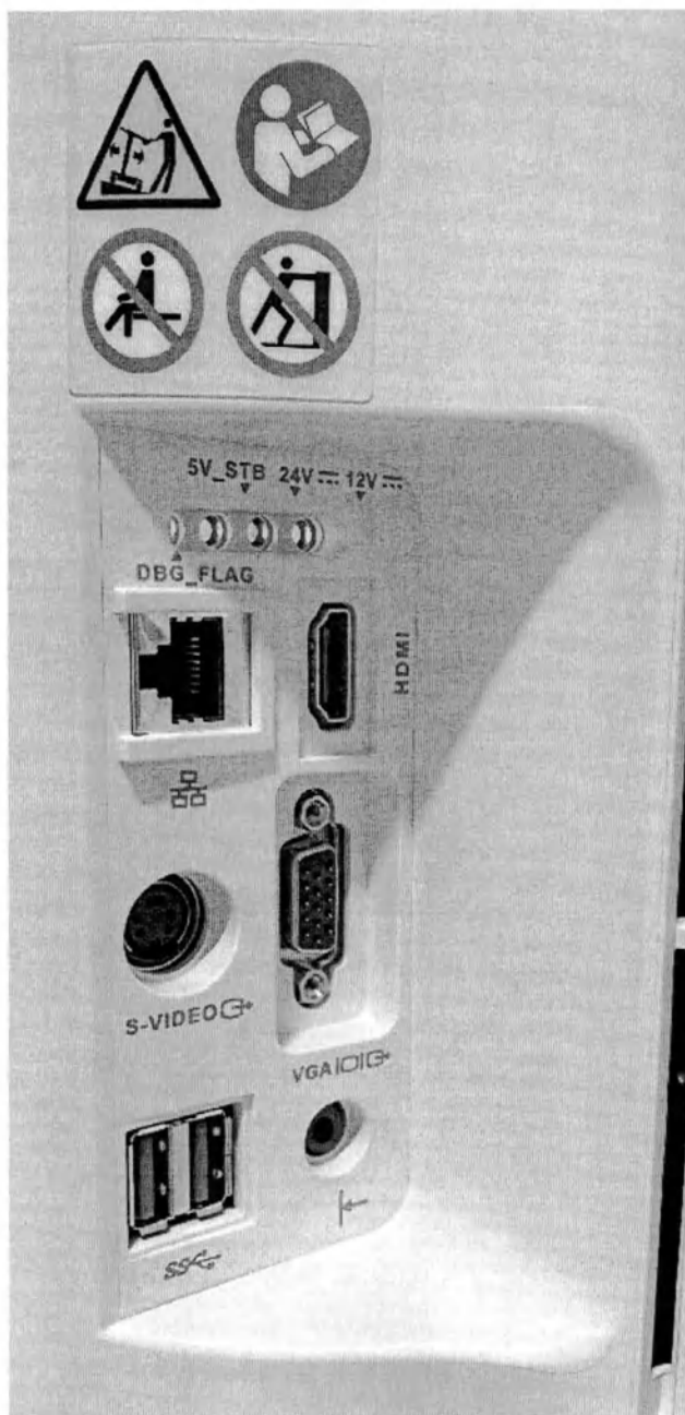
Блок основной. Задняя панель ввода/вывода
