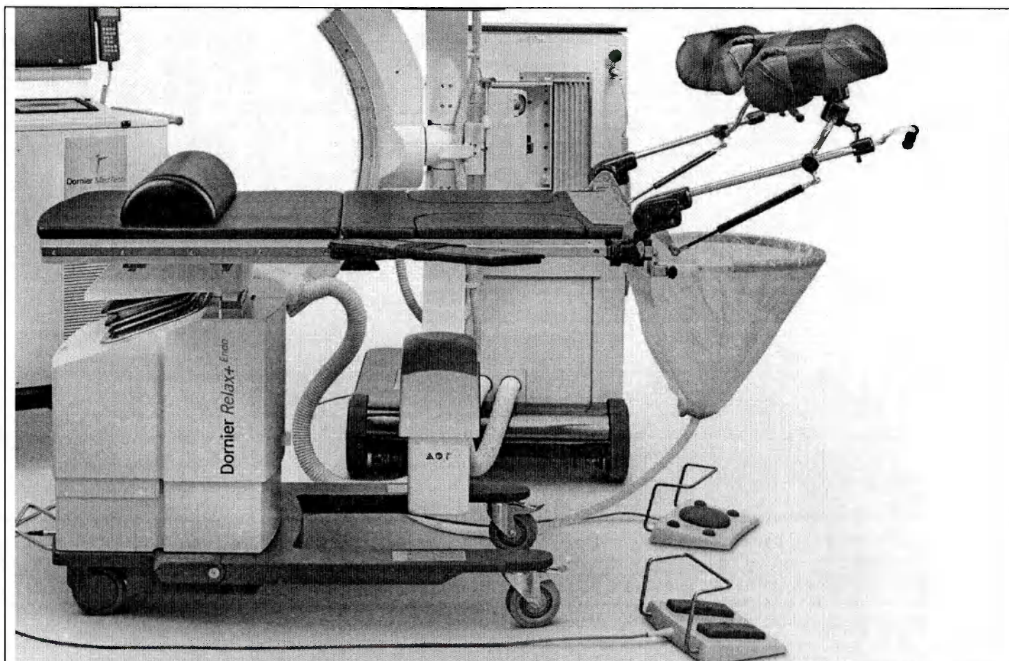
Стол пациента
