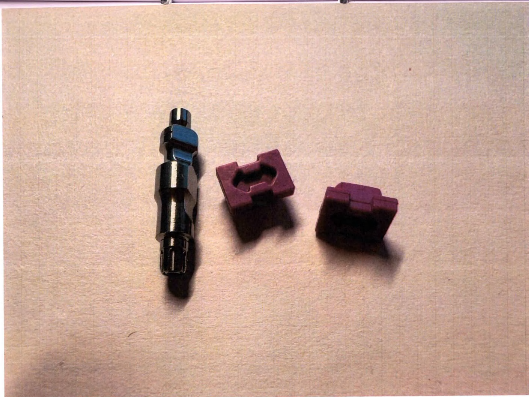
«Трансфер слепочный для циркониевых имплантатов, с прямым интерфейсом (ZIRCONIA IMPLANT EXACT IMPRESSION COPING), артикул: 108.186»
