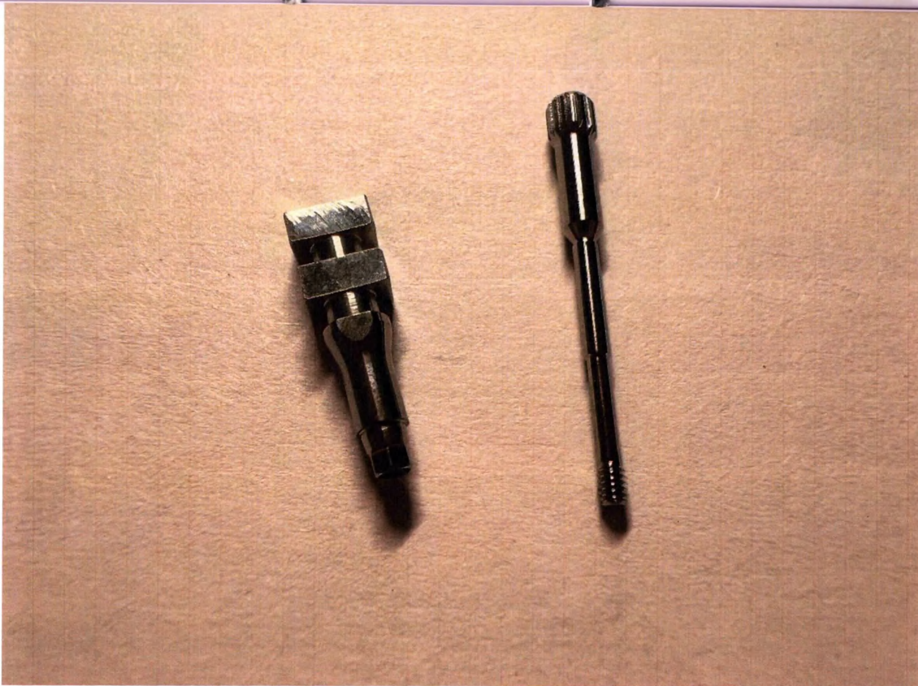
«Трансфер слепочный для тонких имплантатов GM для открытой ложки, с прямым интерфейсом (NGM EXACT IMPLANT IMPRESSION COPING OPEN TRAY), артикул: 108.204»
