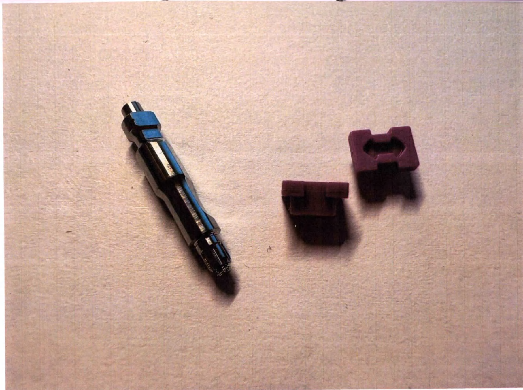
«Трансфер слепочный для циркониевых имплантатов длинный, с прямым интерфейсом (ZIRCONIA IMPLANT EXACT IMPRESSION COPING (LONG)), артикул: 108.187»
