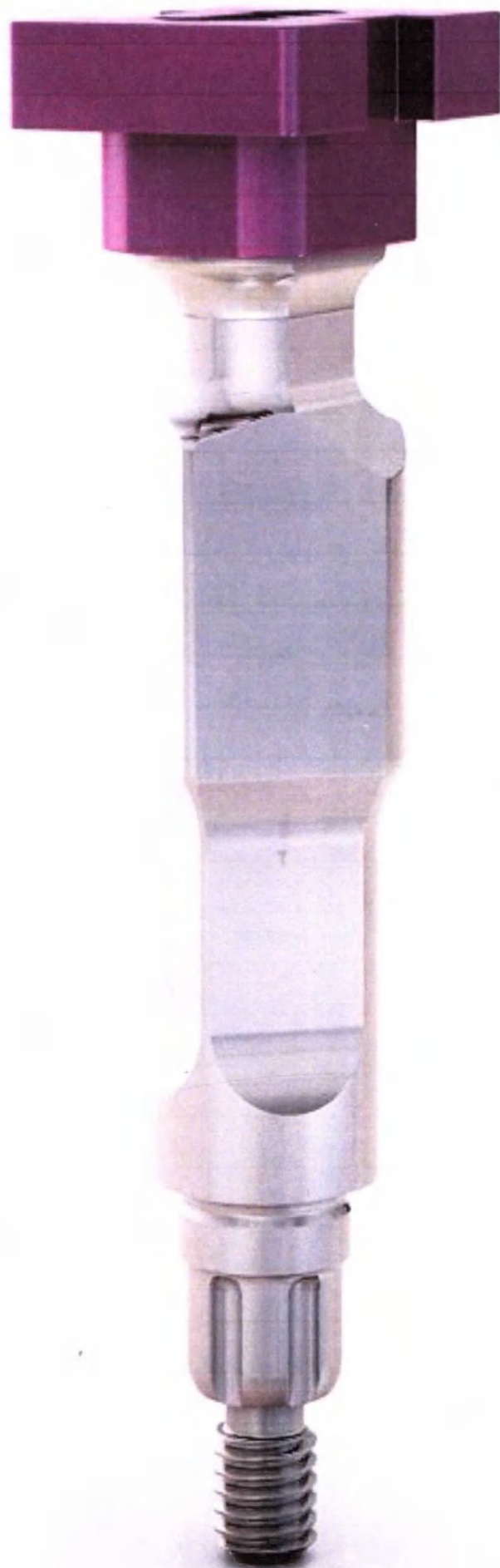
Трансфер слепочный для циркониевых имплантатов длинный, с прямым интерфейсом (ZIRCONIA IMPLANT EXACT IMPRESSION COPING (LONG)), артикул: 108.187
