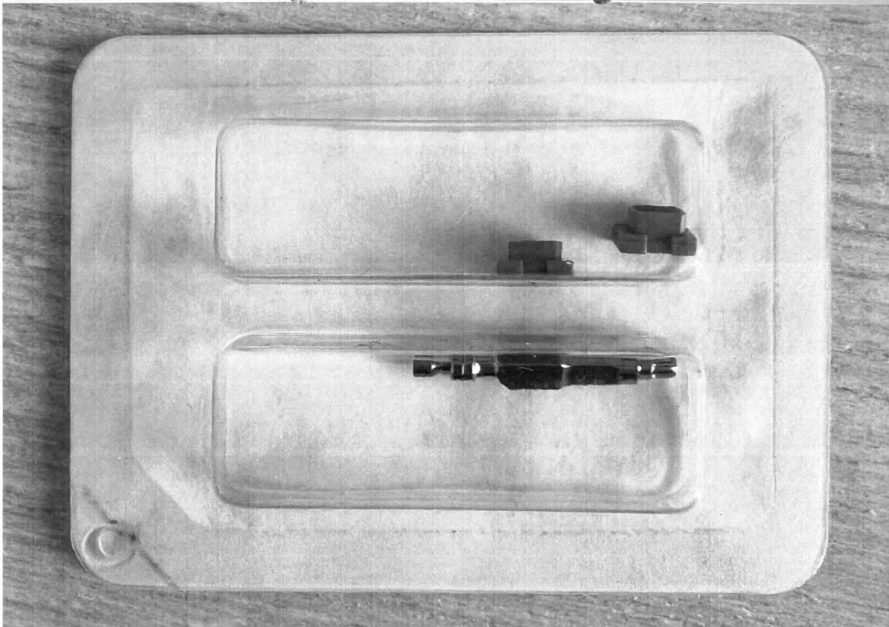
Первичная упаковка с двумя секциями на примере «Трансфер слепочный для циркониевых имплантатов длинный, с прямым интерфейсом (ZIRCONIA IMPLANT EXACT IMPRESSION COPING (LONG)), артикул: 108.187»
