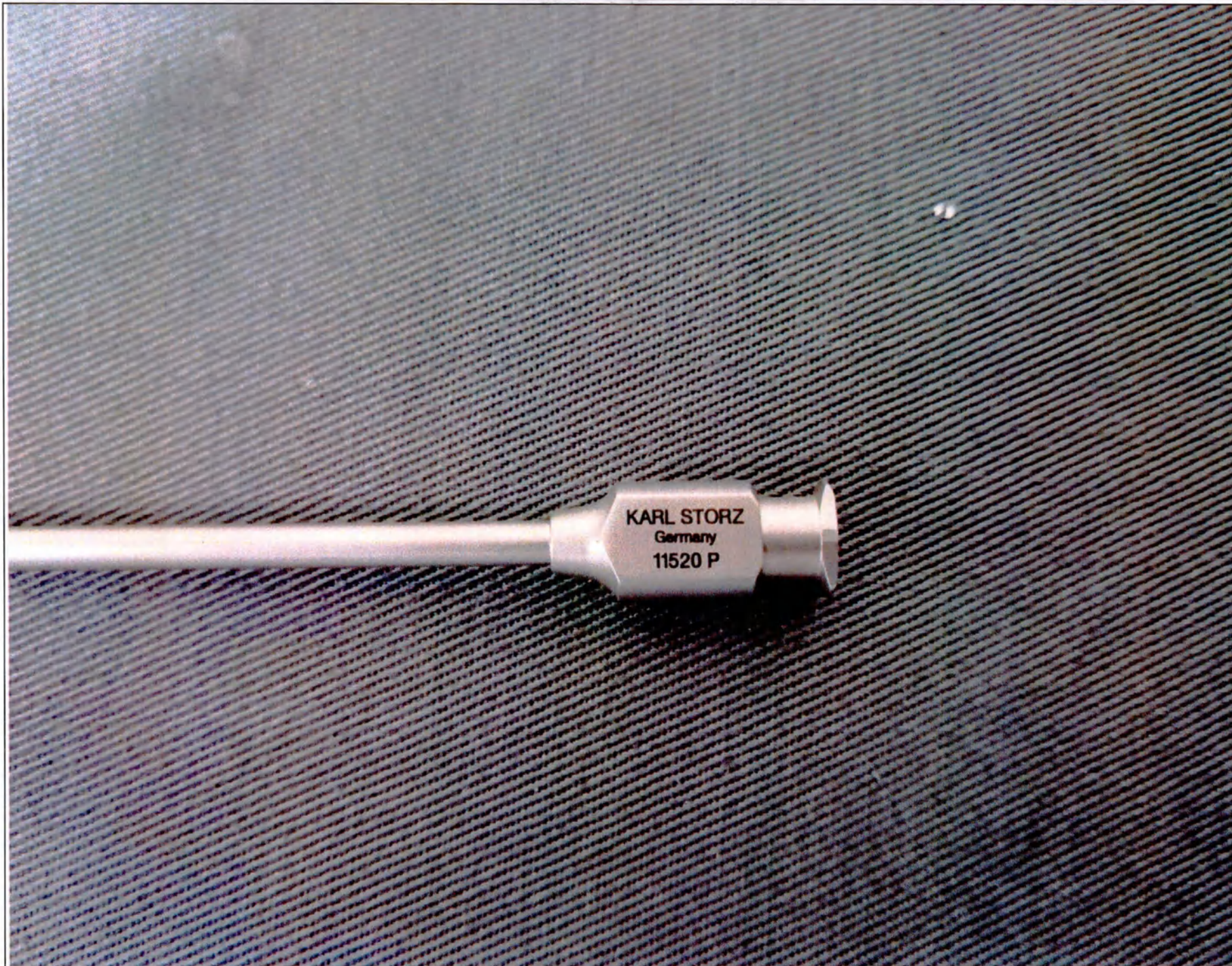
Рис. 9. Гильза защитная, для эндоскопов с рабочей длиной 10-12 см
