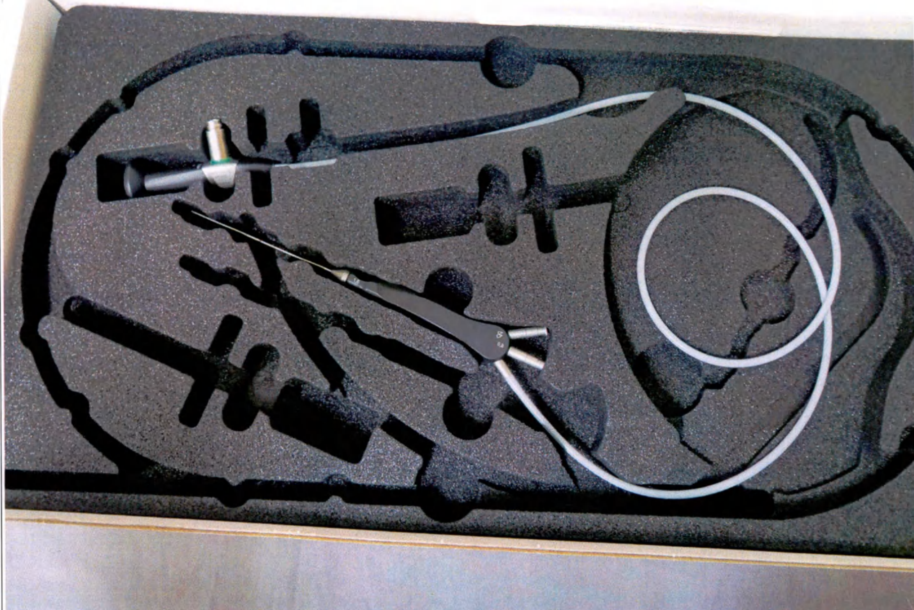
Рис. 20. Эндоскоп жесткий миниатюрный для сиаэндоскопии, направление наблюдения 0^\circ , диаметр 1,7 мм, рабочая длина 10 см, длина 140 см
