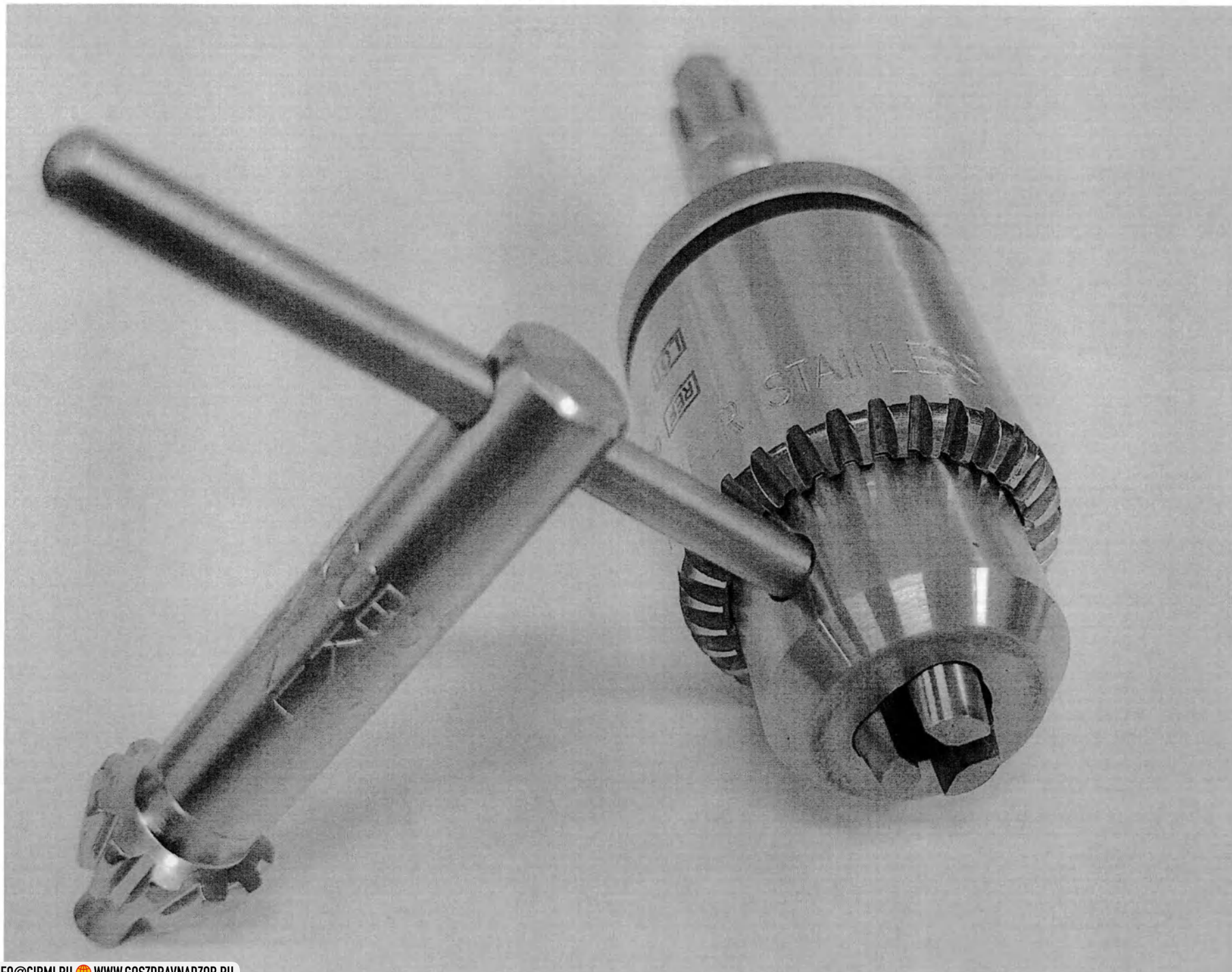
8. Патрон кулачковый 1/4" JACOBS с ключом для дрели хирургической аккумуляторной GDP I
