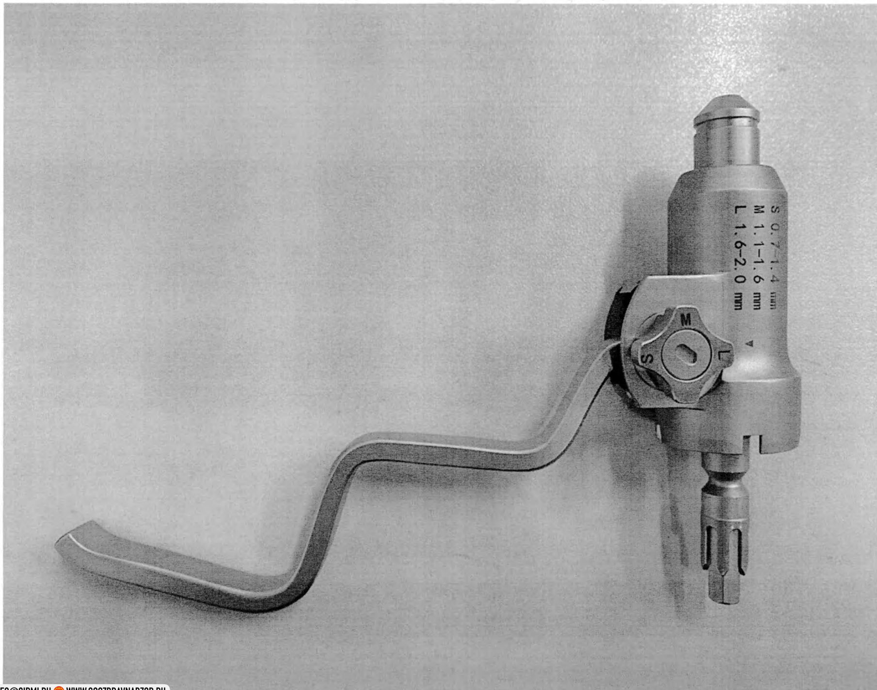
15. Патрон цанговый для спиц Киршнера для дрели хирургической аккумуляторной GDP I, размером: 0,7-2,0 мм
