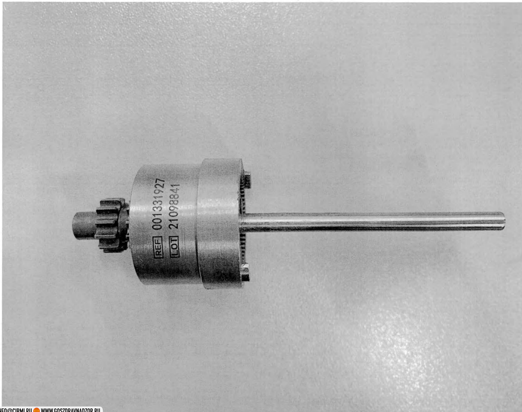
Ремонтный модуль для дрели хирургической аккумуляторной GDP I – Коробка передач
