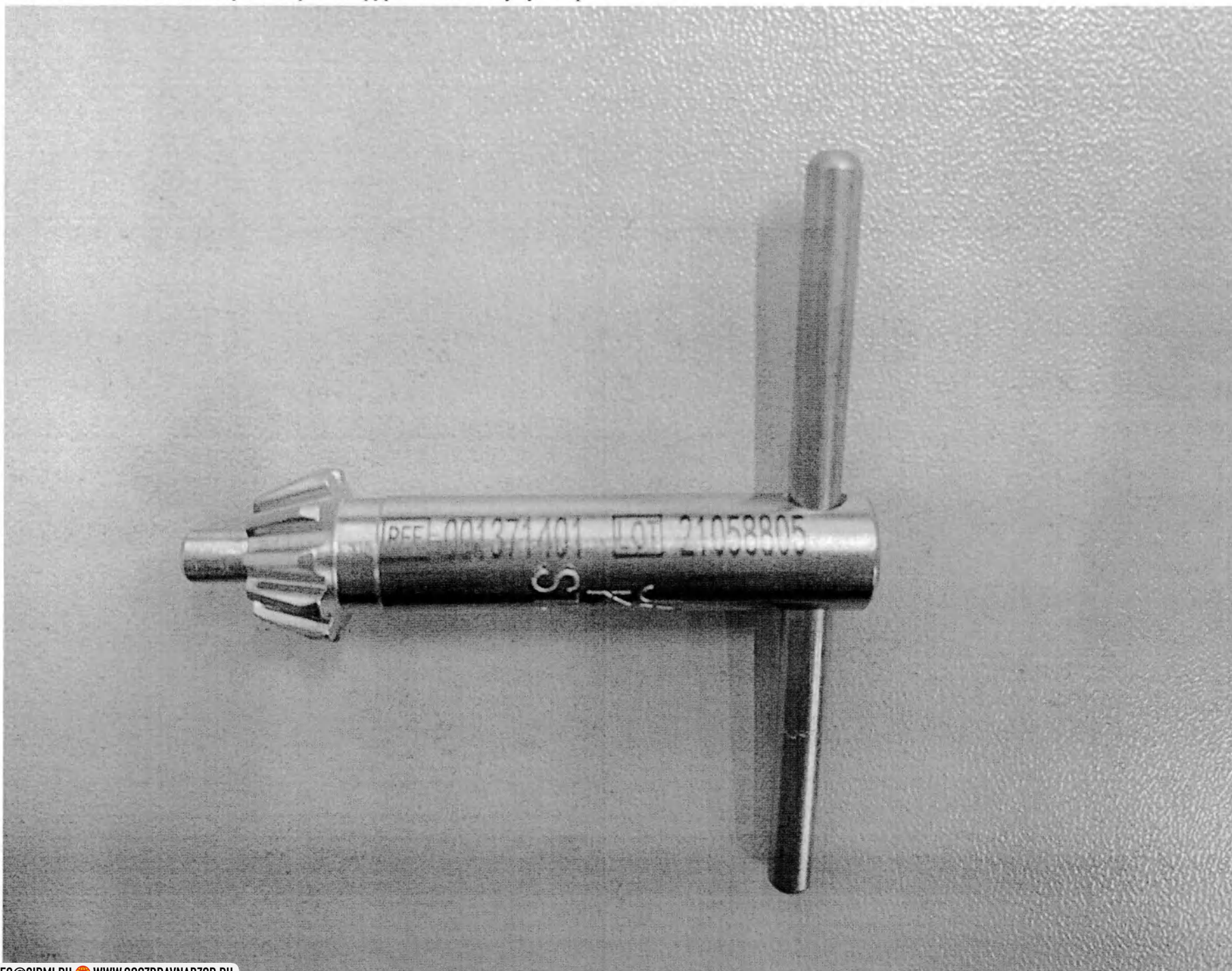
18. Ключ JACOBS для патронов дрели хирургической аккумуляторной GDP I
