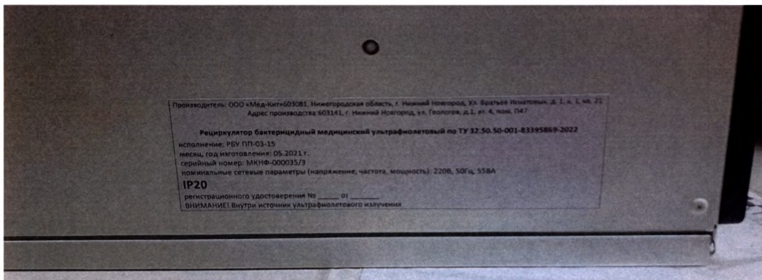
Фото Рециркулятор исполнение «РБУ ПП-03-15» Маркировка изделия
