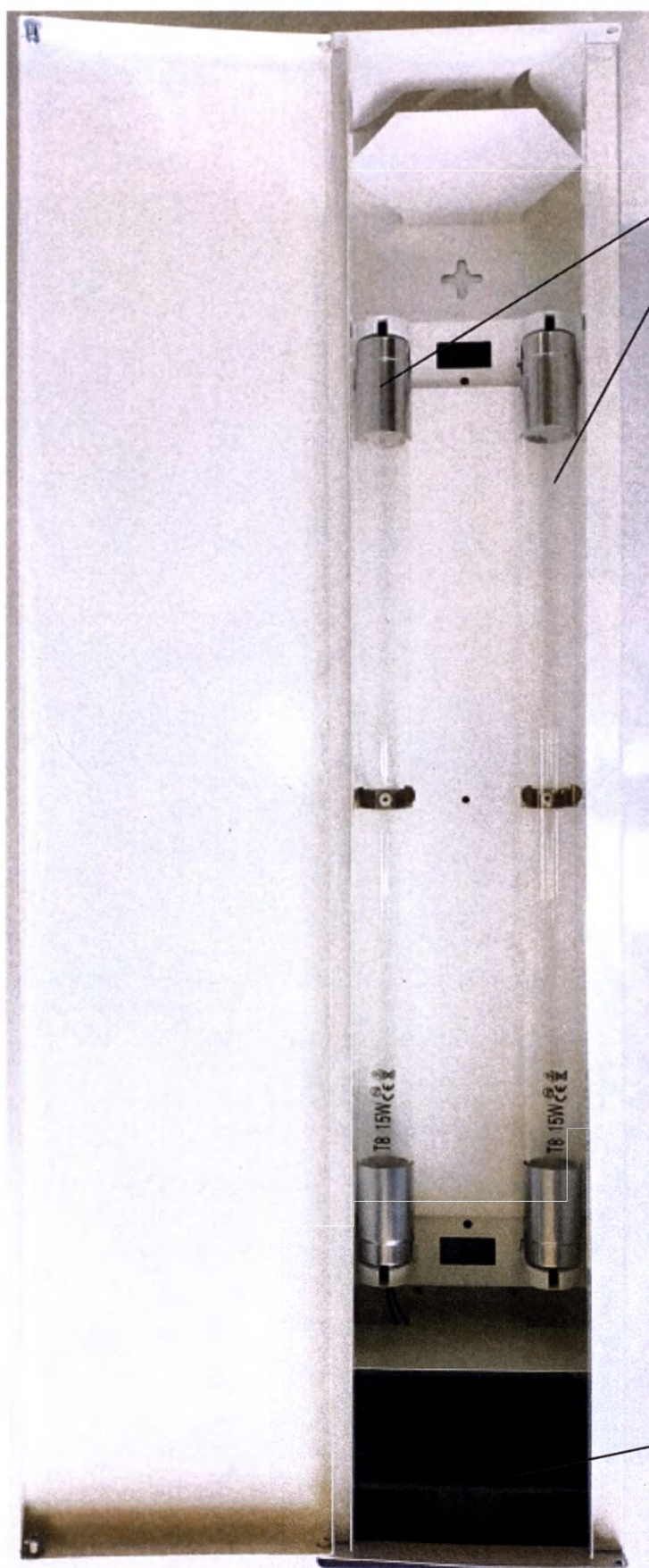
Фото Рециркулятор исполнение «РБУ ПП-02-15» Ультрафиолетовая лампа типа T8 G13 - 2 шт., Вентилятор модель 12025B2HL - 1 шт.
