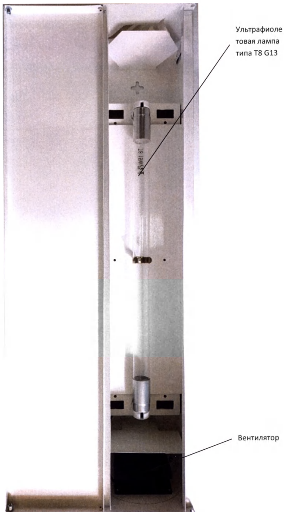
Фото Рециркулятор исполнение «РБУ ПП-01-15» Ультрафиолетовая лампа типа T8 G13 - 1 шт., Вентилятор модель 8038B2HL - 1 шт.
