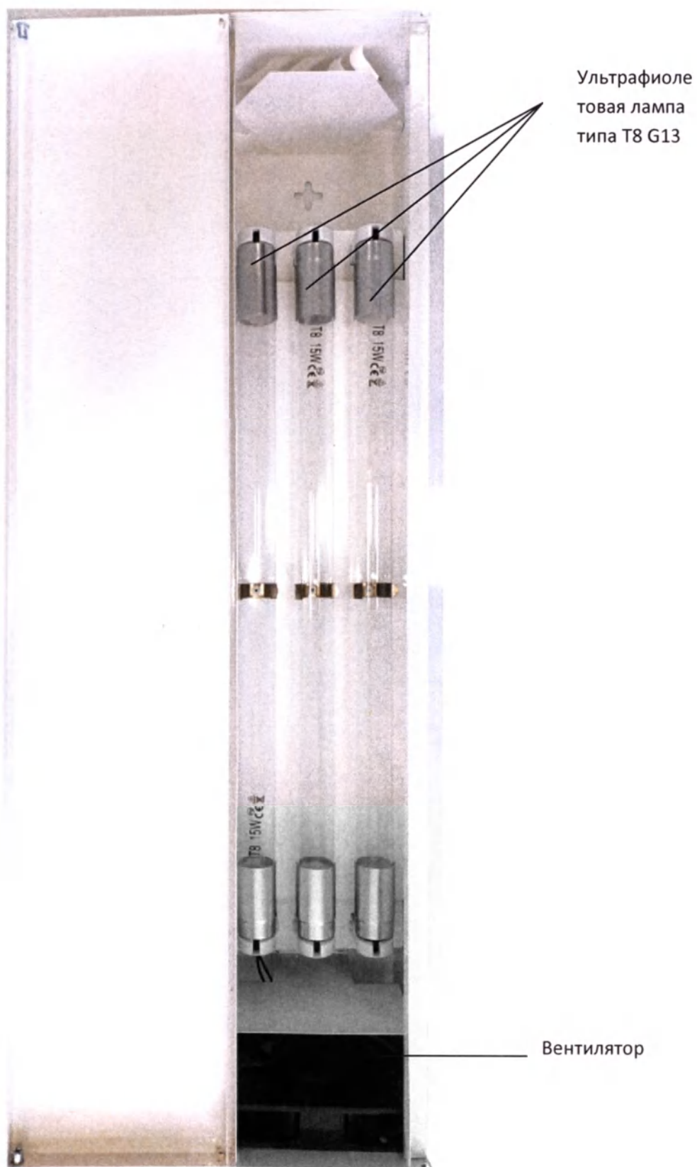
Фото Рециркулятор исполнение «РБУ ПП-03-15» Ультрафиолетовая лампа типа T8 G13 - 3 шт., Вентилятор модель 12025B2HL - 1 шт.
