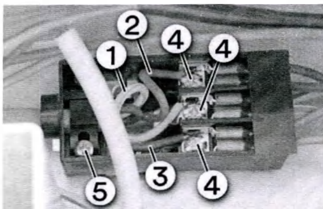
Рис. 14 Внутри сетевой розетки 1) Зелено-желтый провод защитного заземления 2) Коричневый провод 3) Синий провод 4) Винты крепления кабеля 5) Установочный винт для разгрузки натяжения сетевого кабеля
