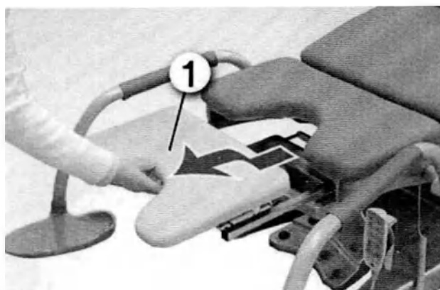
Рис. 83 Выдвижение ножной секции 1) Ножная секция
