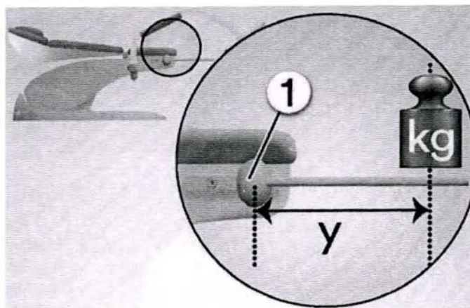
Рис. 2 Определение расстояния y 1) Зажим крепежный (упрощенная схема)
