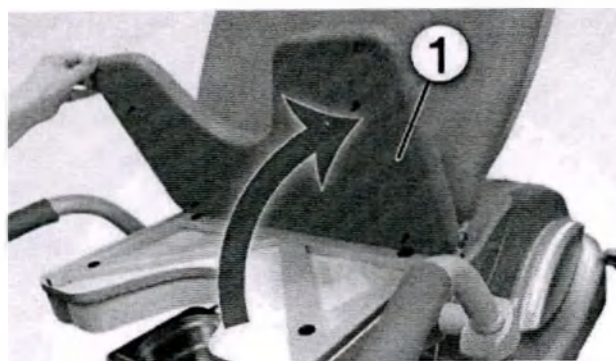
Рис. 49 Снятие старого сиденья 1) Сиденье
