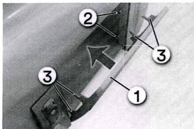
Рис. 21 Установка кожуха розетки 1) Кожух розетки 2) Установочный штифт 3) Фиксирующие зажимы
