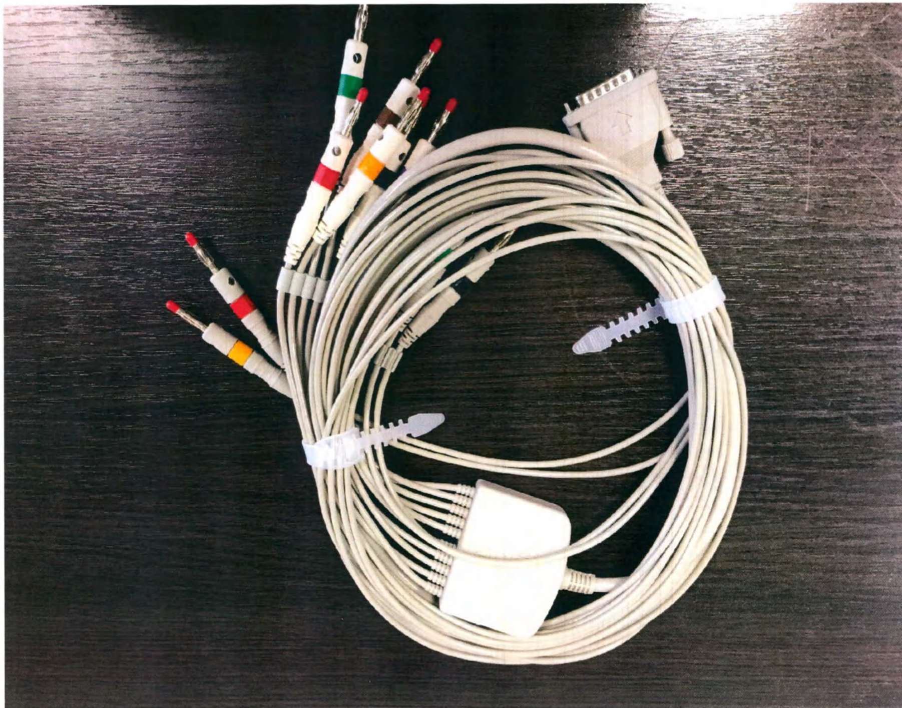
Кабель ЭКГ на 12 отведений тип 3 (общий вид))
