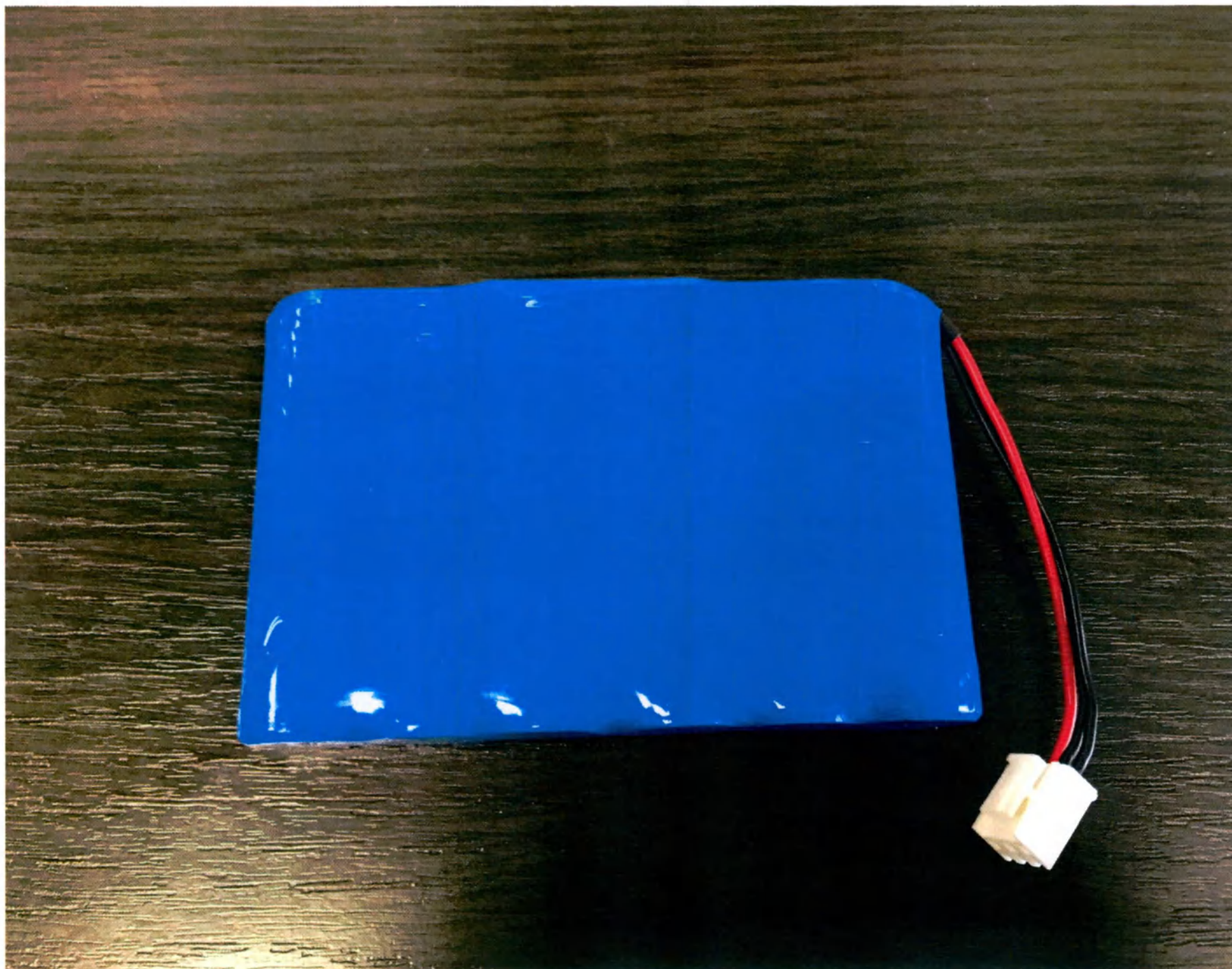
Батарея литиевая для модели CM1200A (общий вид)
