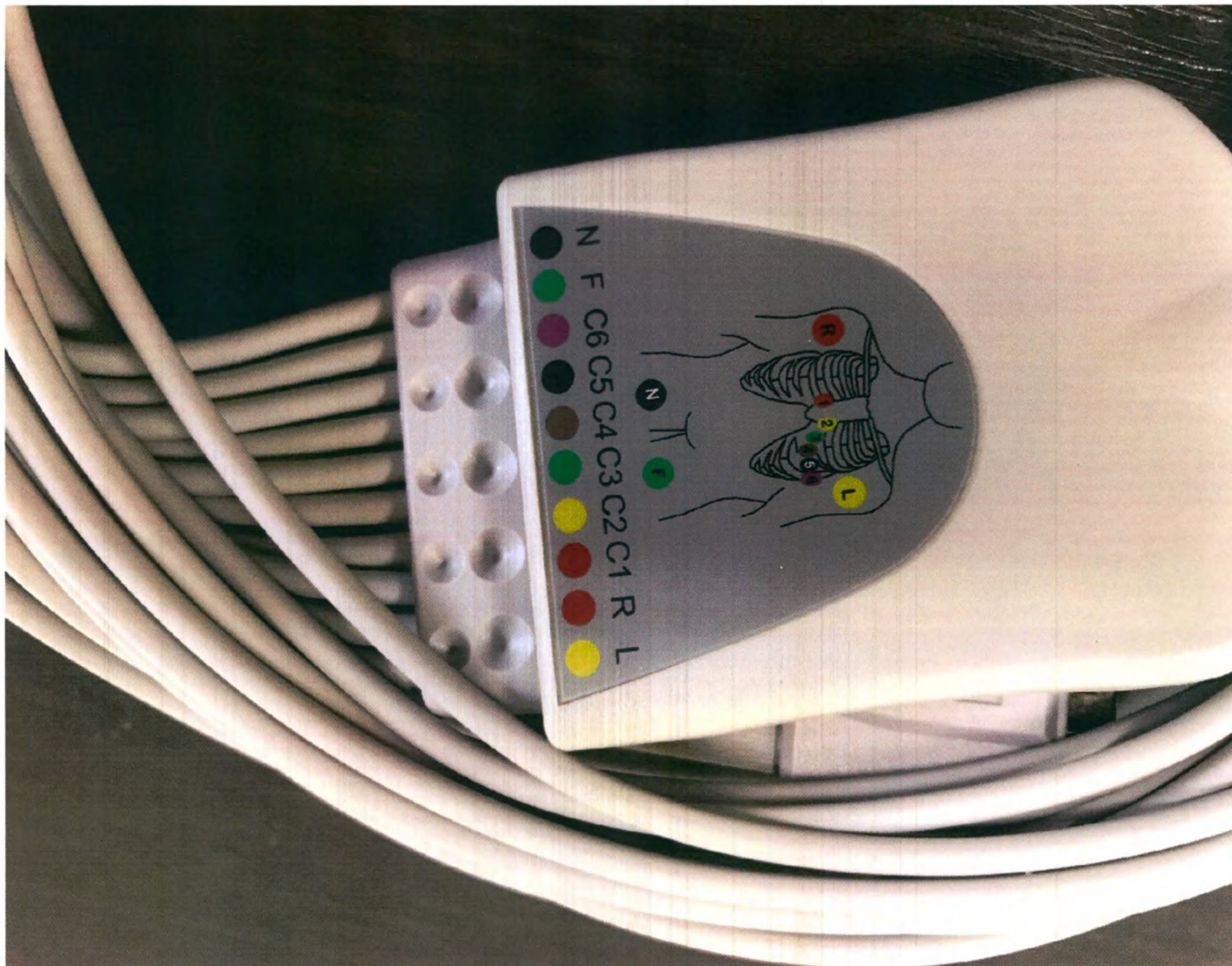
Кабель ЭКГ на 12 отведений тип 1 (разъем отведений)
