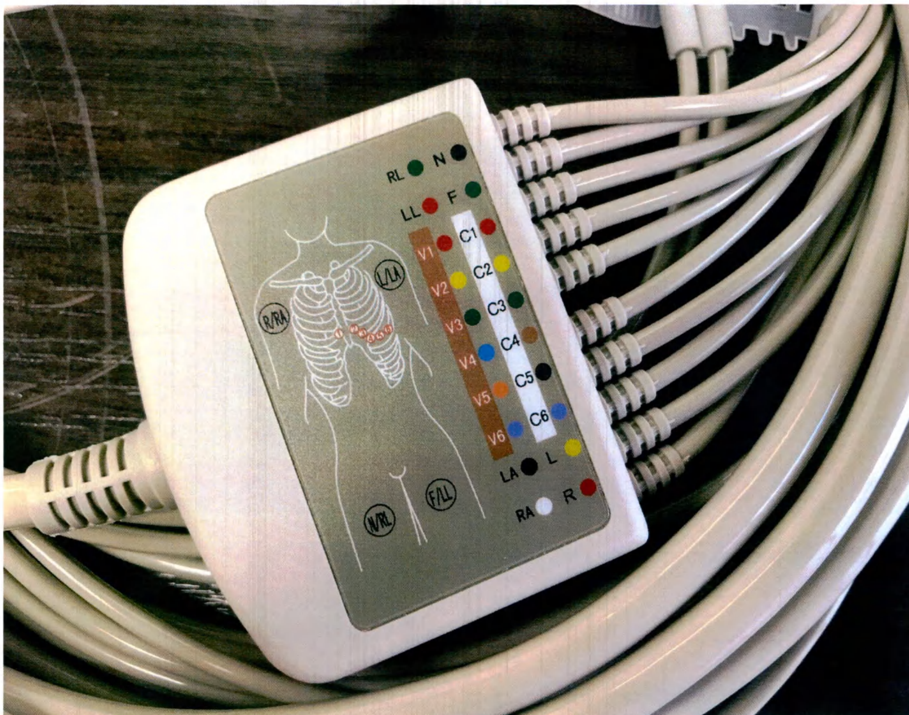
Кабель ЭКГ на 12 отведений тип 3 (разъем отведений)
