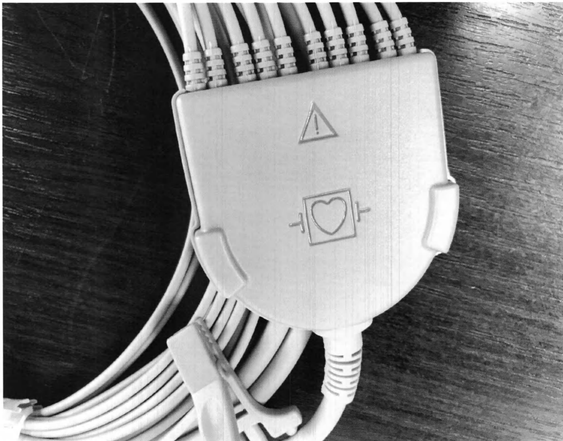
Кабель ЭКГ на 12 отведений тип 4 (маркировка разъема отведений)
