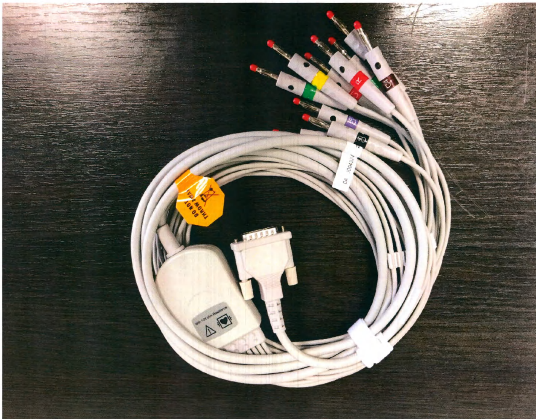
Кабель ЭКГ на 12 отведений тип 2 (общий вид)
