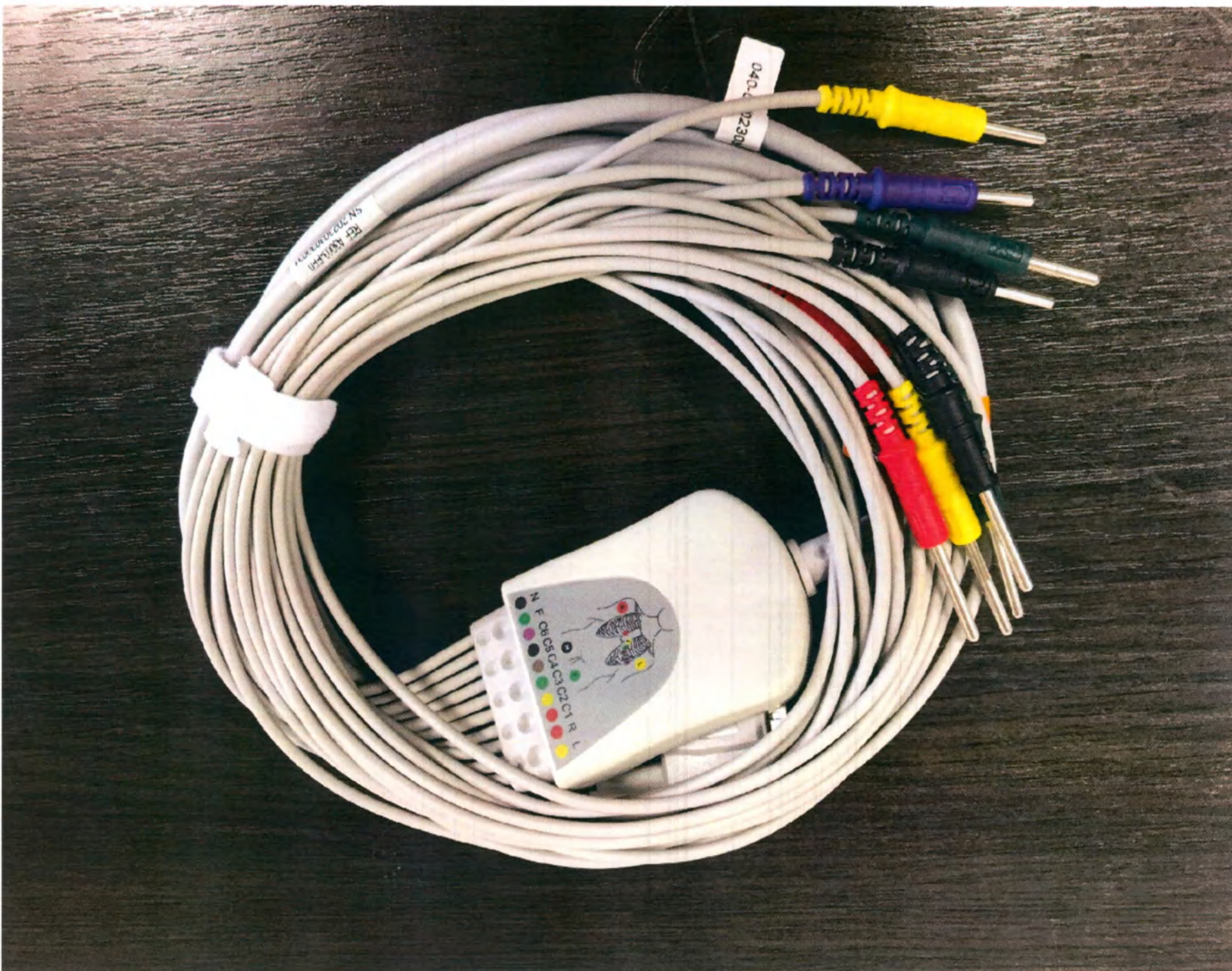
Кабель ЭКГ на 12 отведений тип 1 (общий вид)
