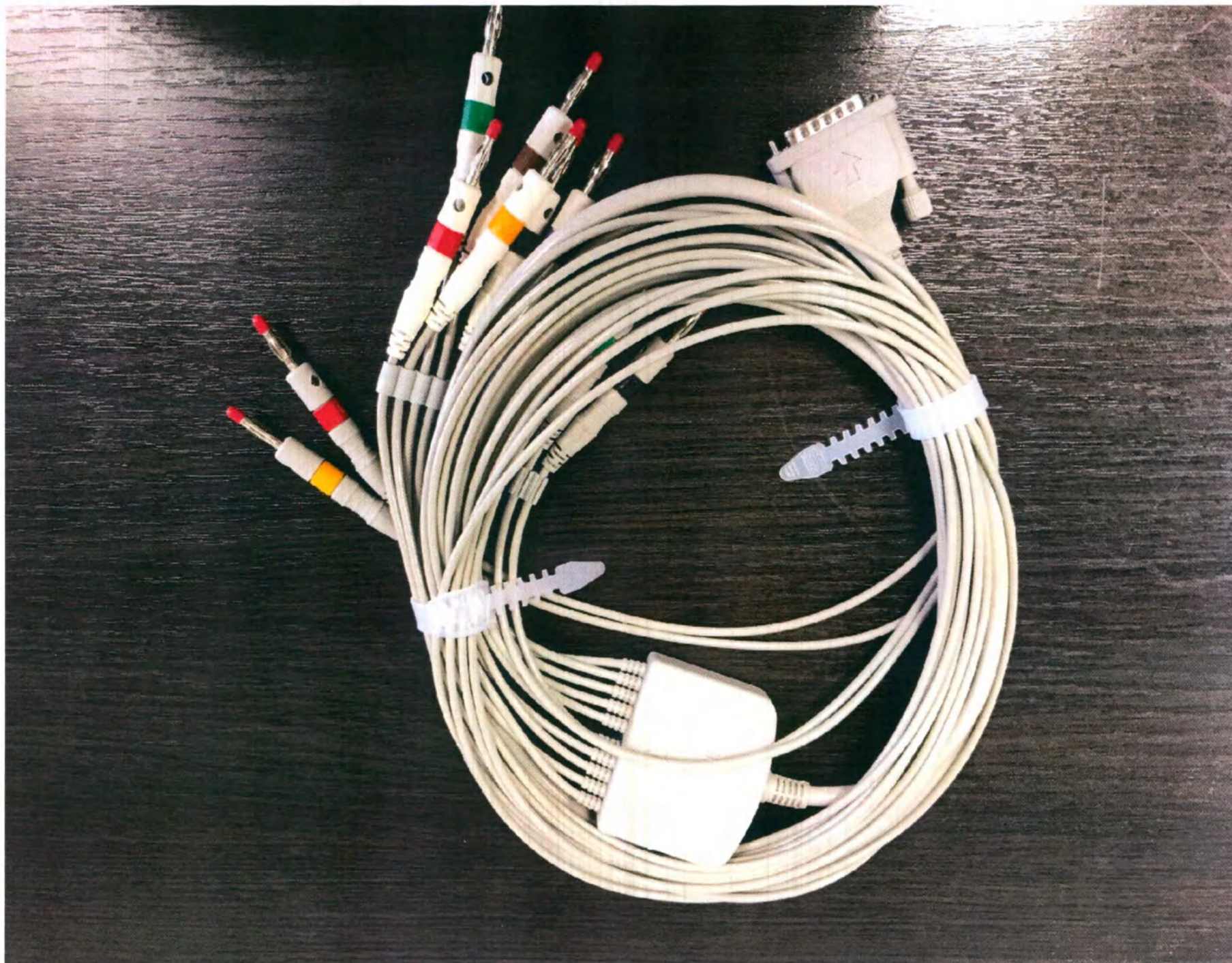
Кабель ЭКГ на 12 отведений тип 4 (общий вид)
