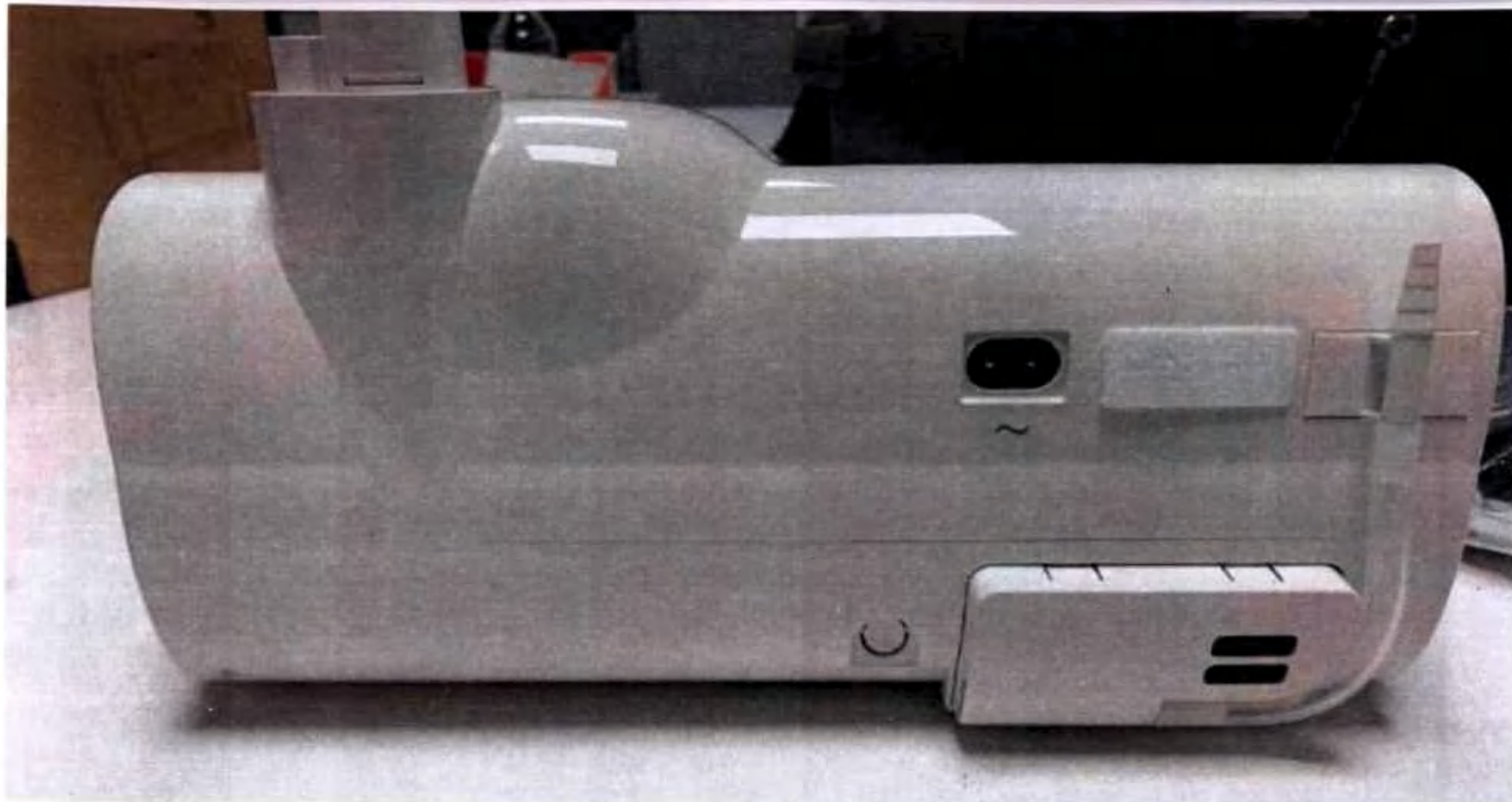
Блок основной HUMID-BM. Вид сзади
