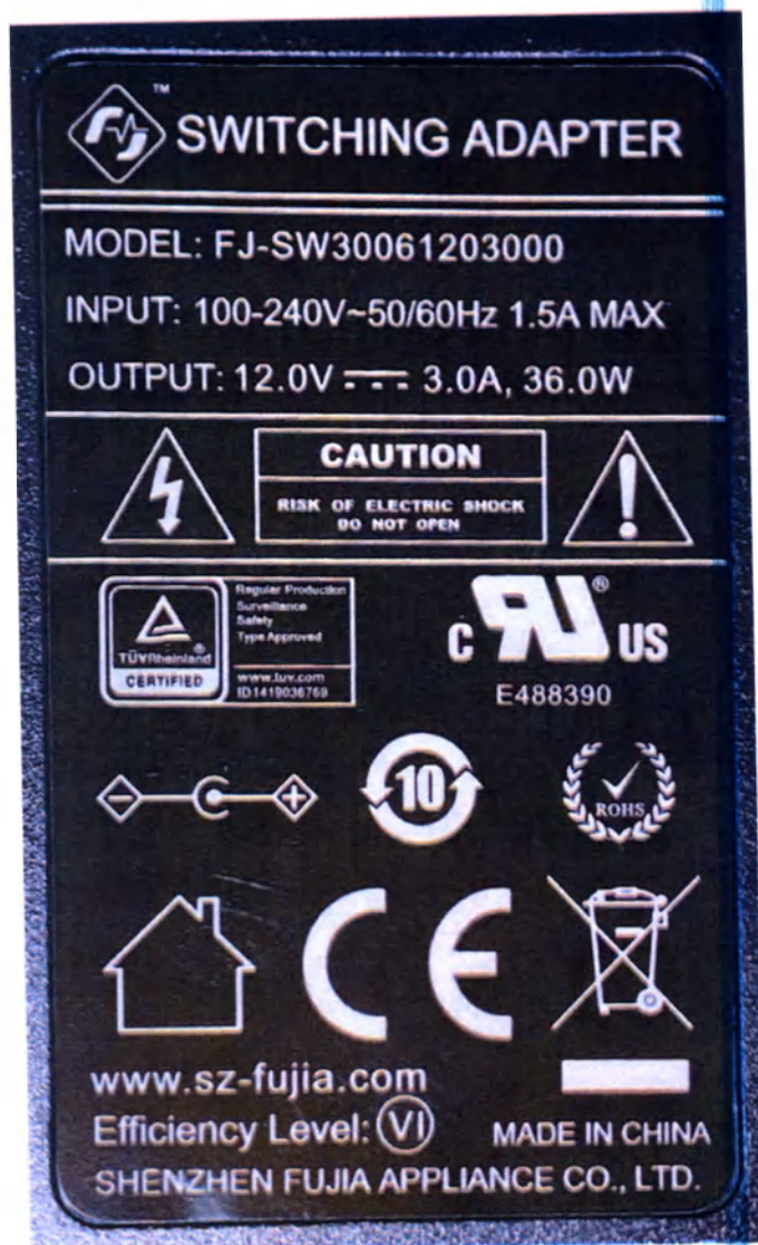
Фото 30. Оригинальная маркировка производителя на блоке питания видеопроцессора.
