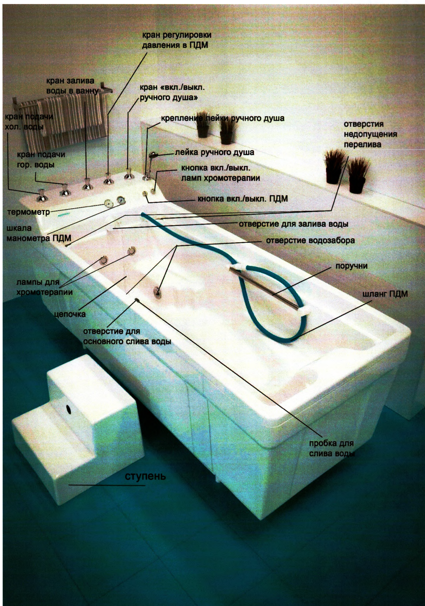
Фото 1 – Общий вид. Исполнение №1.
