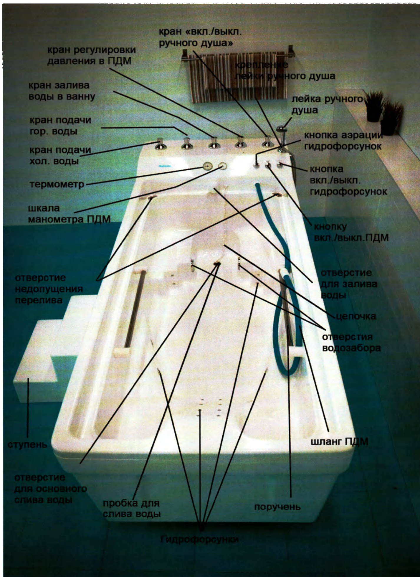
Фото 3 – Общий вид. Исполнение №2. («Ванна водолечебная «Гольфстрим», модификация – гидромассажная, с ПДМ): ПДМ/Г16
