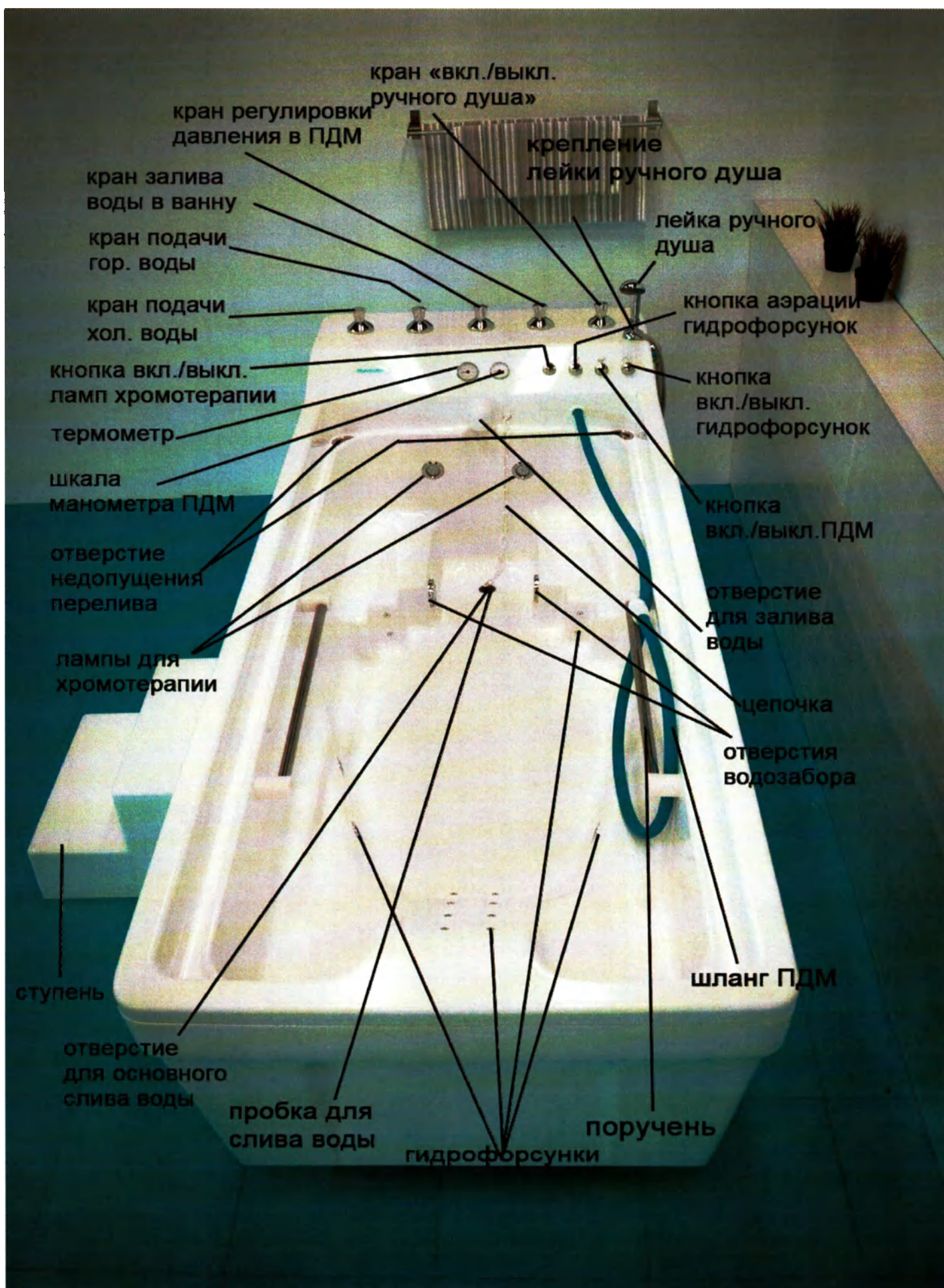
Фото 5 – Общий вид. Исполнение №3. («Ванна водолечебная «Гольфстрим», модификация – гидромассажная, с ПДМ, с хромолампами): ПДМ/Г16/Х
