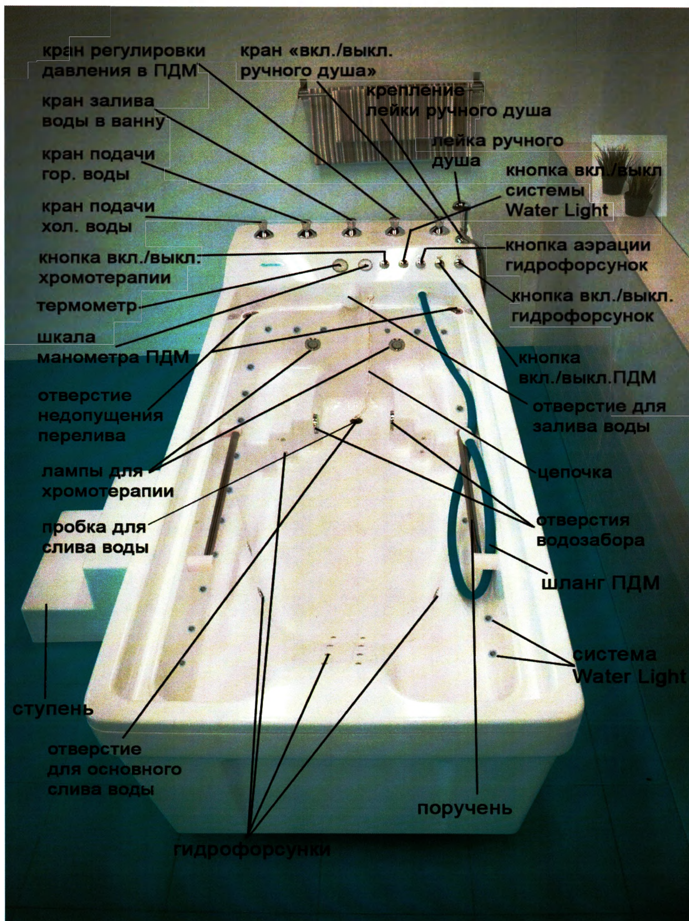
Фото 25 – Общий вид. Исполнение №13.
