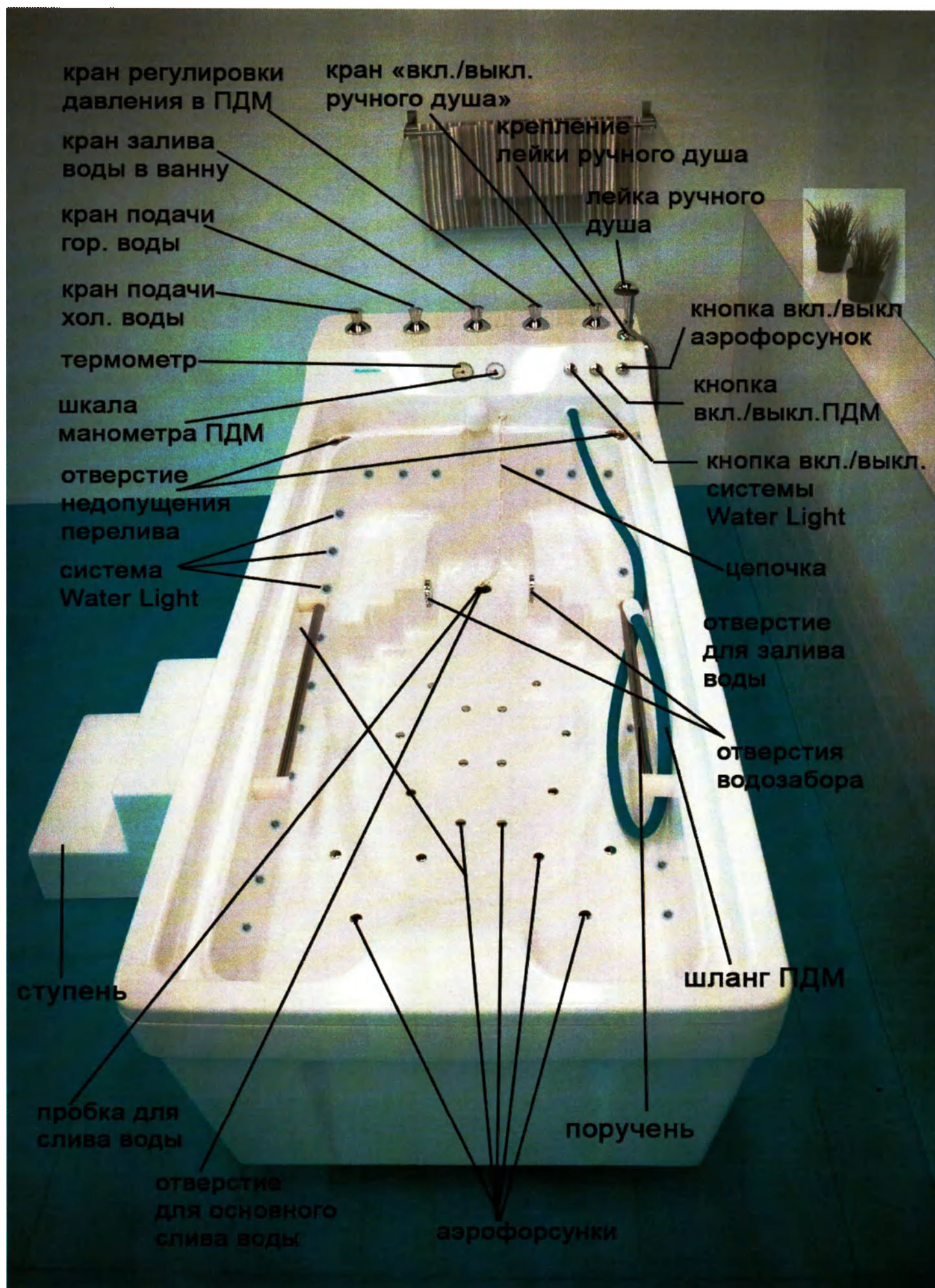
Фото 15 – Общий вид. Исполнение №8. («Ванна водолечебная «Гольфстрим», модификация – аромассажная, с ПДМ, с системой Water Light): ПДМ/A18/C
