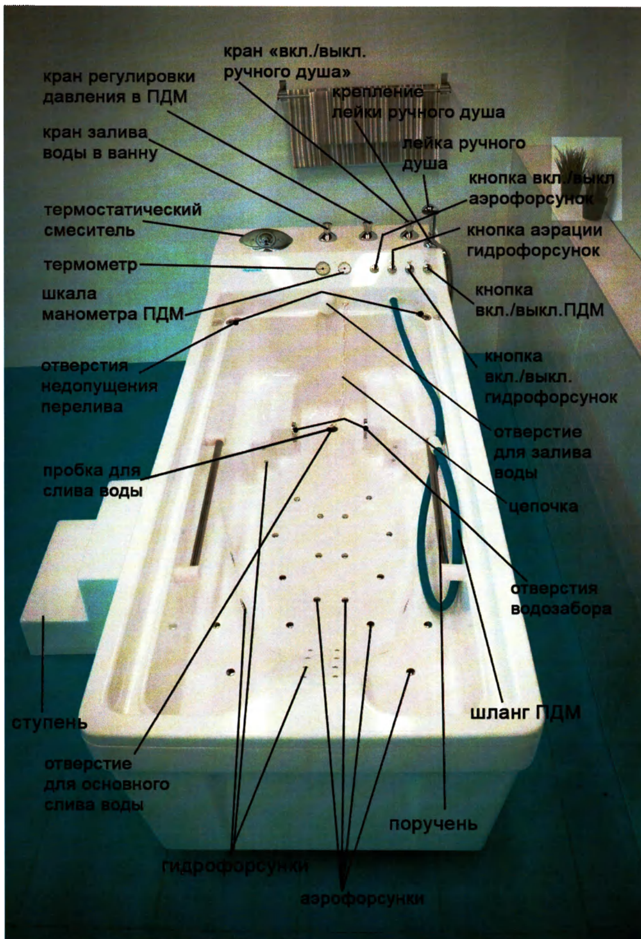
Фото 23 – Общий вид. Исполнение №12. («Ванна водолечебная «Гольфстрим», модификация – гидро/аэромассажная, с ПДМ, с термостатом): ПДМ/Г16/А18/Т
