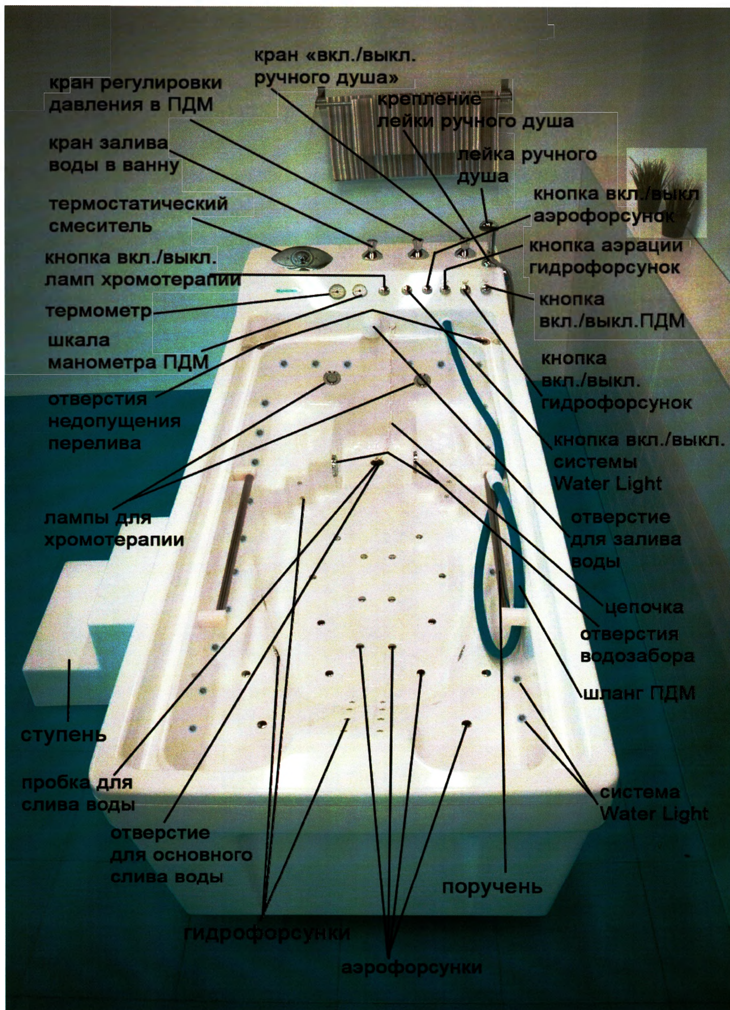
Фото 21 – Общий вид. Исполнение №11.
