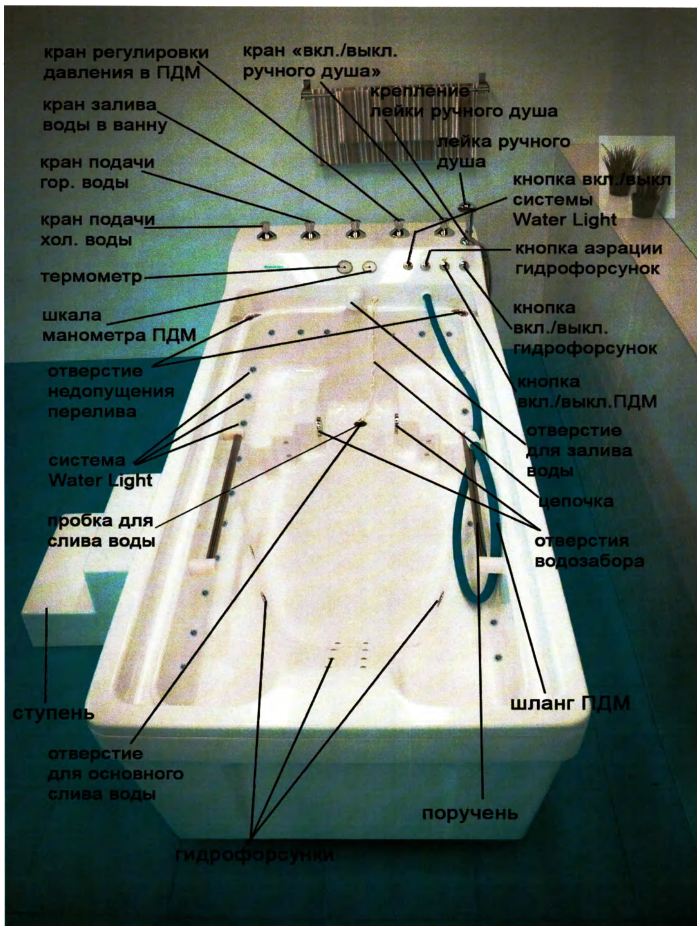
Фото 27 – Общий вид. Исполнение №14. («Ванна водолечебная «Гольфстрим», модификация - гидромассажная, с ПДМ, с системой Water Light): ПДМ/Г16/С
