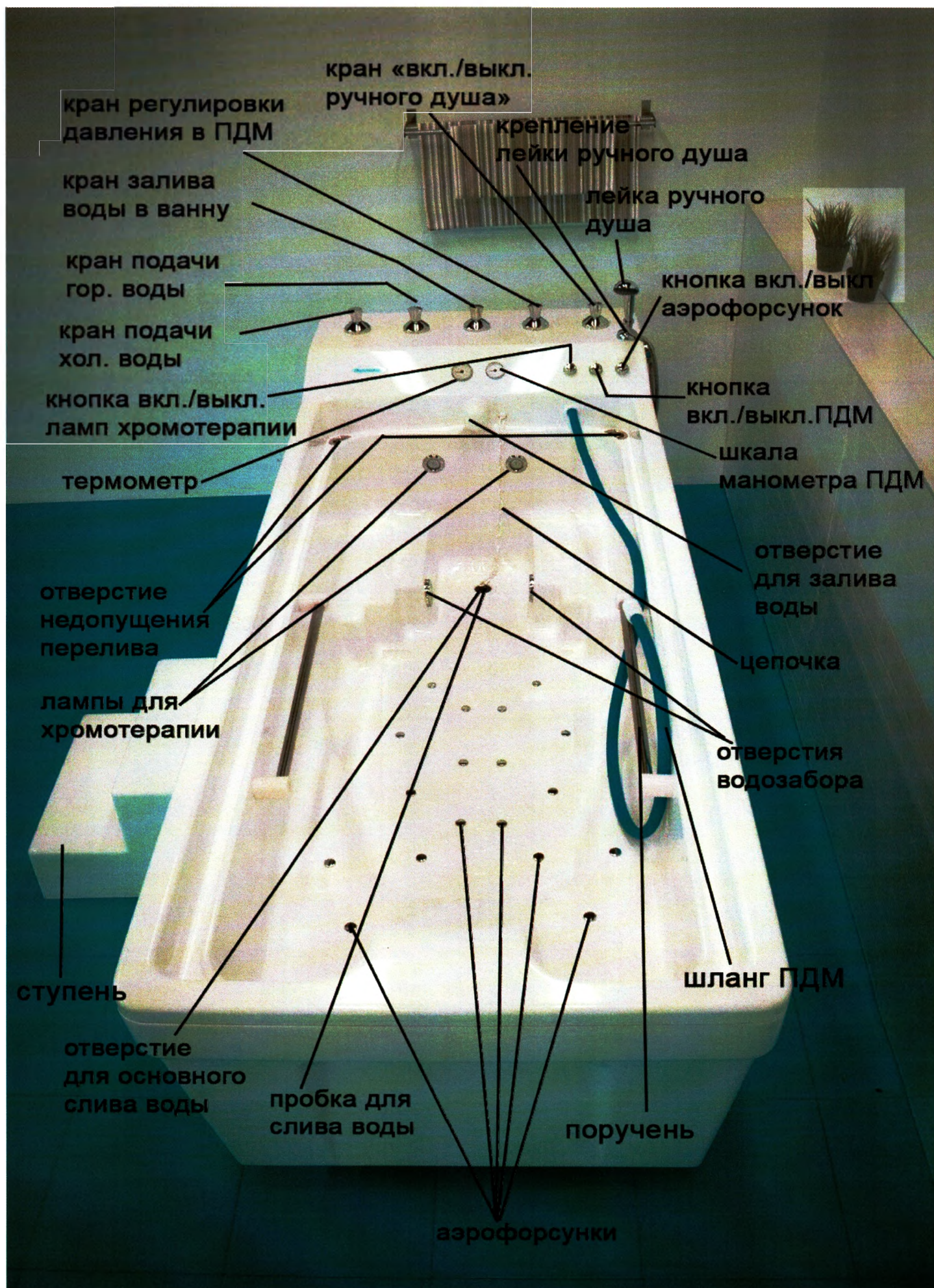
Фото 13 – Общий вид. Исполнение №7. («Ванна водолечебная «Гольфстрим», модификация – аэромассажная, с ПДМ, с хромолампами): ПДМ/А18/Х
