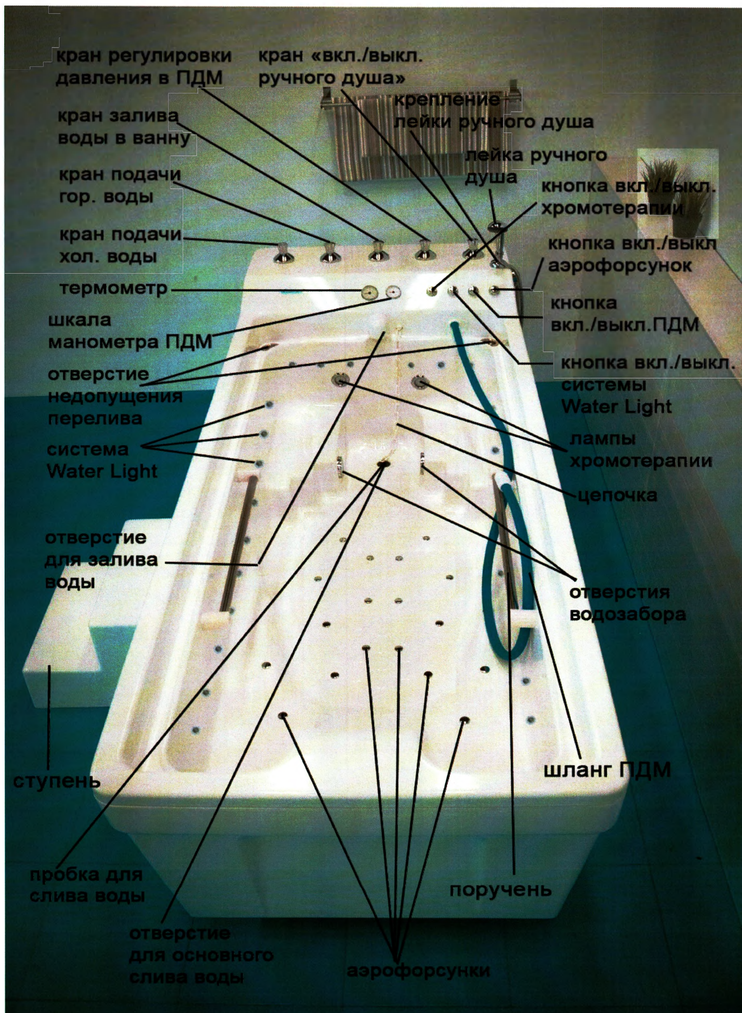
Фото 17 – Общий вид. Исполнение №9.
