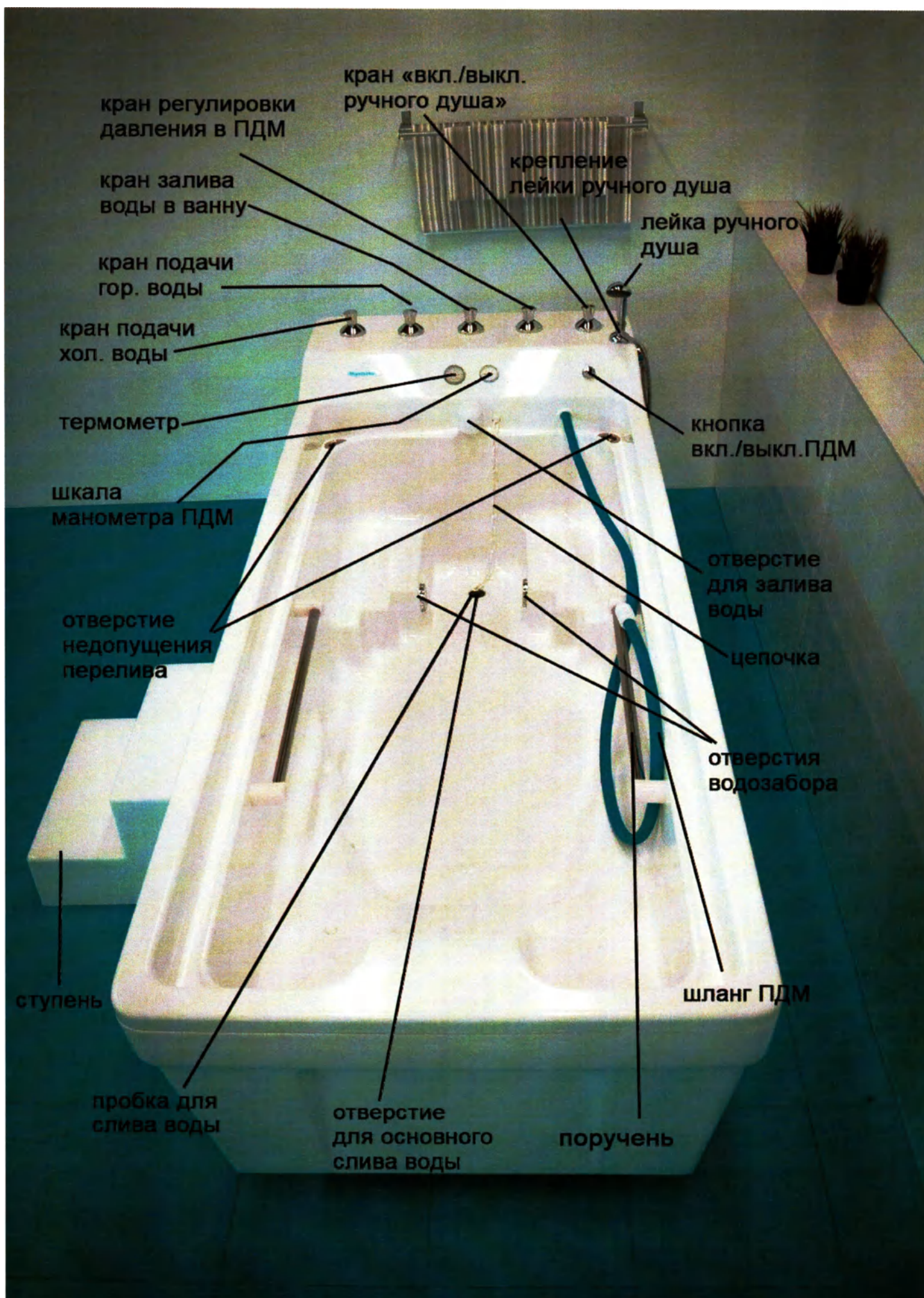
Фото 19 – Общий вид. Исполнение №10. («Ванна водолечебная «Гольфстрим», модификация – с ПДМ):ПДМ
