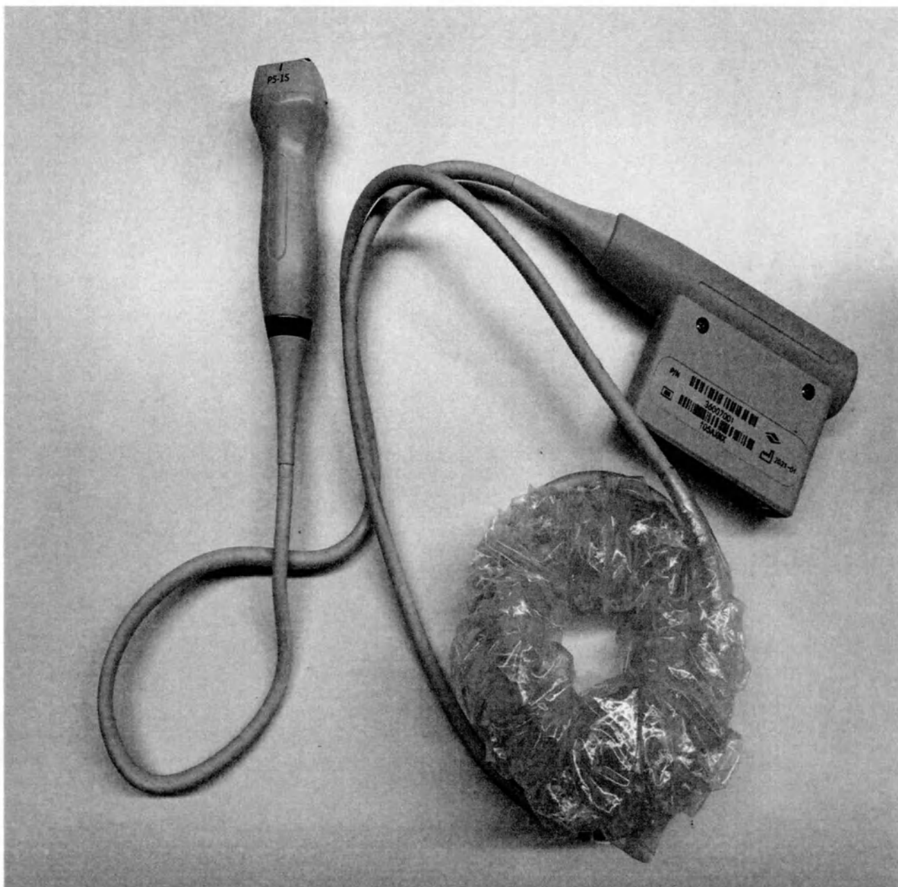
Датчик P5-1S
