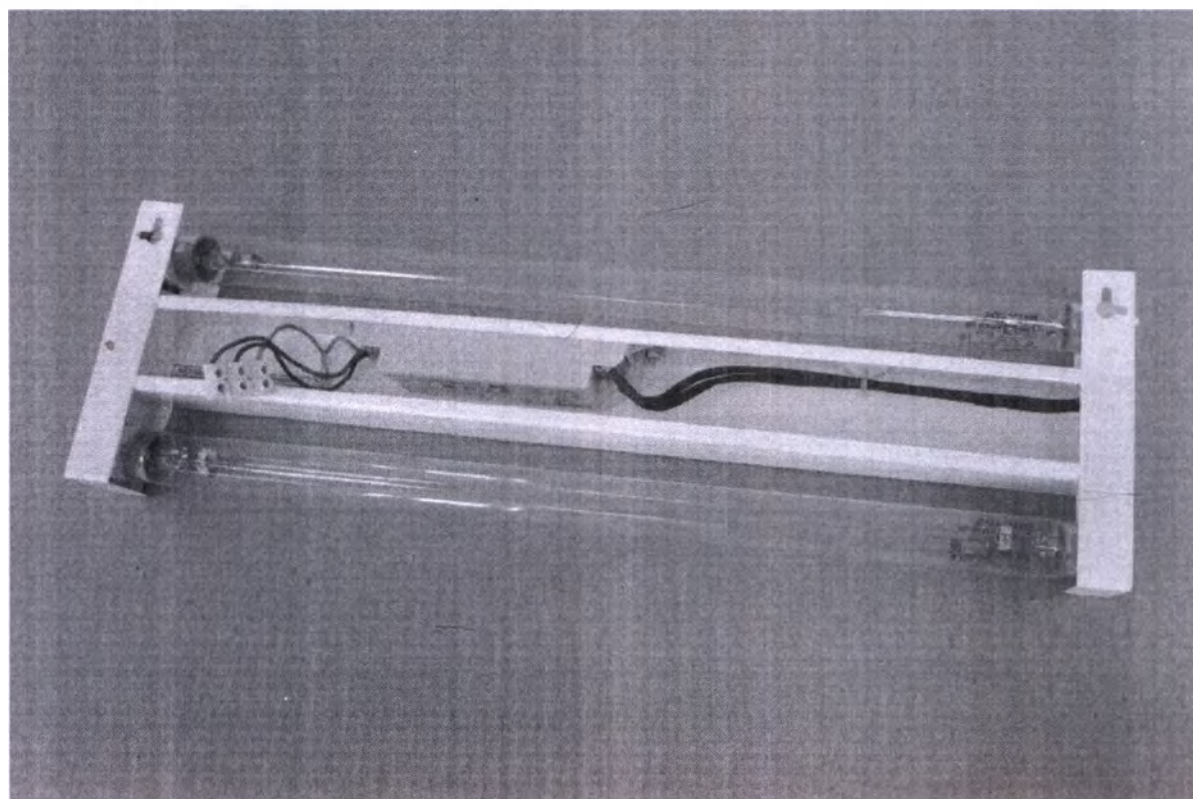
Фотография 6. Облучатель УФ-бактерицидный ОБН-70-«СПДС». Вид сзади.
