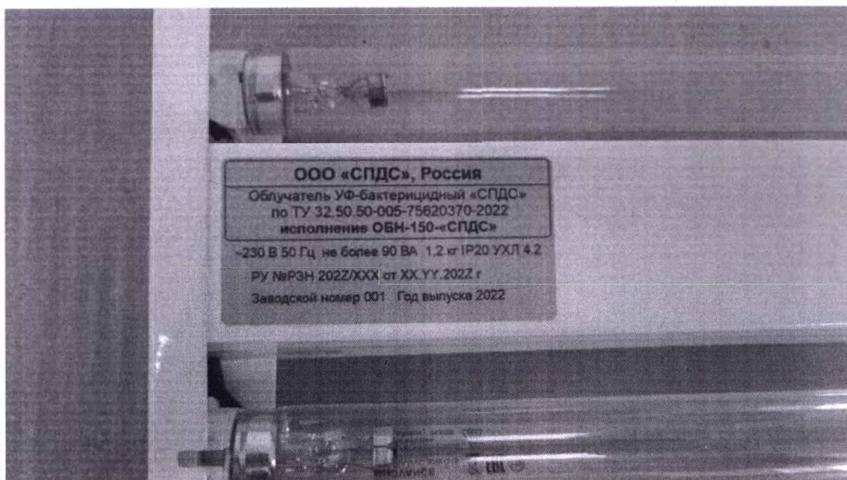
Фотография 19. Облучатель УФ-бактерицидный ОБН-150-«СПДС». Маркировка облучателя
