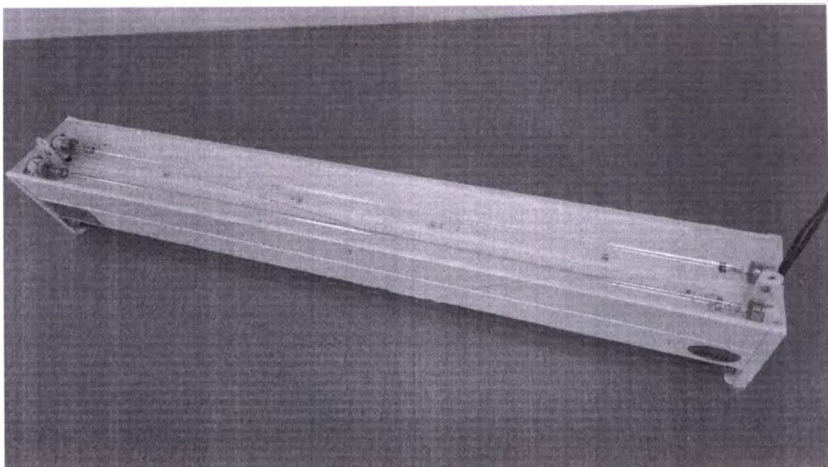
Фотография 42. Облучатель УФ-бактерицидный ОБК-300-«СПДС». Вид сверху.
