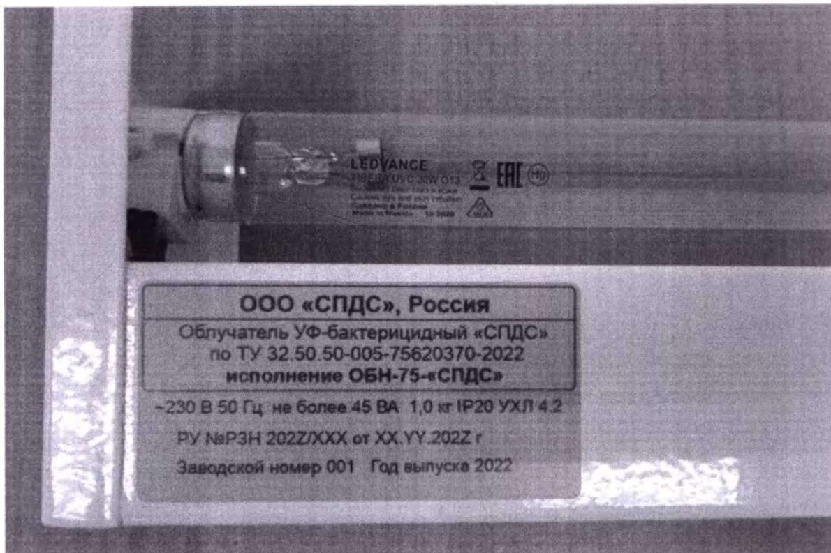
Фотография 11. Облучатель УФ-бактерицидный ОБН-75-«СПДС». Маркировка облучателя.
