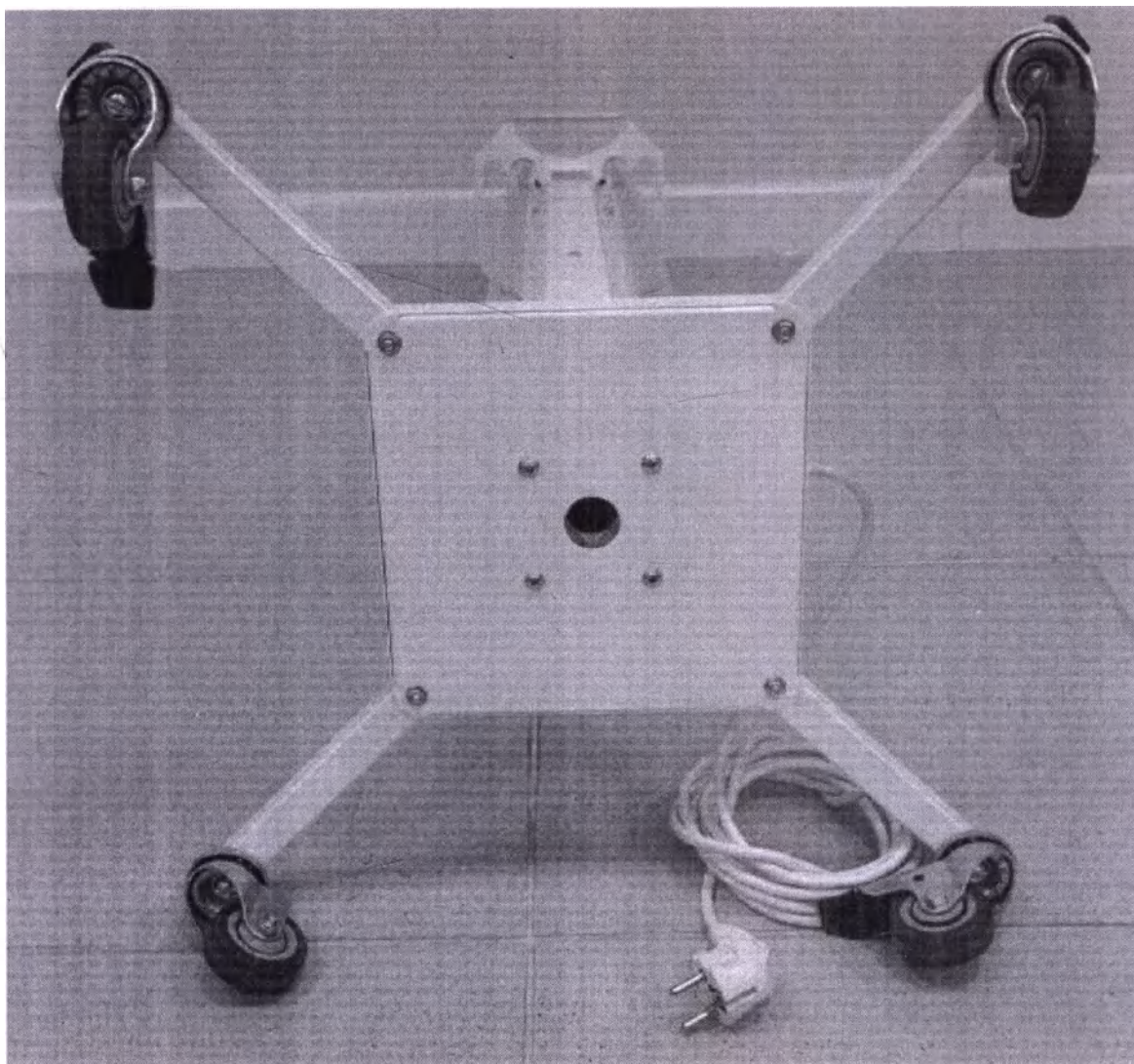
Фотография 73. Облучатель УФ-бактерицидный ОБПп-300-«СПДС». Вид снизу.
