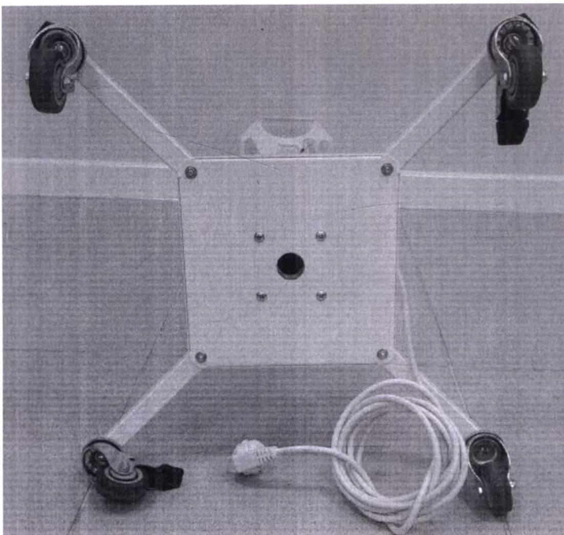
Фотография 58. Облучатель УФ-бактерицидный ОБП-225-«СПДС». Вид снизу.
