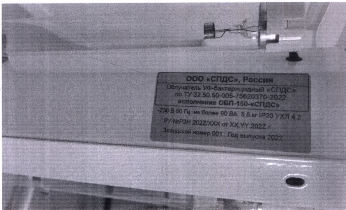
Фотография 50. Облучатель УФ-бактерицидный ОБП-150-«СПДС». Маркировка облучателя.
