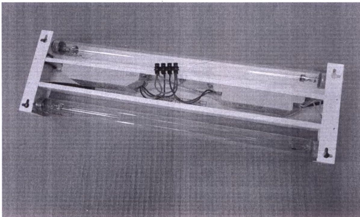
Фотография 31. Облучатель УФ-бактерицидный ОБК-90-«СПДС». Вид сзади.
