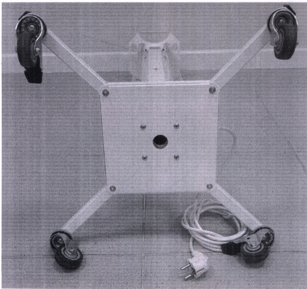
Фотография 68. Облучатель УФ-бактерицидный ОБП-300-«СПДС». Вид снизу.
