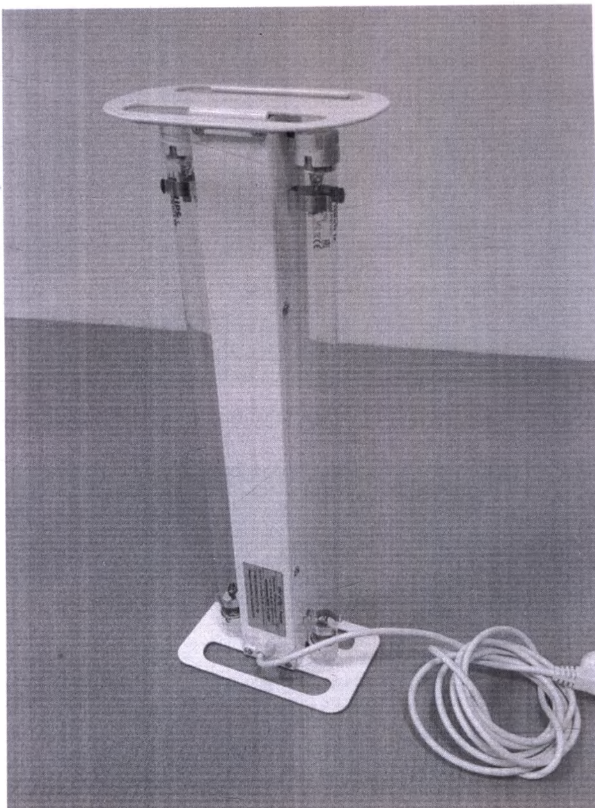
Фотография 89. Облучатель УФ-бактерицидный ОБПН-70-«СПДС». Вид сзади.
