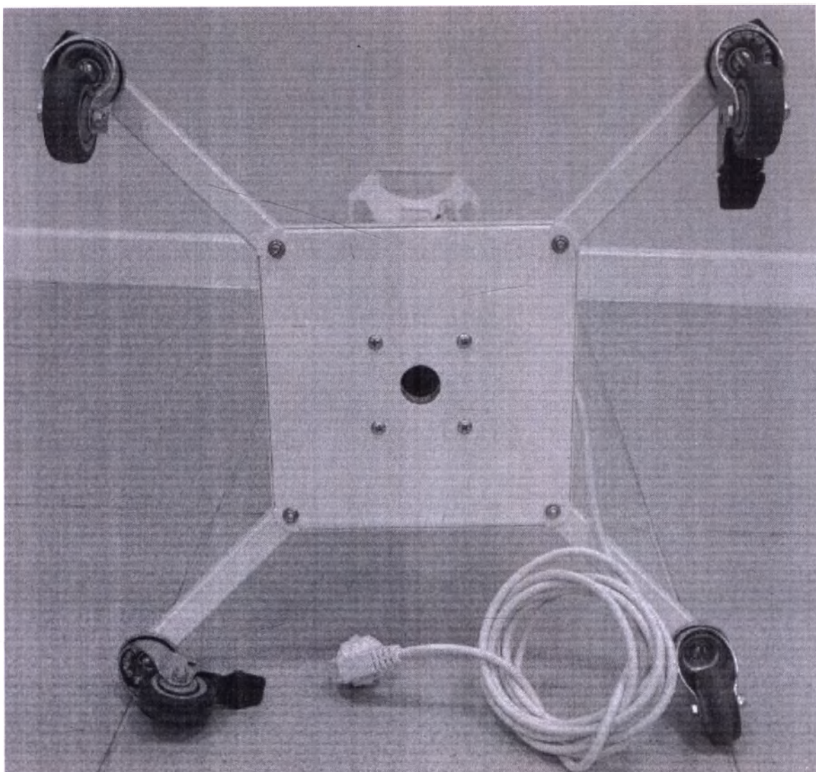
Фотография 63. Облучатель УФ-бактерицидный ОБП-225-«СПДС». Вид снизу.
