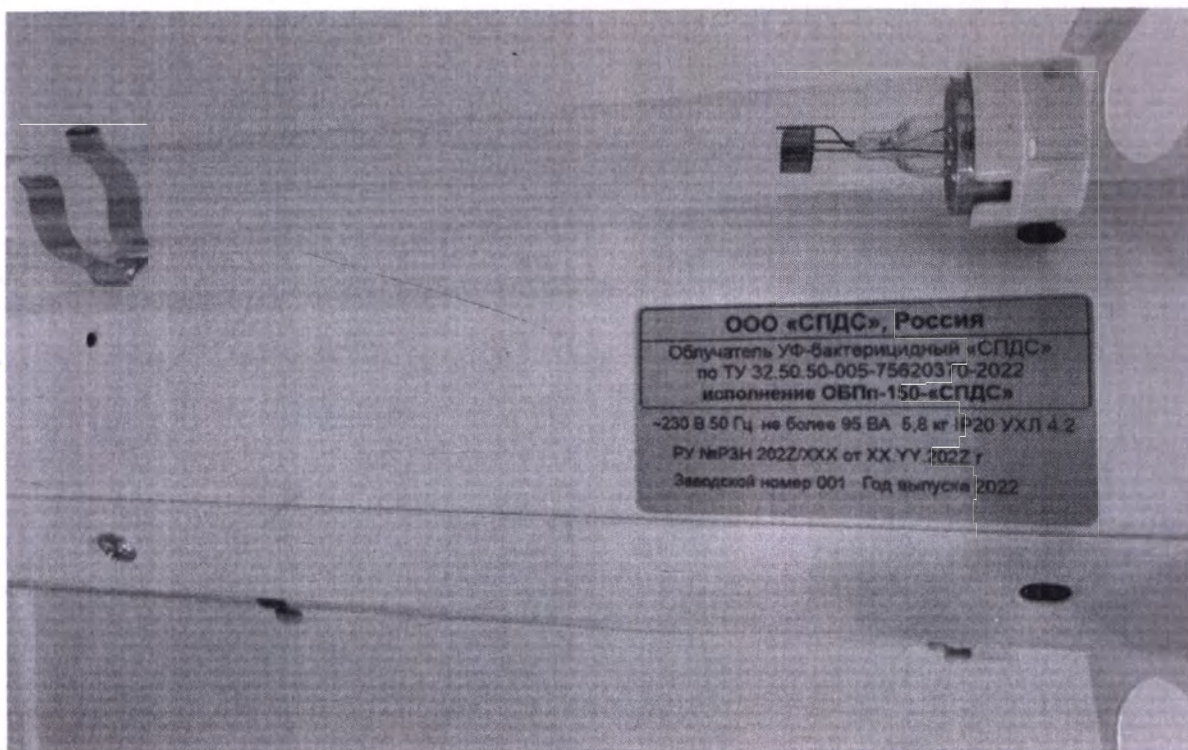
Фотография 55. Облучатель УФ-бактерицидный ОБП-150-«СПДС». Маркировка облучателя.
