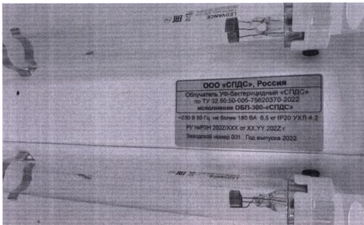
Фотография 70. Облучатель УФ-бактерицидный ОБП-300-«СПДС». Маркировка облучателя.
