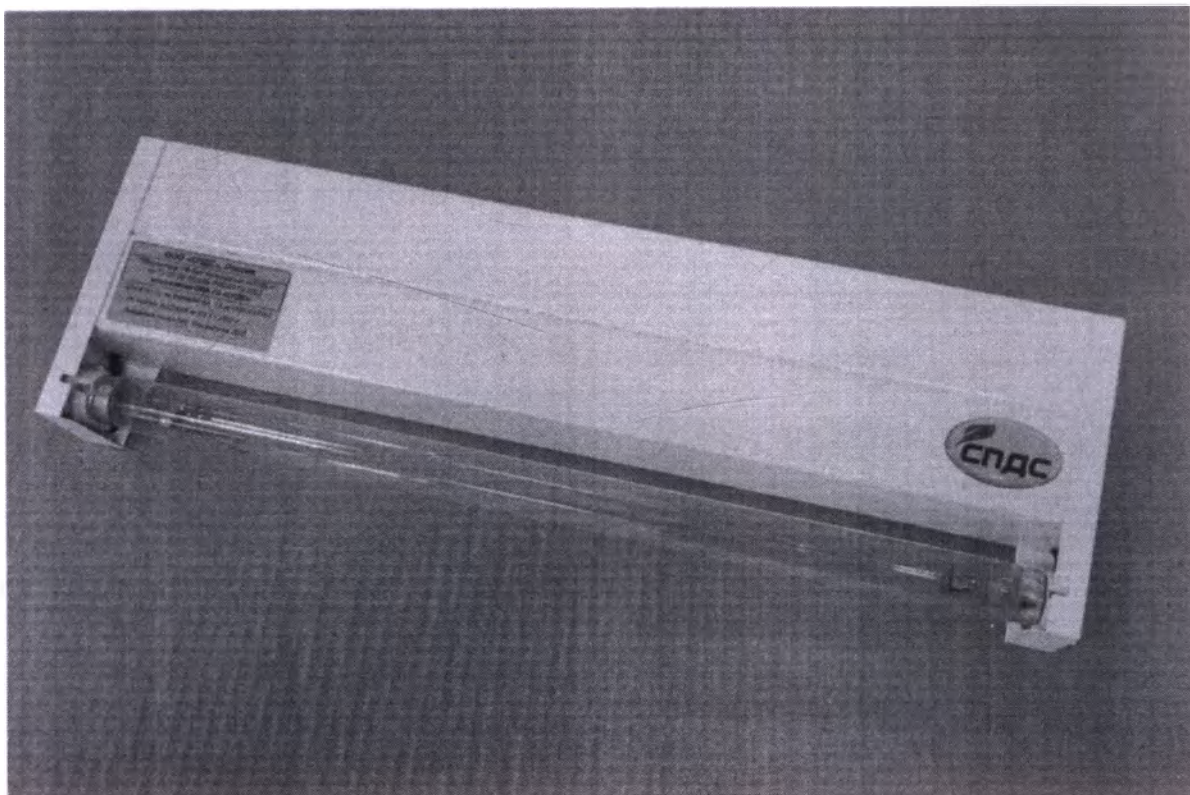
Фотография 26. Облучатель УФ-бактерицидный ОБК-70-«СПДС». Вид спереди.
