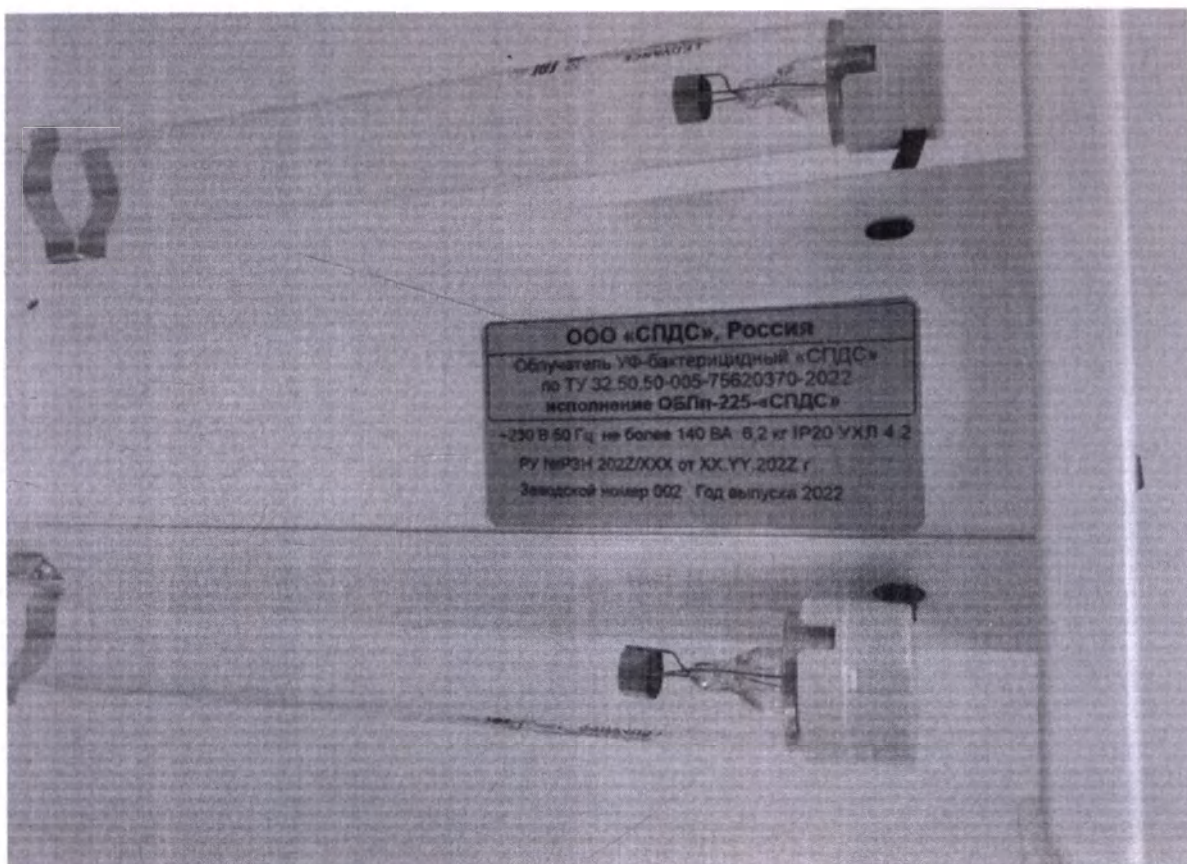
Фотография 65. Облучатель УФ-бактерицидный ОБП-225-«СПДС». Маркировка облучателя.
