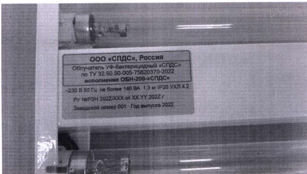
Фотография 23. Облучатель УФ-бактерицидный ОБН-200-«СПДС». Маркировка облучателя
