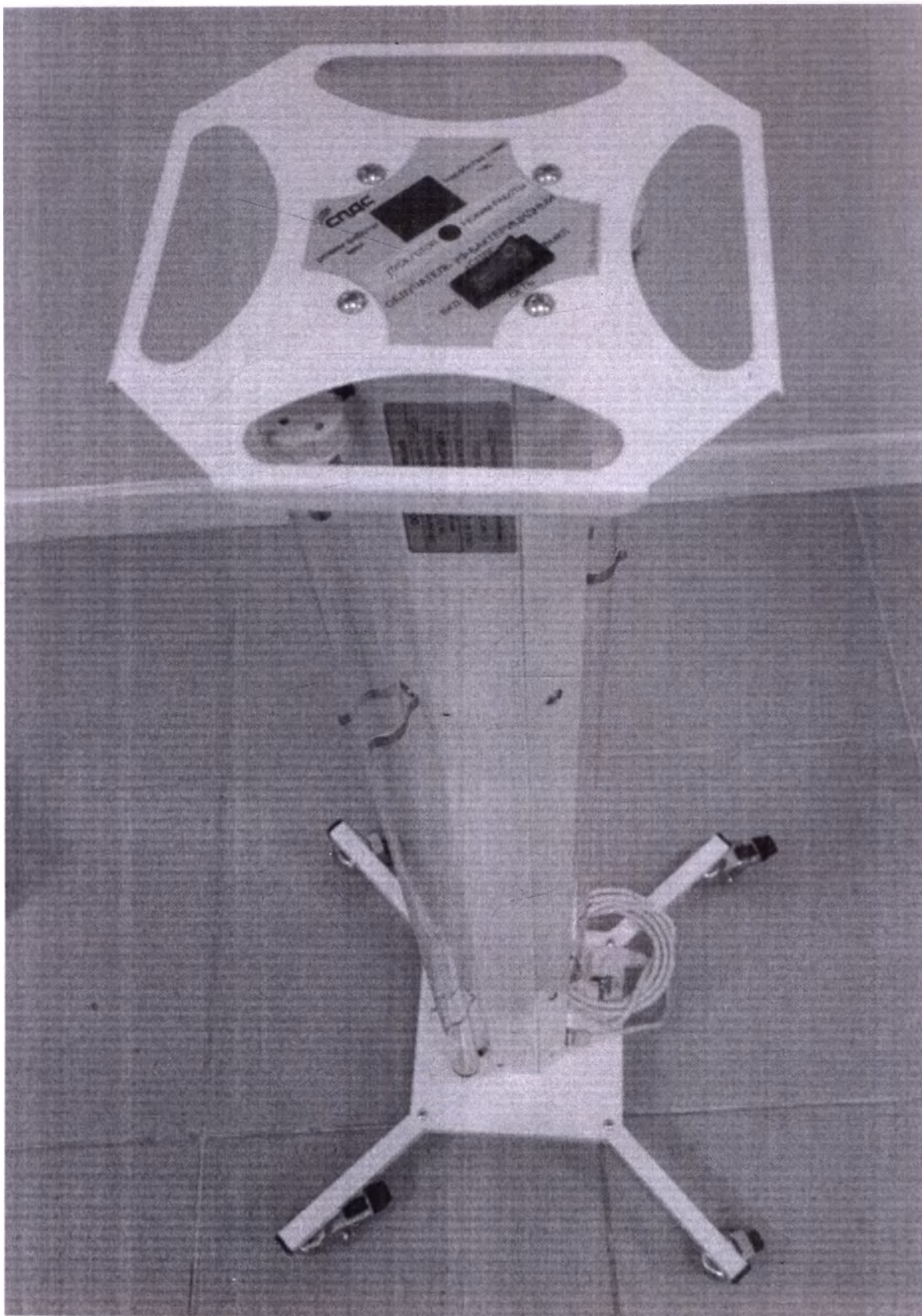
Фотография 62. Облучатель УФ-бактерицидный ОБПп-225-«СПДС». Вид сверху.
