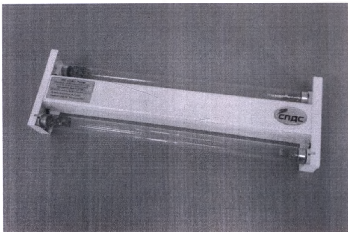
Фотография 5. Облучатель УФ-бактерицидный ОБН-70-«СПДС». Вид спереди.
