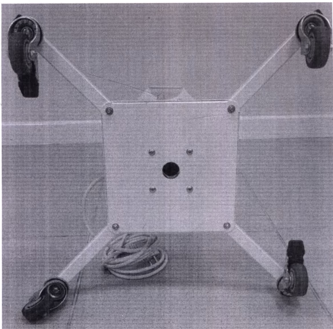
Фотография 78. Облучатель УФ-бактерицидный ОБПп-300-«СПДС». Вид снизу.
