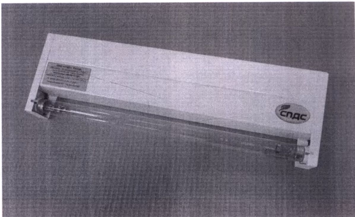
Фотография 30. Облучатель УФ-бактерицидный ОБК-90-«СПДС». Вид спереди.
