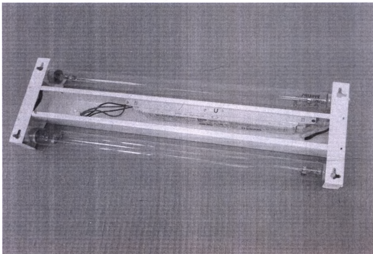
Фотография 14. Облучатель УФ-бактерицидный ОБН-90-«СПДС». Вид сзади.
