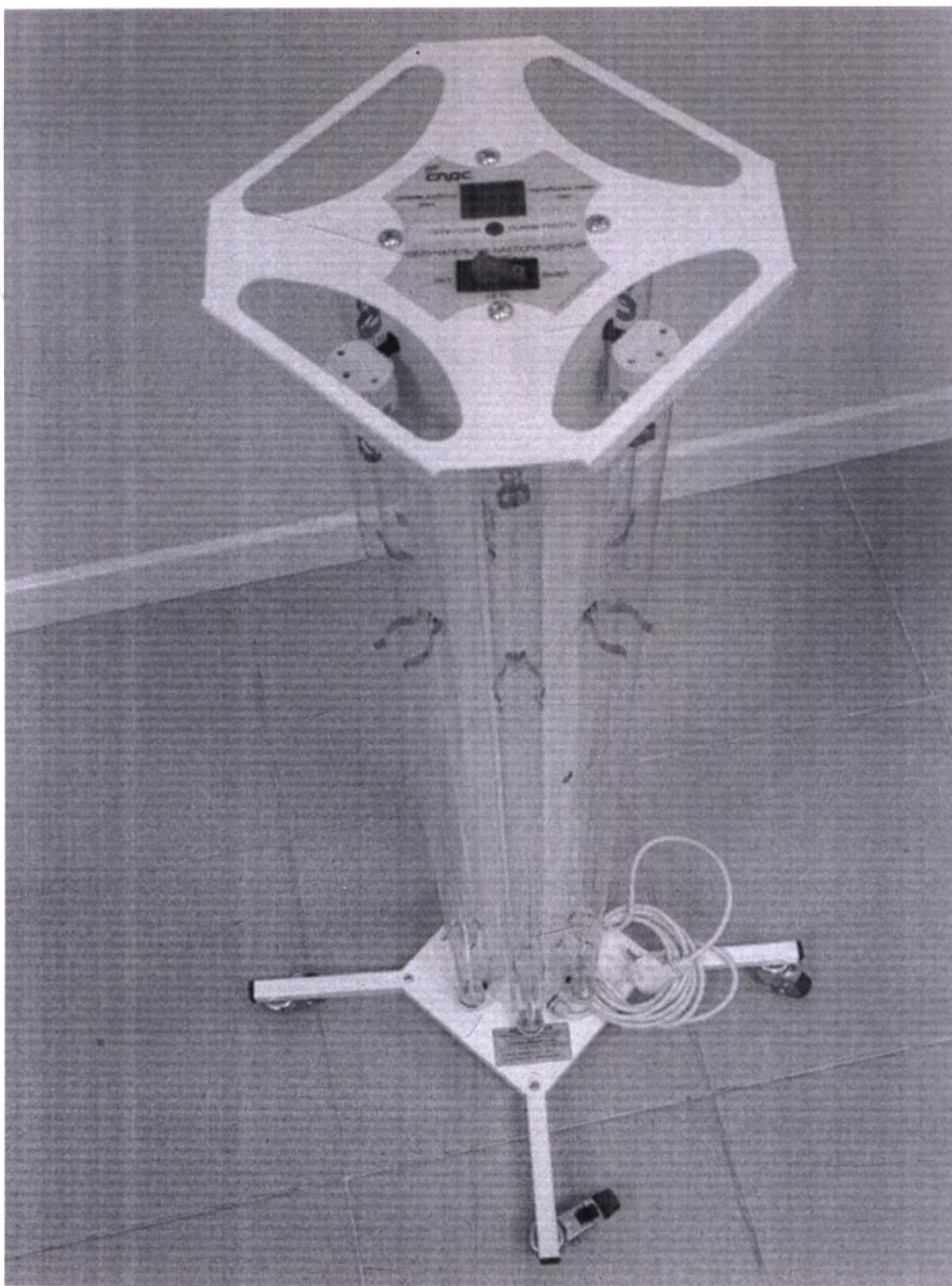
Фотография 82. Облучатель УФ-бактерицидный ОБП-450-«СПДС». Вид сверху.
