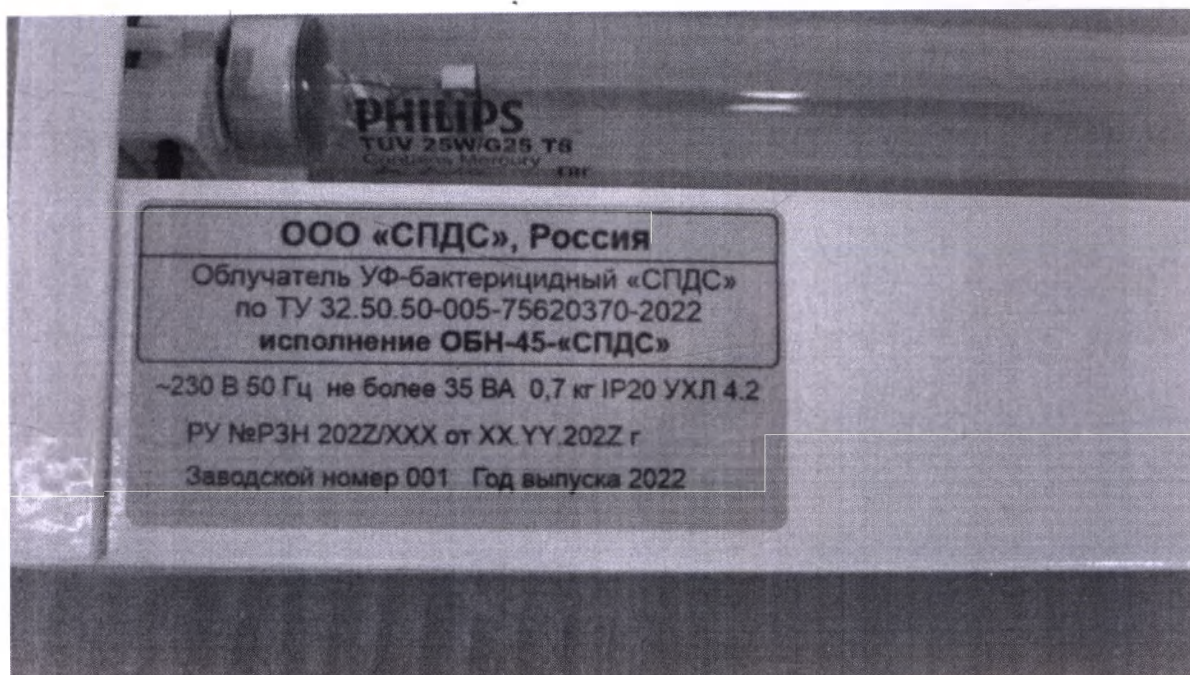
Фотография 3. Облучатель УФ-бактерицидный ОБН-45-«СПДС». Маркировка облучателя.
