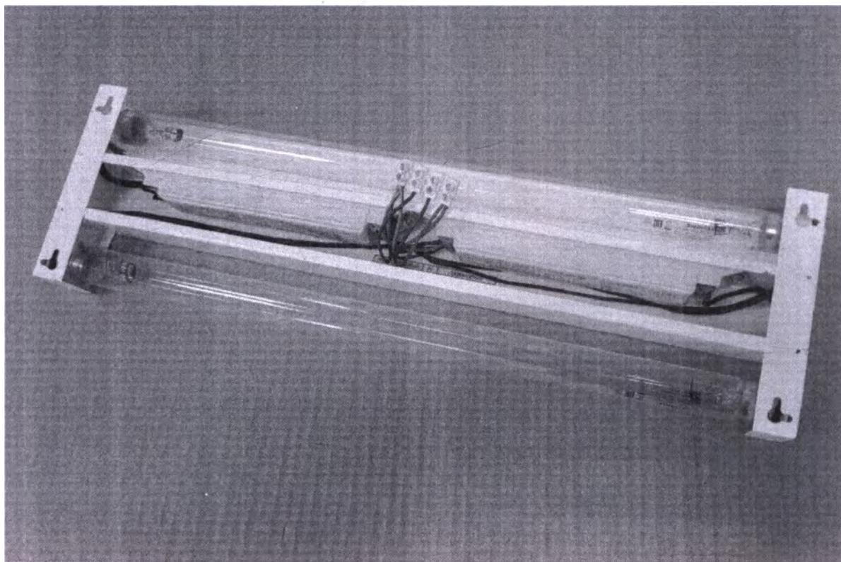
Фотография 27. Облучатель УФ-бактерицидный ОБК-70-«СПДС». Вид сзади.
