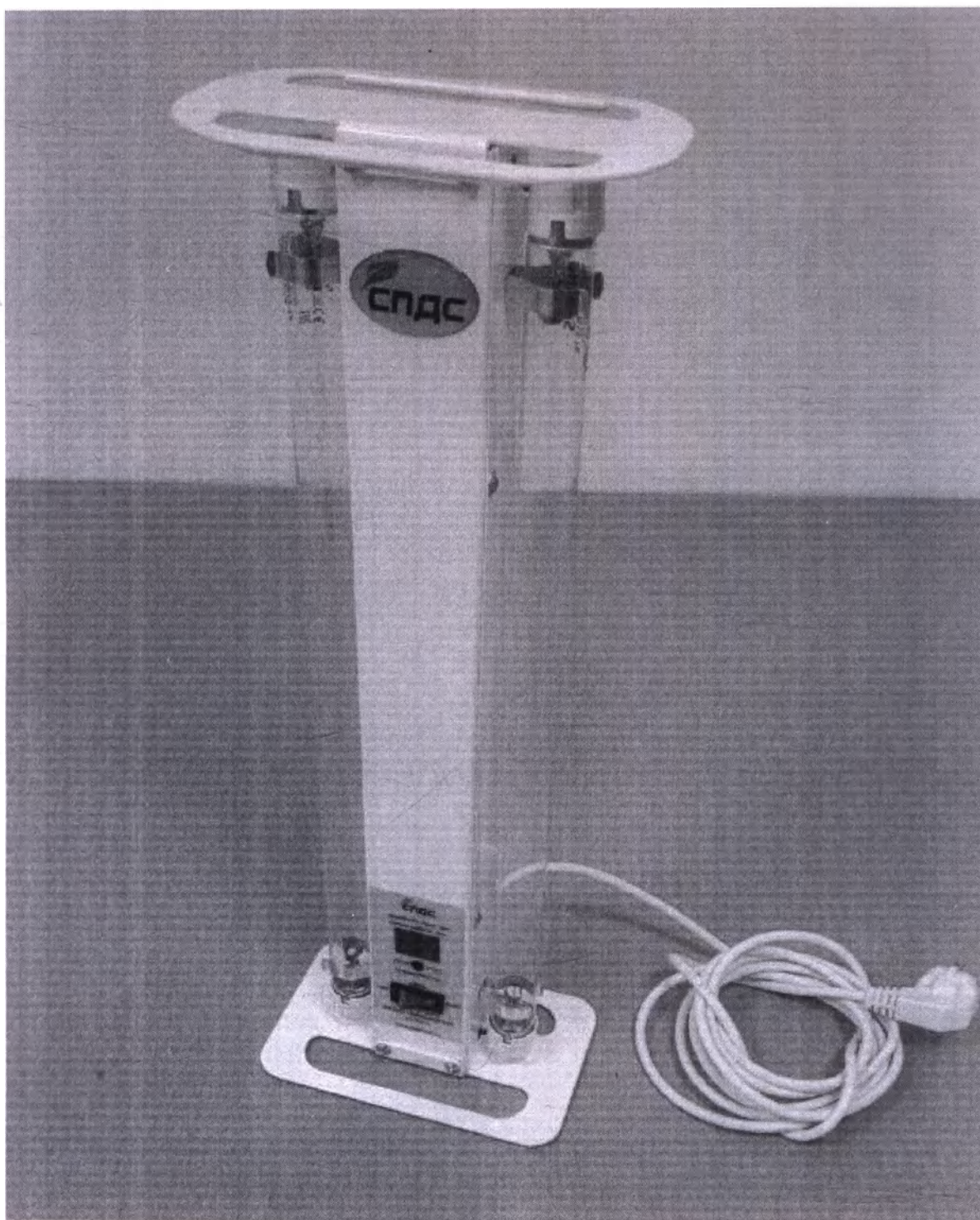
Фотография 88. Облучатель УФ-бактерицидный ОБПН-70-«СПДС». Вид спереди.
