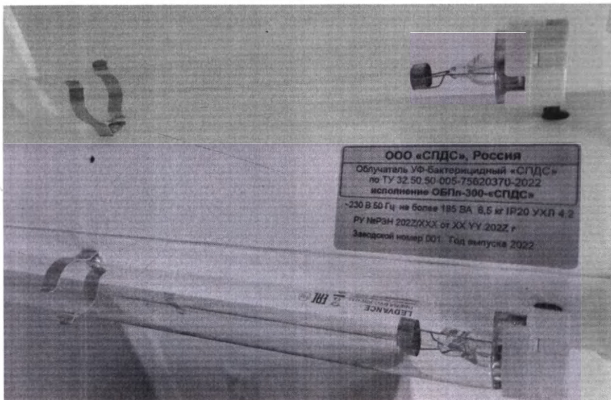
Фотография 75. Облучатель УФ-бактерицидный ОБПп-300-«СПДС». Маркировка облучателя.
