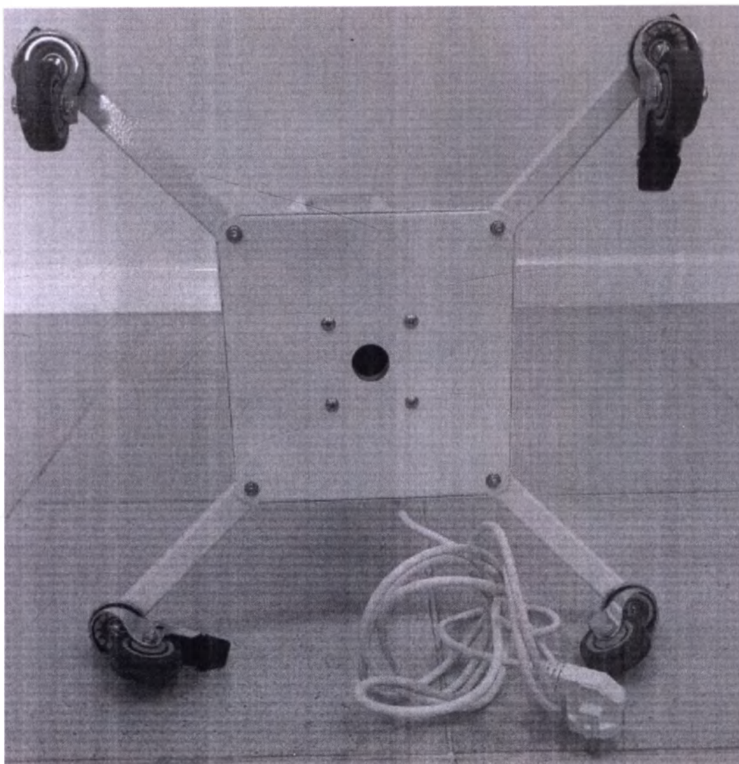
Фотография 53. Облучатель УФ-бактерицидный ОБПп-150-«СПДС». Вид снизу.
