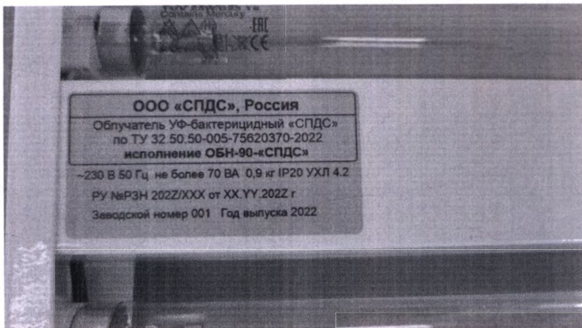
Фотография 15. Облучатель УФ-бактерицидный ОБН-90-«СПДС». Маркировка облучателя
