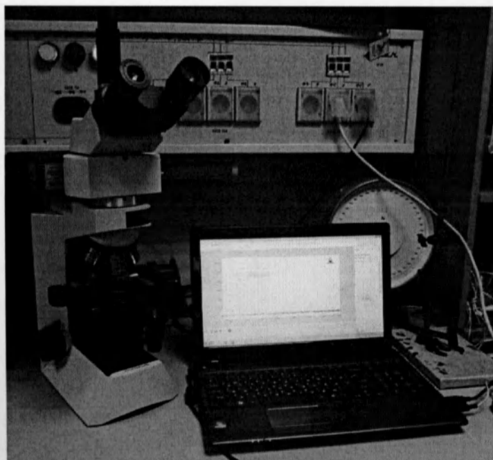
Спектрометр ИнСпектр М-532 в комплекте с микроскопом и ПК
